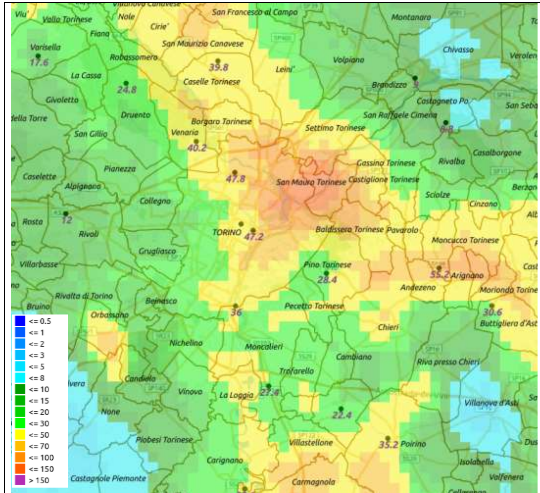
Figura 14 Mappa di precipitazione cumulata su 24 ore da radar, con dati pluviometrici in sovrapposizione per la giornata del 09 giugno 2020. Dettaglio su Torino e comuni limitrofi.
