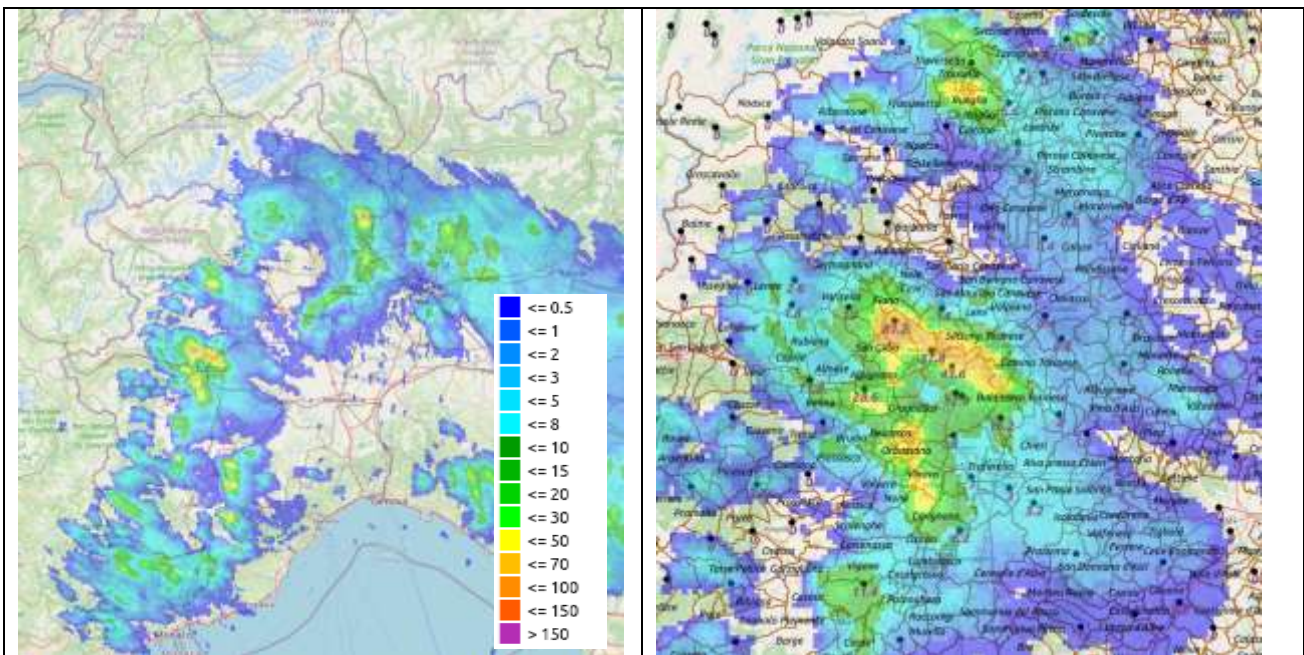
Figura 16 Mappa di precipitazione cumulata su 24 ore da radar, con dati pluviometrici in sovrapposizione e mappa di probabilità di grandine su Chieri (TO) a sinistra. Giornata del 15 giugno 2020
