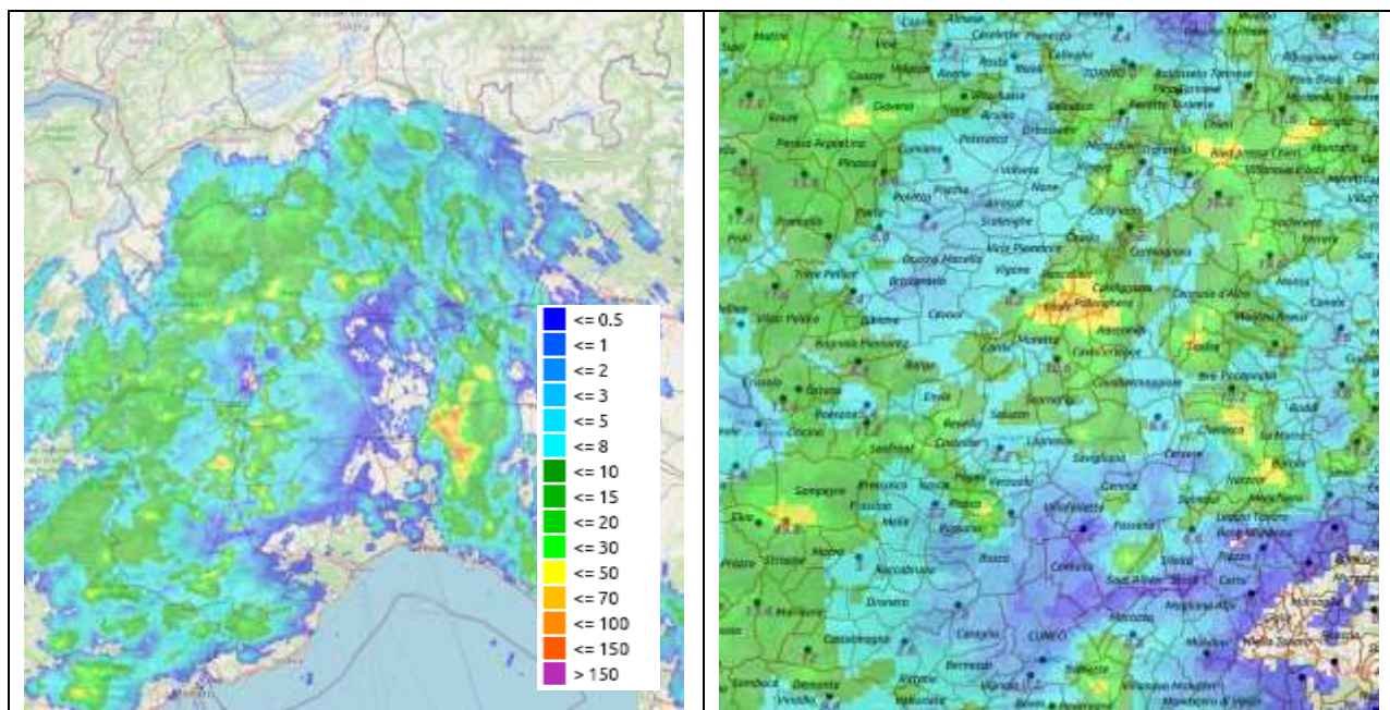
Figura 19 Mappa di precipitazione cumulata su 24 ore da radar, con dati pluviometrici in sovrapposizione e dettaglio su Polonghera (CN). Giornata del 16 giugno 2020
