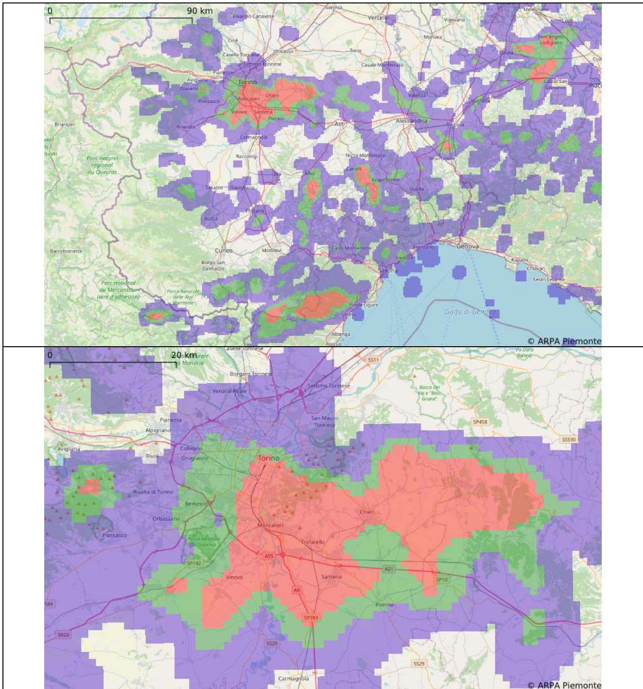
Figura 20 Mappa di probabilità di grandine sul basso Piemonte (alto) e dettaglio su Torino-Moncalieri (basso)
