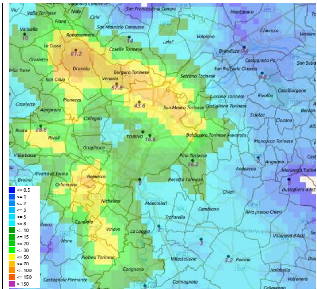
Figura 17 Mappa di precipitazione cumulata su 24 ore da radar, con dati pluviometrici in sovrapposizione per la giornata del 15 giugno 2020. Dettaglio su Torino e comuni limitrofi.
