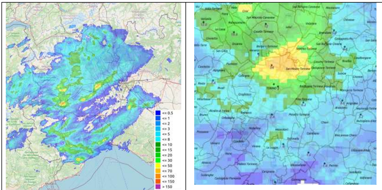
Figura 24 Giornata del 18 giugno 2020. Mappa di precipitazione cumulata su 24 ore da radar, con dati pluviometrici in sovrapposizione; dettaglio su Torino e comuni limitrofi a destra.
