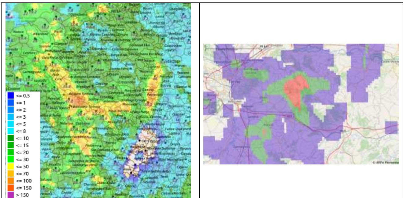
Figura 13 Mappa di precipitazione cumulata su 24 ore da radar, con dati pluviometrici in sovrapposizione e mappa di probabilità di grandine su Chieri (TO) a sinistra. Giornata del 09 giugno 2020.
