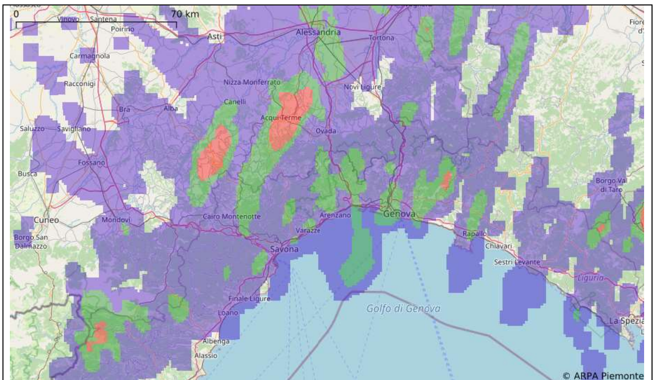
Figura 6 Mappa di probabilità di grandine per la giornata del 14 maggio 2020, sull'Alessandrino
