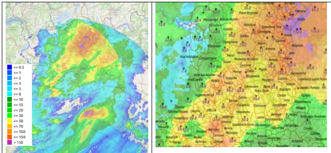
Figura 11 Pioggia cumulata stimata da radar per il 7 giugno 2020 e particolare su biellese, con dati pluviometrici della rete meteorologica.
