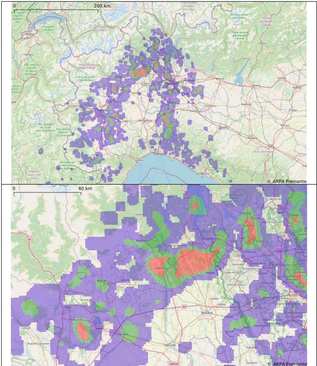
Figura 18 Mappa di probabilità di grandine sul Piemonte (alto) e dettaglio su Biella-Novara (basso) nella giornata del 16 giugno 2020.
