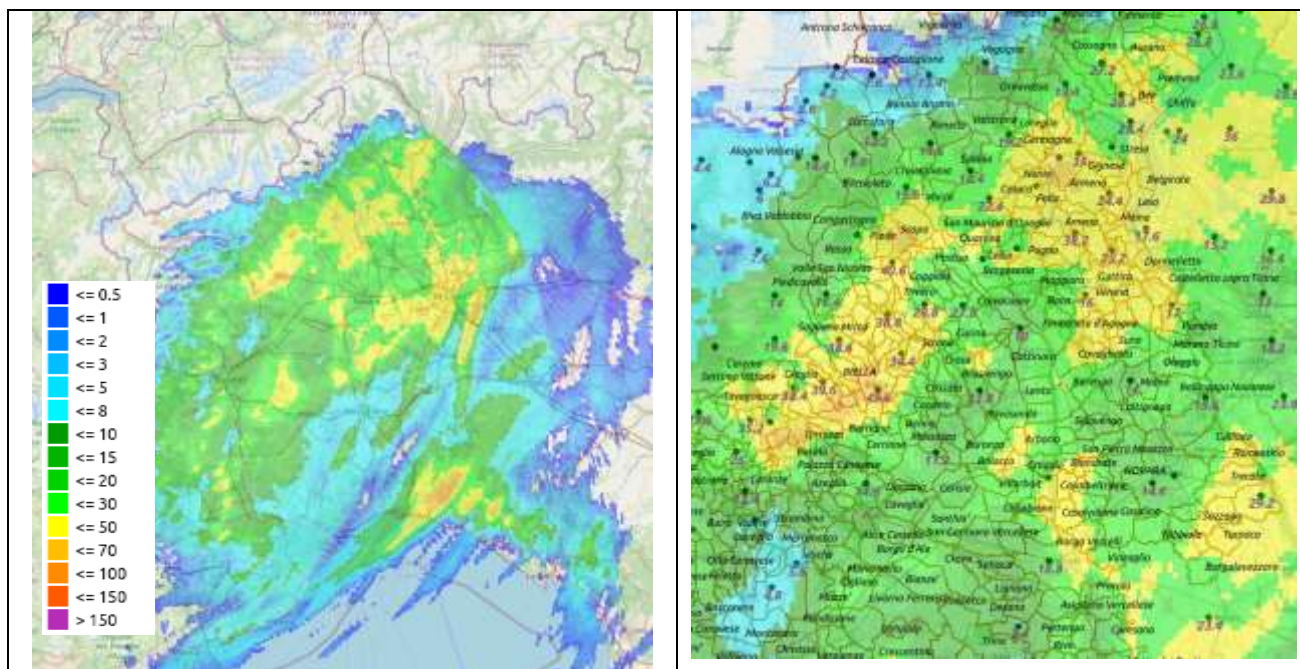
Figura 7 Mappe di precipitazione cumulata stimata da radar sulle 24 ore del 15 maggio 2020. Nei pannelli in basso particolare su Biellese, Verbanese e Novarese, con annesse misure pluviometriche.
