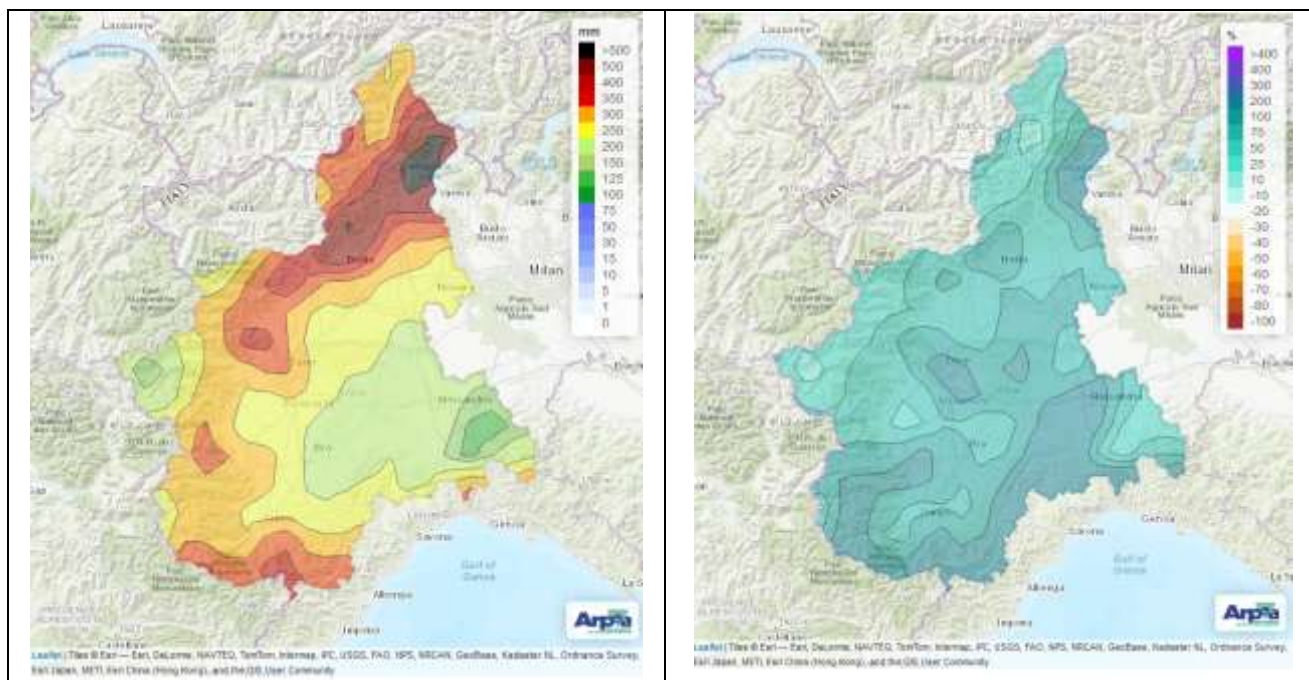
Figura 2 Precipitazione cumulata tra il 9 maggio ed il 18 giugno 2020, per complessivi 40 giorni (a sinistra) e anomalia di precipitazione cumulata rispetto al medesimo periodo 1981 – 2010 (a destra).
