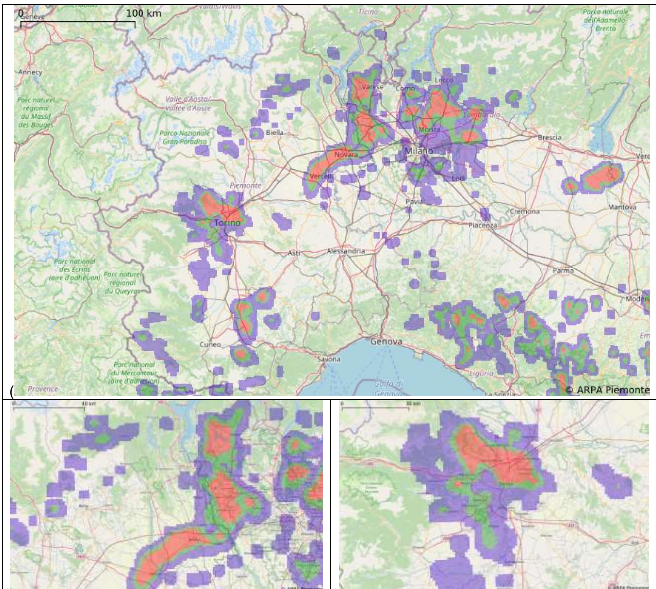
Figura 15 Mappa di probabilità di grandine sul Piemonte (alto) e dettaglio su Novara (basso sx) e Torino (basso dx)
