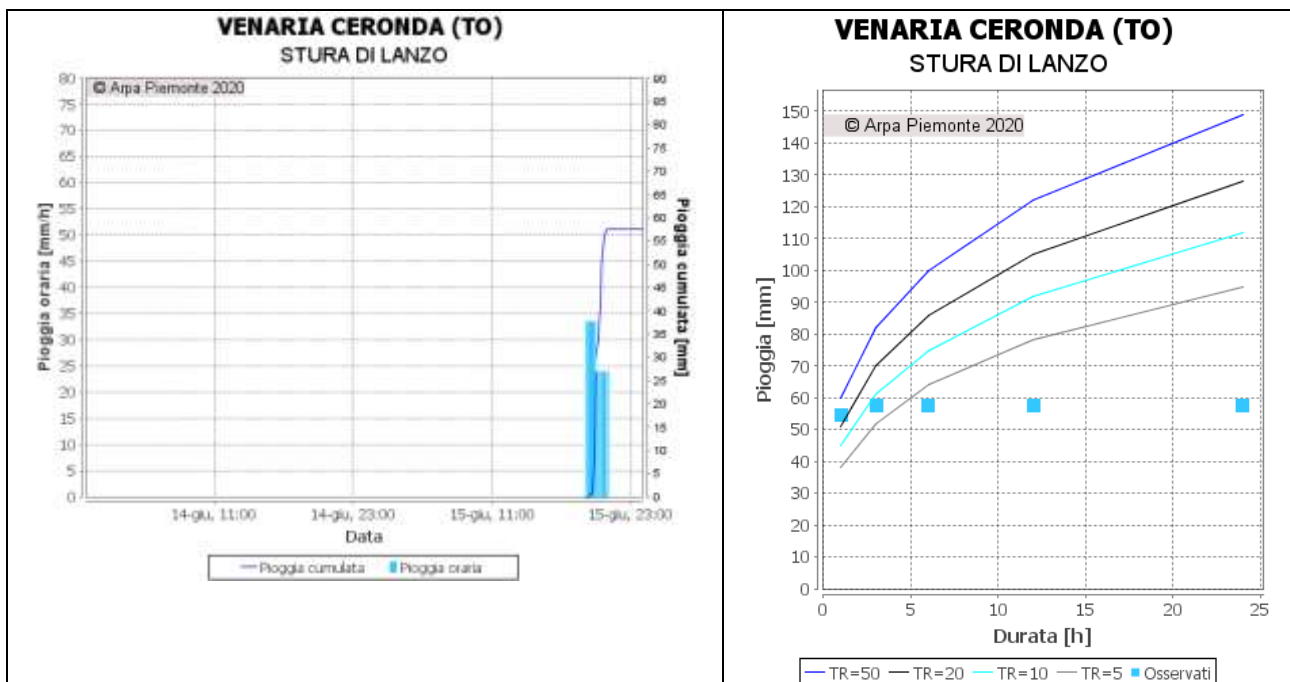
Figura 23 Ietogrammi delle stazioni che hanno registrato le precipitazioni maggiori e linee segnalatrici di possibilità pluviometrica per la determinazione del tempo di ritorno del fenomeno
