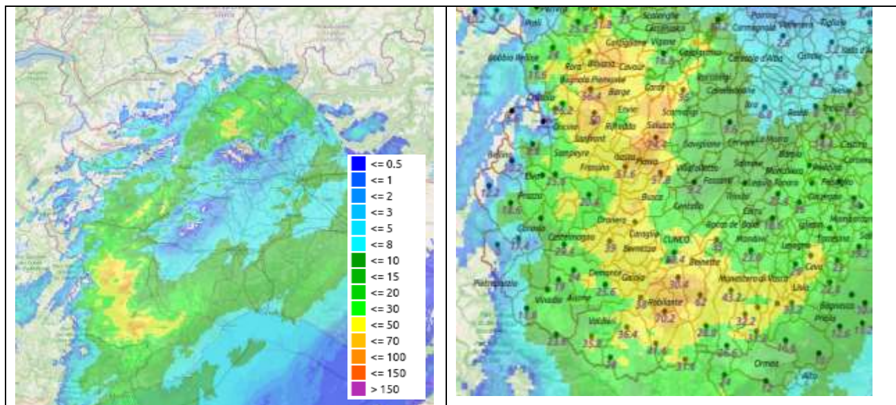
Figura 8 Pioggia cumulata stimata da radar per il 16 maggio 2020 e particolare su Cuneese sud-occidentale, con dati pluviometrici.
