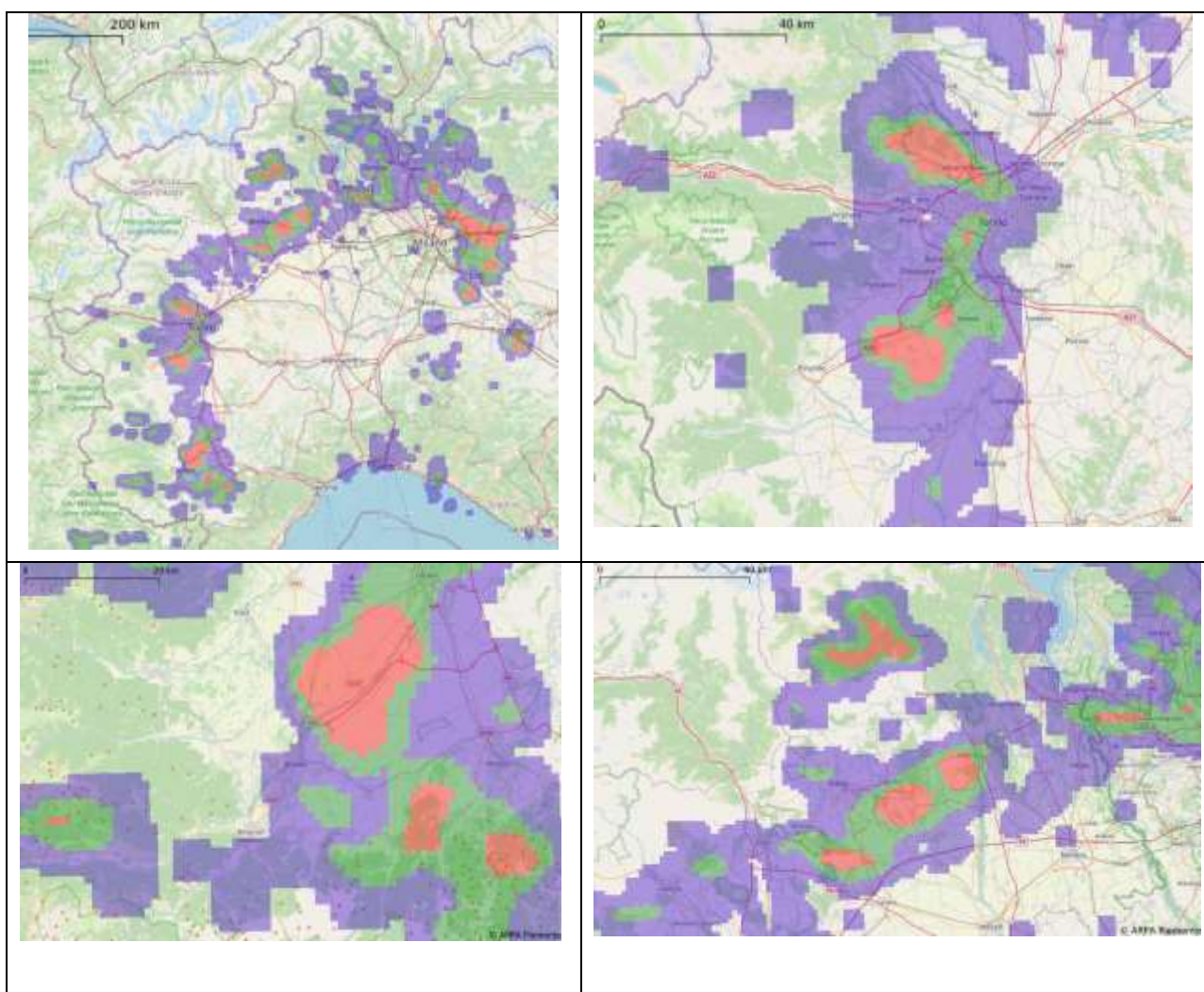
Figura 9 Mappa di probabilità di grandine sul Piemonte (alto a sinistra) e dettaglio su torinese (alto destra), cuneese (basso sinistra) e biellese (basso destra).
