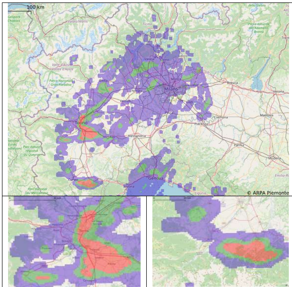
Figura 10 Mappa di probabilità di grandine sul Piemonte (alto) e dettaglio su Torino, in basso a sinistra e Mondovì (CN) in basso a destra.
