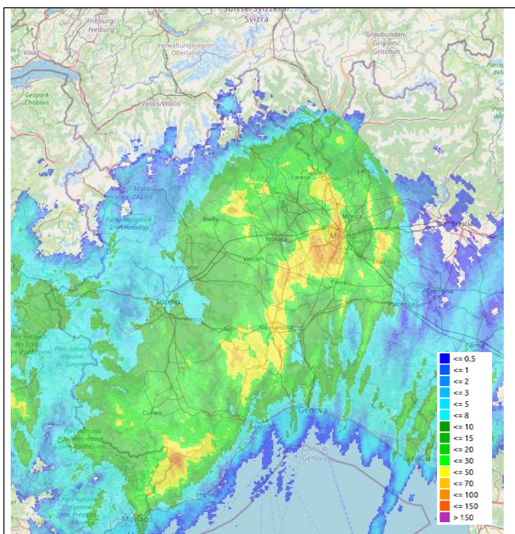
Figura 5 Precipitazione cumulata su 24 ore del 14 maggio 2020 stimata da radar
