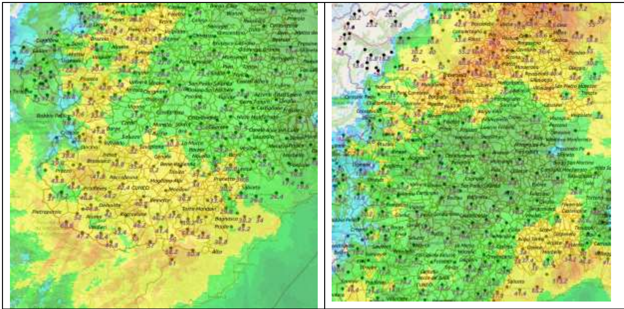
Figura 4 Precipitazione cumulata su 24 ore; a sinistra 10 maggio 2020, a destra: 11 maggio 2020.
