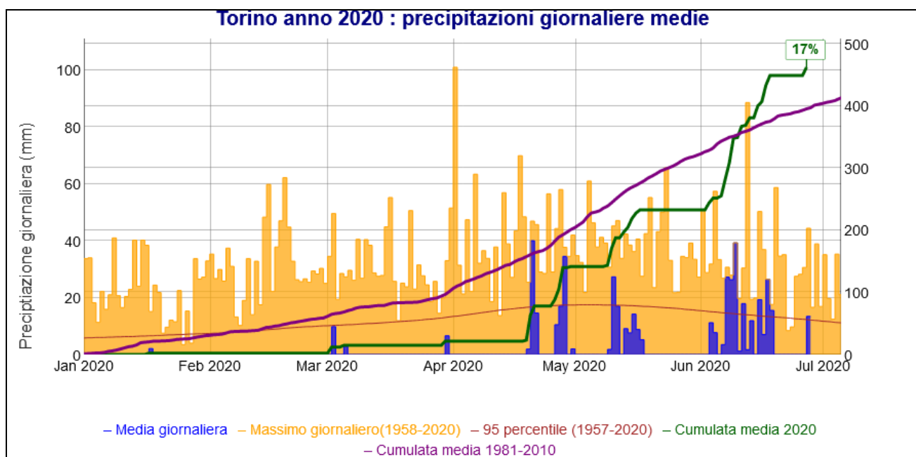
Figura 1 Andamento delle precipitazioni nel 2020 su Torino.
