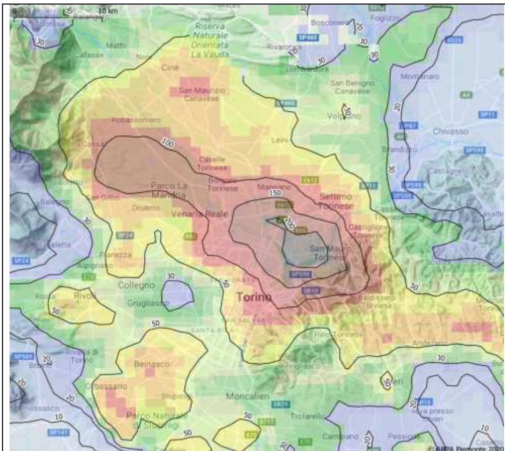
Figura 25 Mappa di precipitazione cumulata sulle tre giornate del 9, 15, e 18 giugno 2020 da sistemi radarmeteorologici, con dati pluviometrici su Torino e comuni limitrofi.
