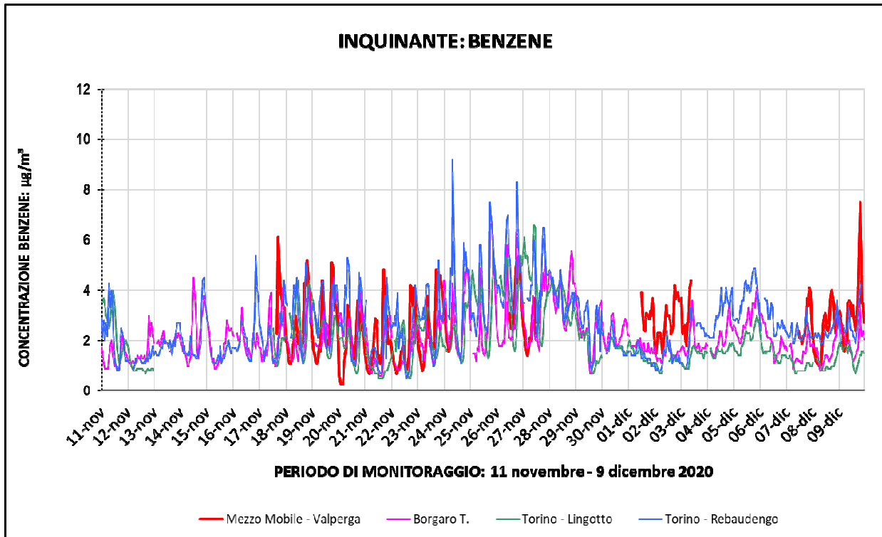
Figura 4: andamento Benzene a Valperga – prima campagna di monitoraggio
