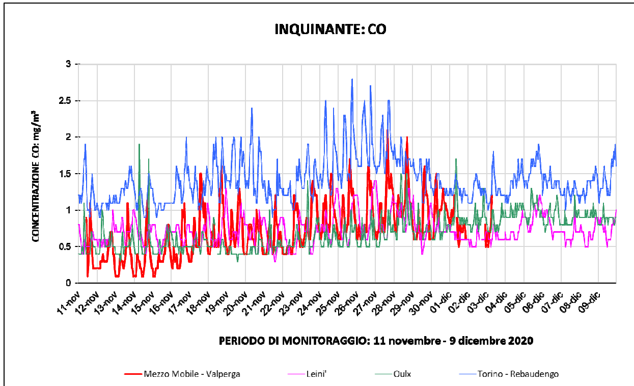
Figura 10: andamento CO a Valperga – prima campagna di misura
