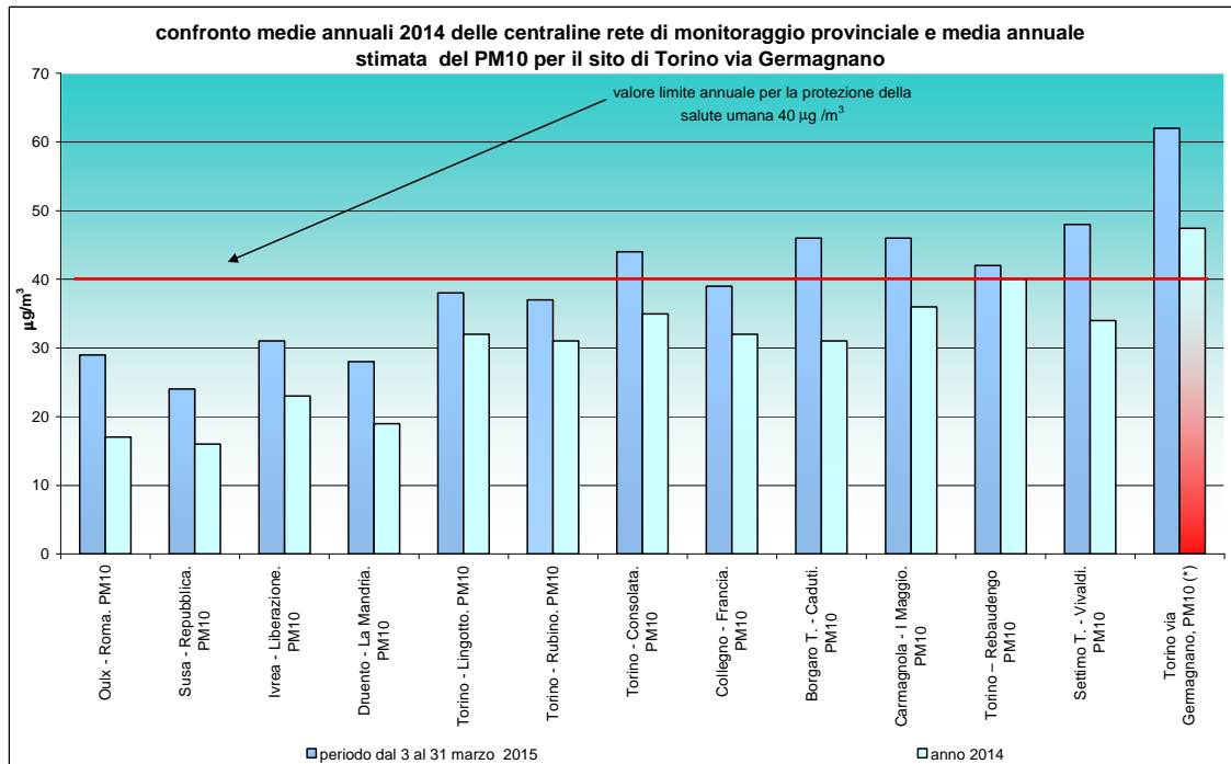
Figura 3: confronto medie annuali 2014 e concentrazioni medie rilevate nel periodo di campionamento
