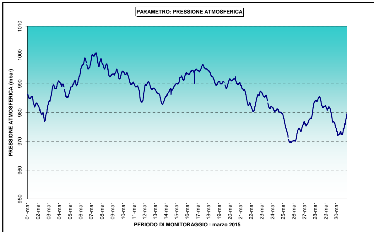
Figura 10: Pressione Atmosferica
