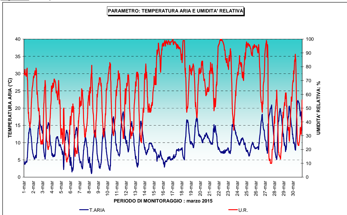
Figura 9: Temperatura Aria e Umidità Relativa
