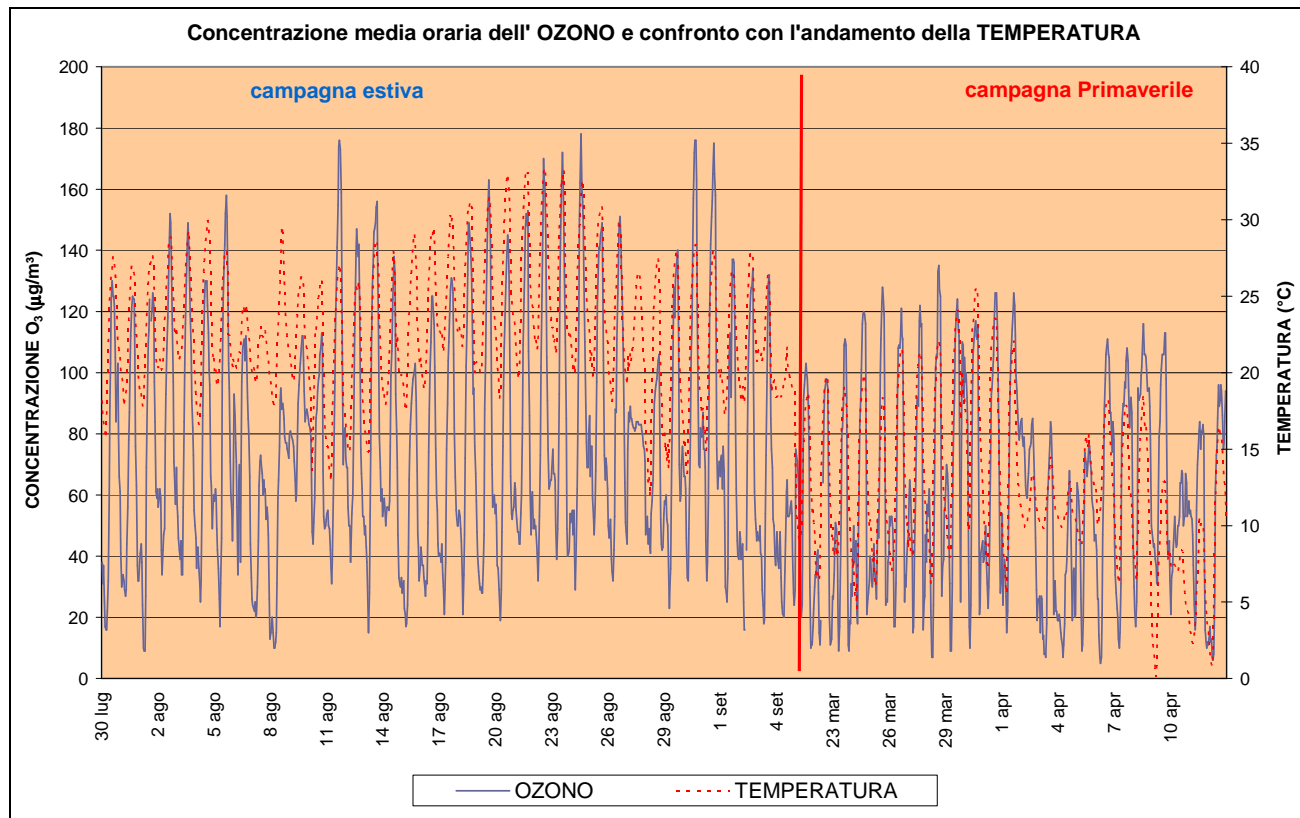
Figura 32 – Andamento orario dell'Ozono rispetto alla temperatura dell'aria, nel corso delle due campagne di monitoraggio
