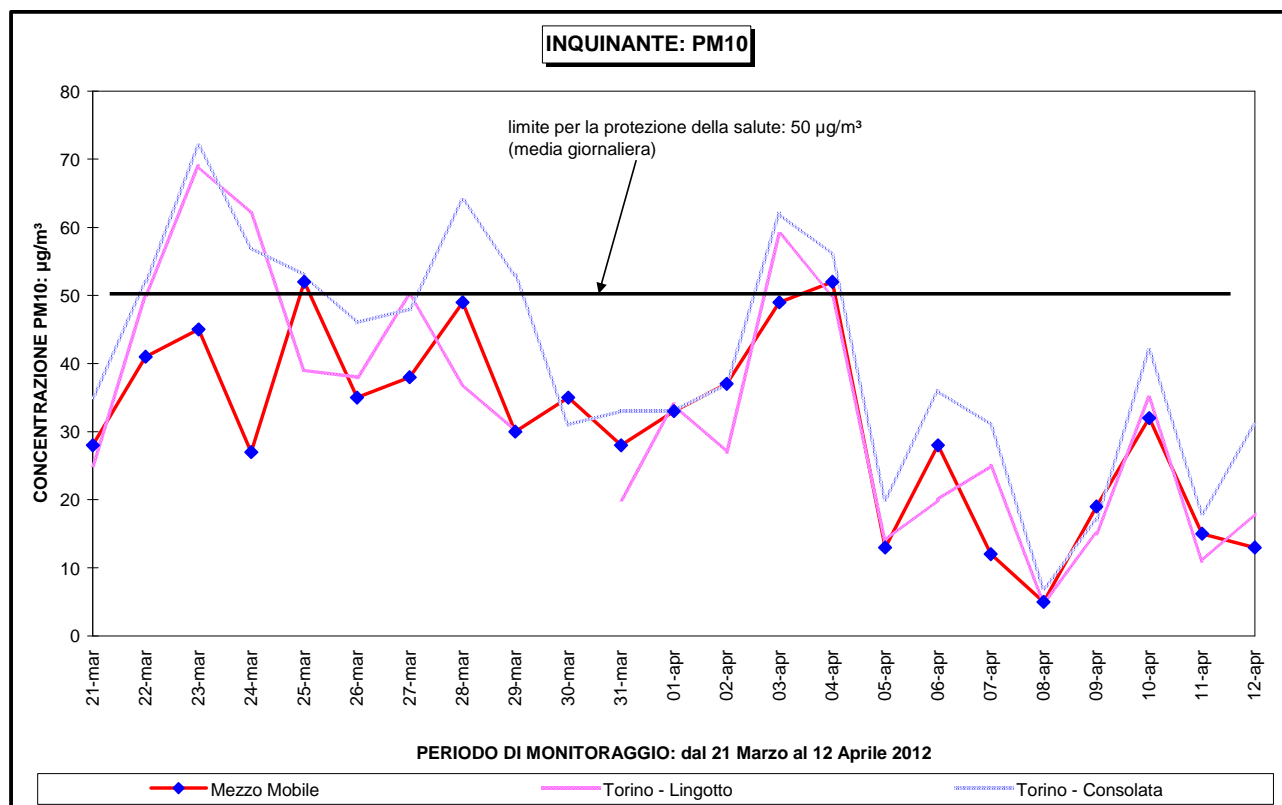
Figura 25 – Particolato sospeso PM 10 : confronto con il limite giornaliero per la protezione della salute
