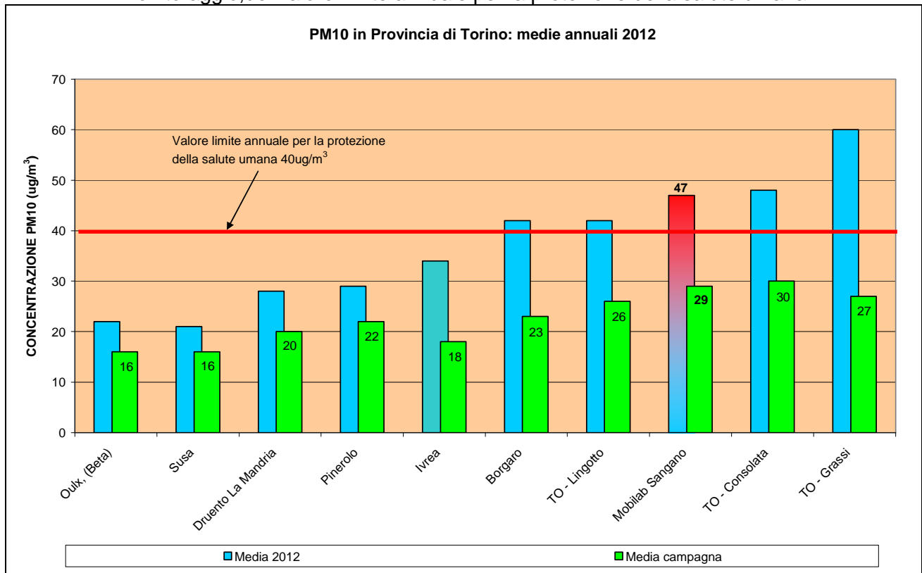
Figura 27 – Particolato sospeso PM 10 : confronto medie annuali e medie nel periodo di monitoraggio, del valore limite annuale per la protezione della salute umana
