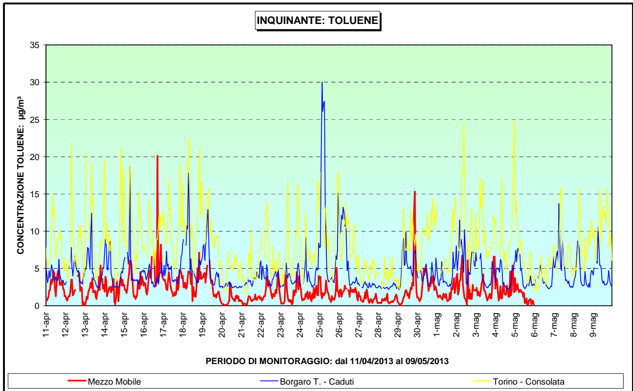
Figura 23 – Toluene: andamento della concentrazione oraria nel corso della campagna di monitoraggio
