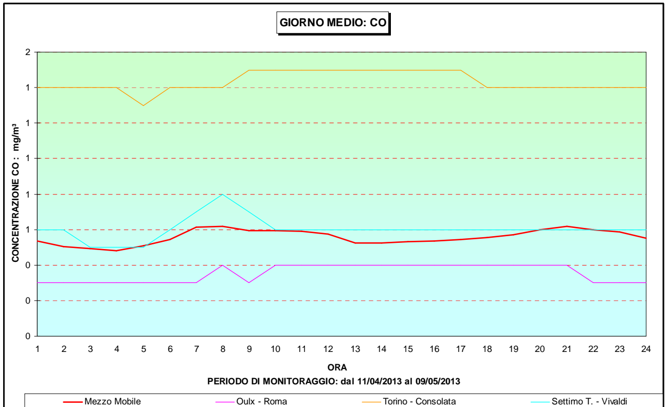
Figura 16 - CO andamento del giorno medio
