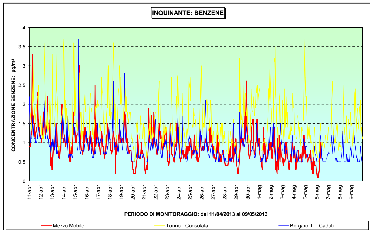
Figura 22 – Benzene: andamento della concentrazione oraria nel corso della campagna di monitoraggio
