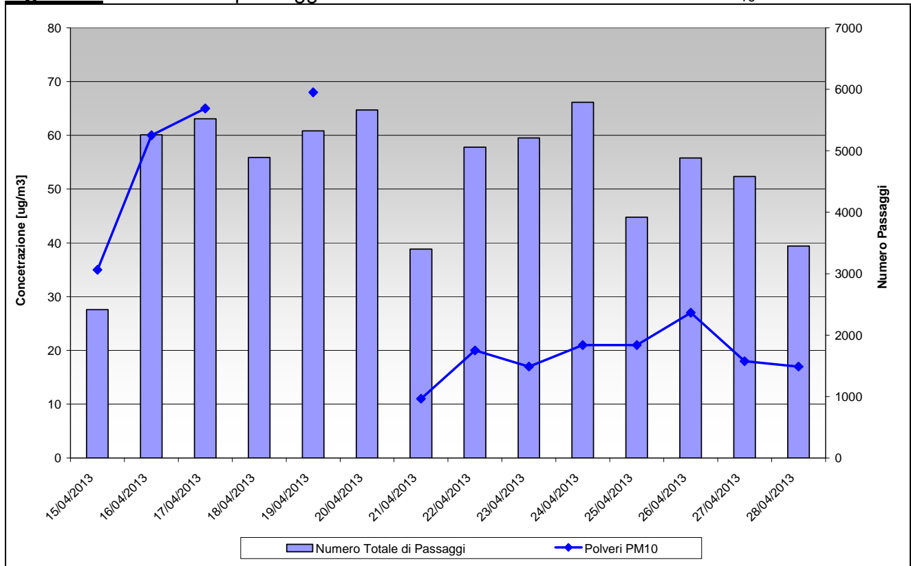
Figura 34 – Numero di passaggi di veicoli e valore di concentrazione di PM 10
