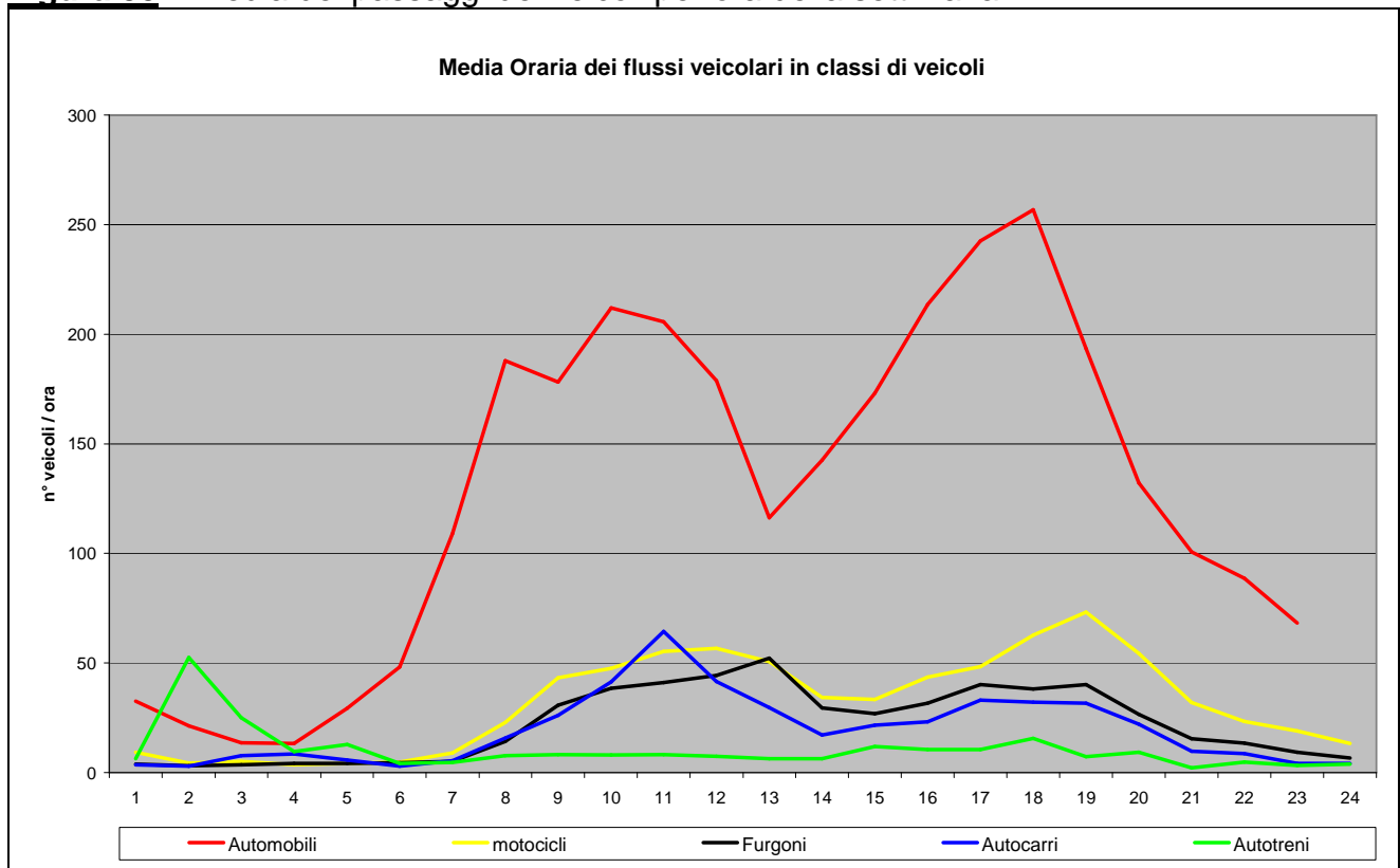
Figura 35 – Media dei passaggi dei veicoli per ora della settimana
