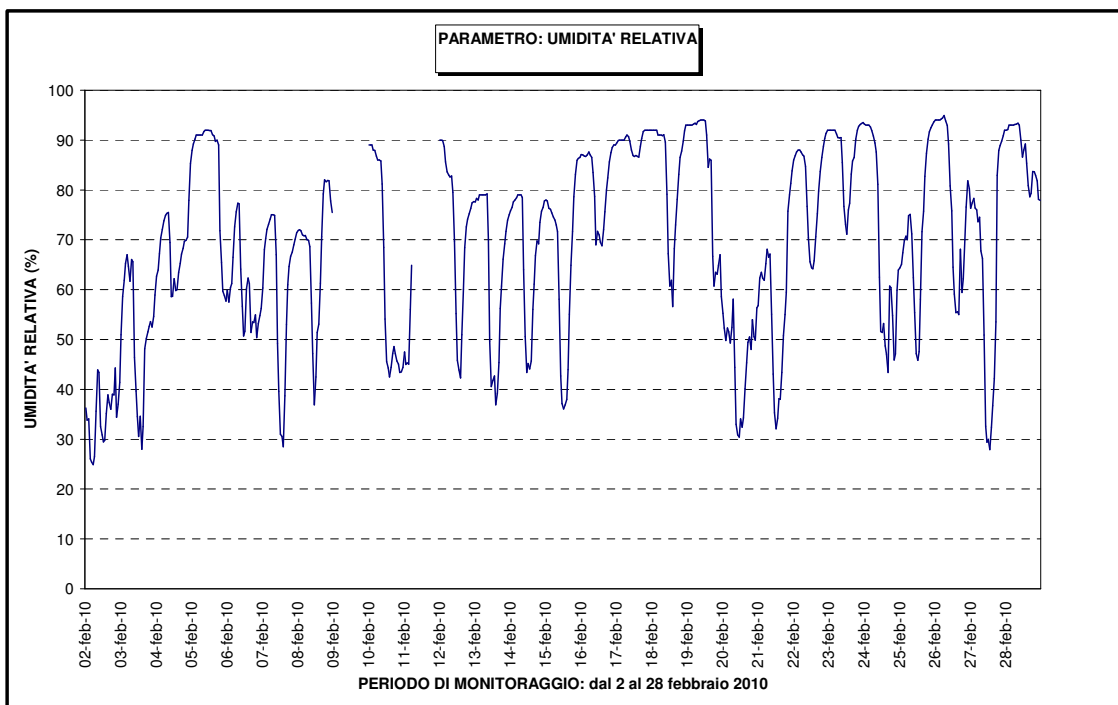
Figura 5: Umidità relativa
