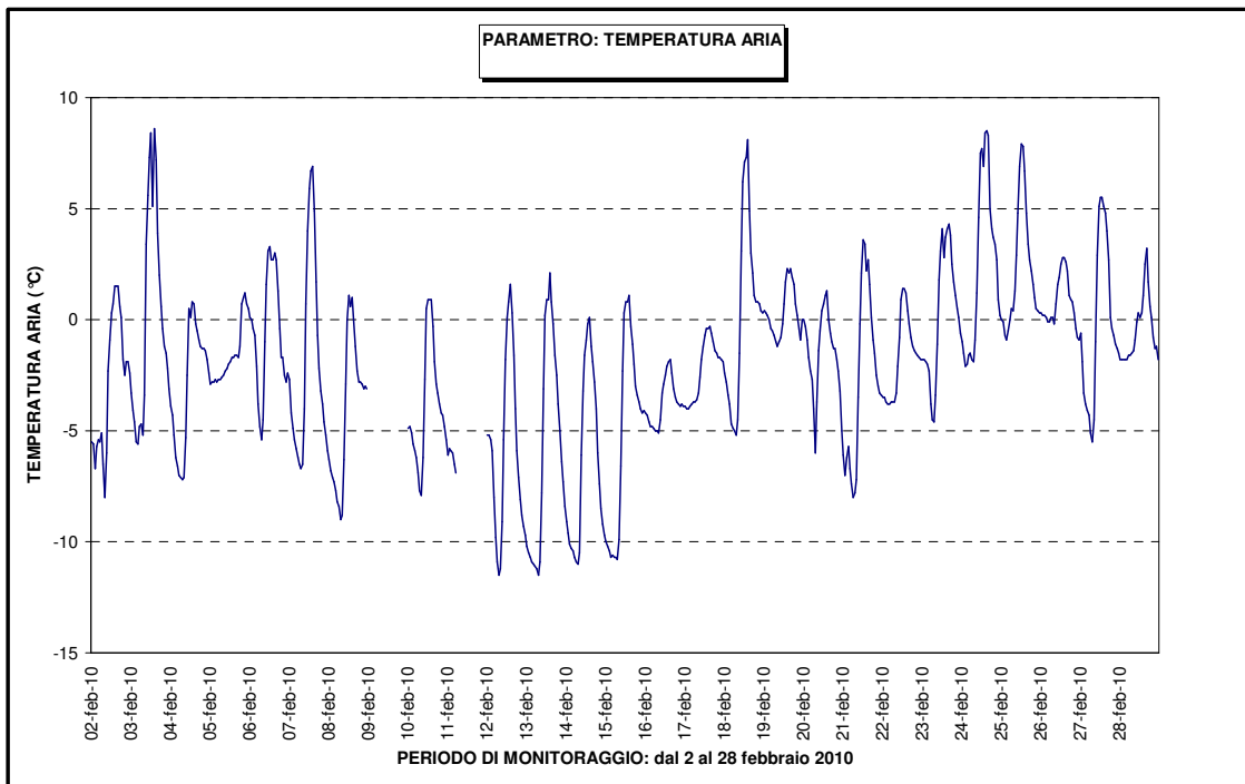
Figura 4: Temperatura Aria
