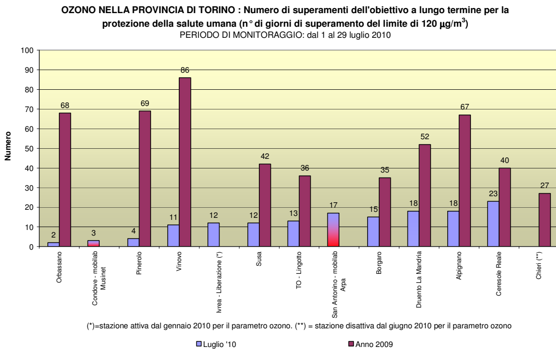
Figura 11 : O3 confronto Numero di superamenti dell'obiettivo a lungo termine per la protezione della salute umana (n° di giorni di superamento del limite di 120 µg/m3)
