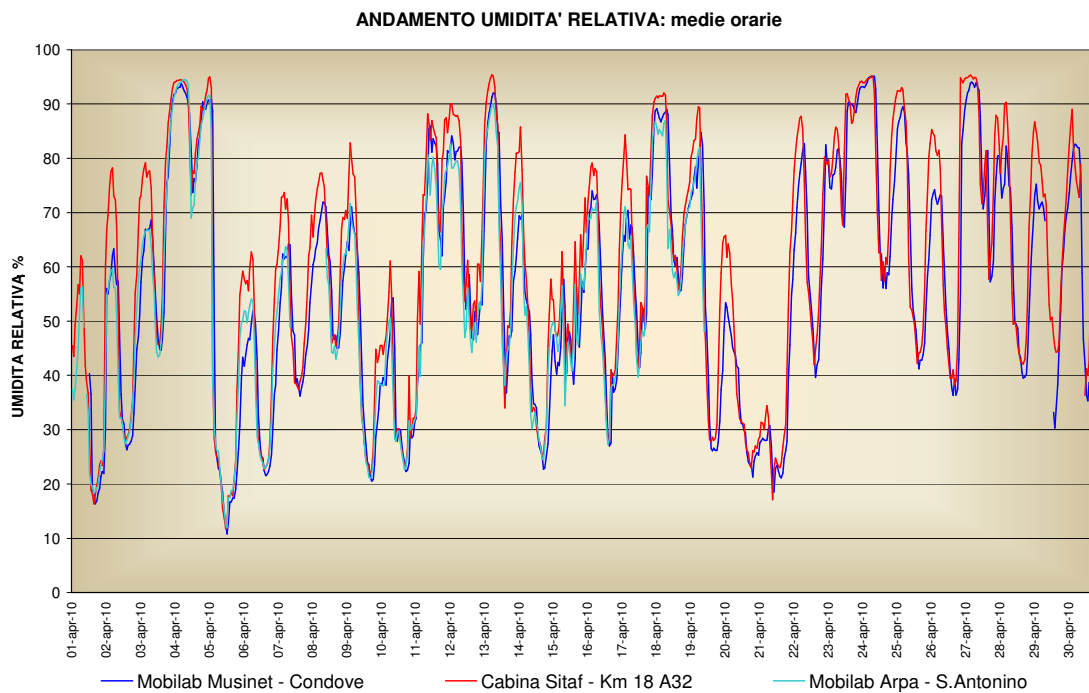
Figura 6: Umidità relativa
