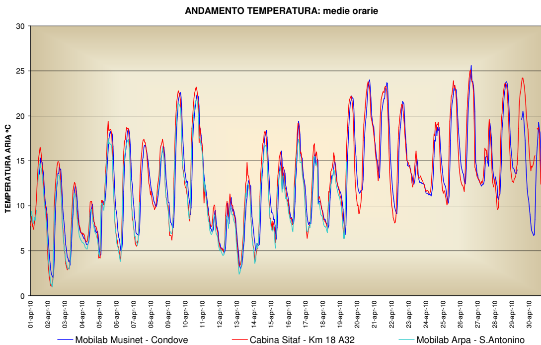
Figura 5: Temperatura Aria
