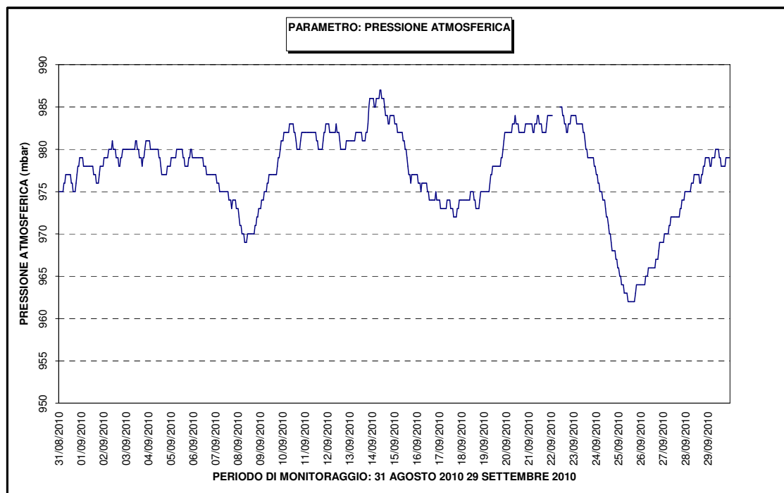
Figura 3: Pressione Atmosferica
