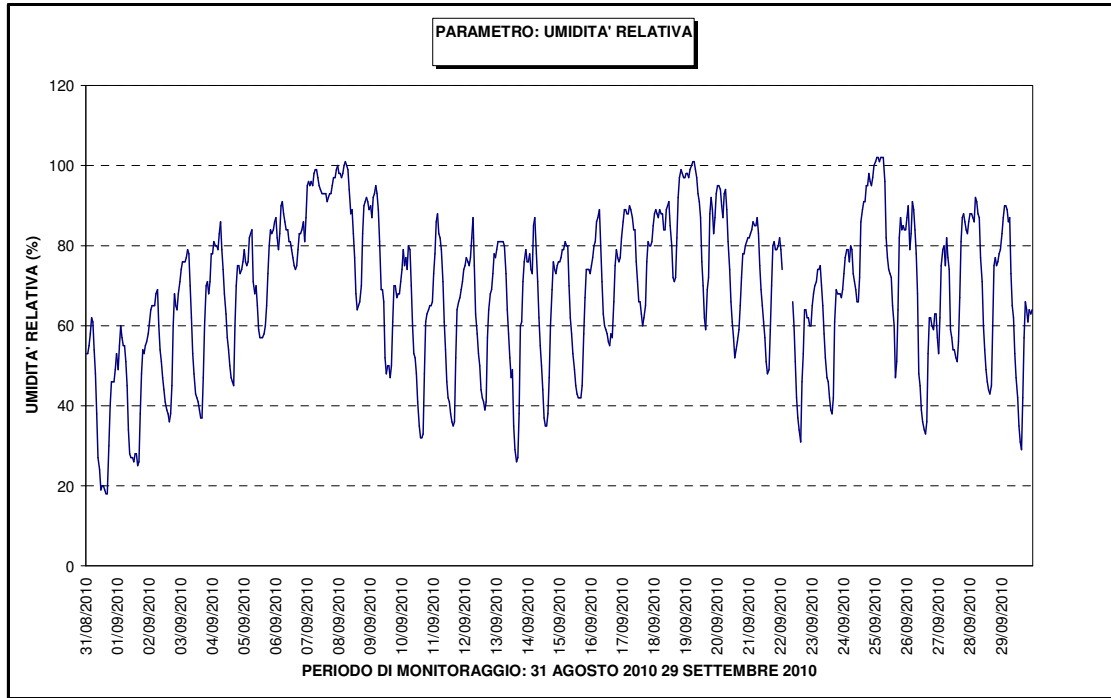
Figura 4: Umidità Relativa
