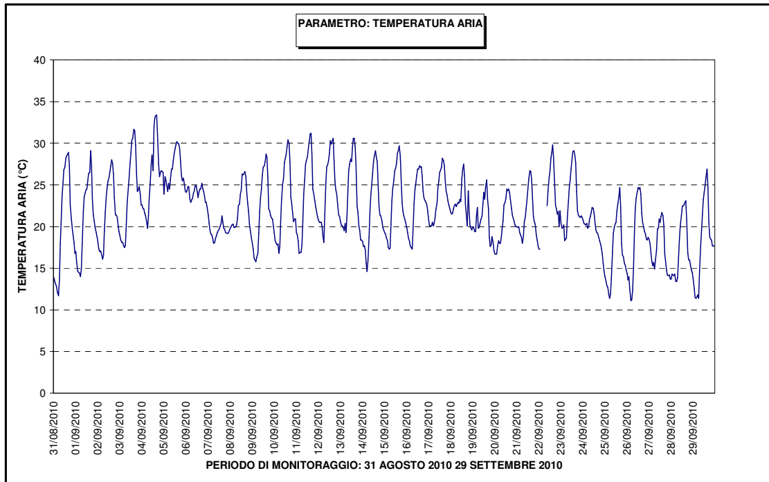
Figura 5: Temperatura aria
