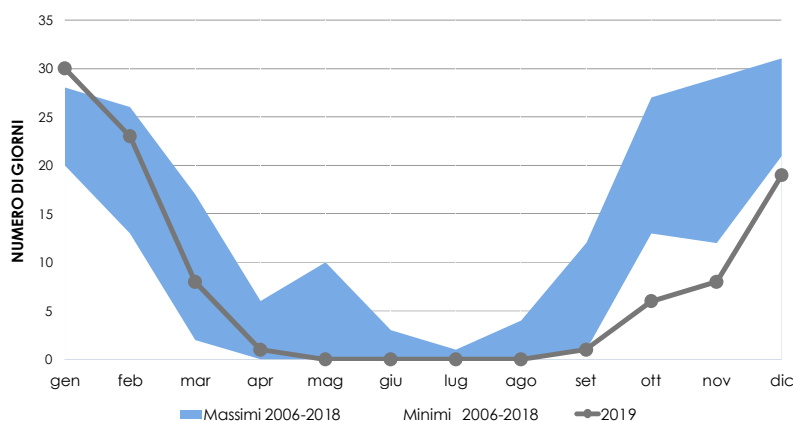
NUMERO DI GIORNI FAVOREVOLI ALL'ACCUMULO DI PM10 AGGLOMERATO TORINESE 2006-2019
