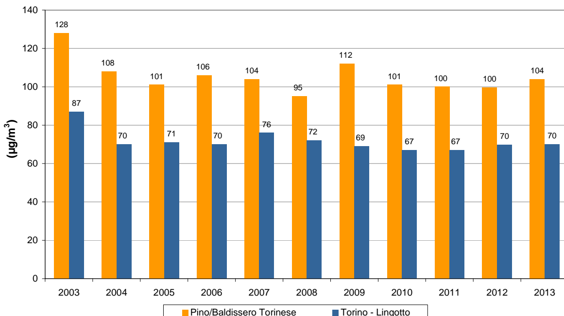
CONCENTRAZIONI MEDIE ESTIVE (maggio - settembre) di OZONO 2003 - 2013
