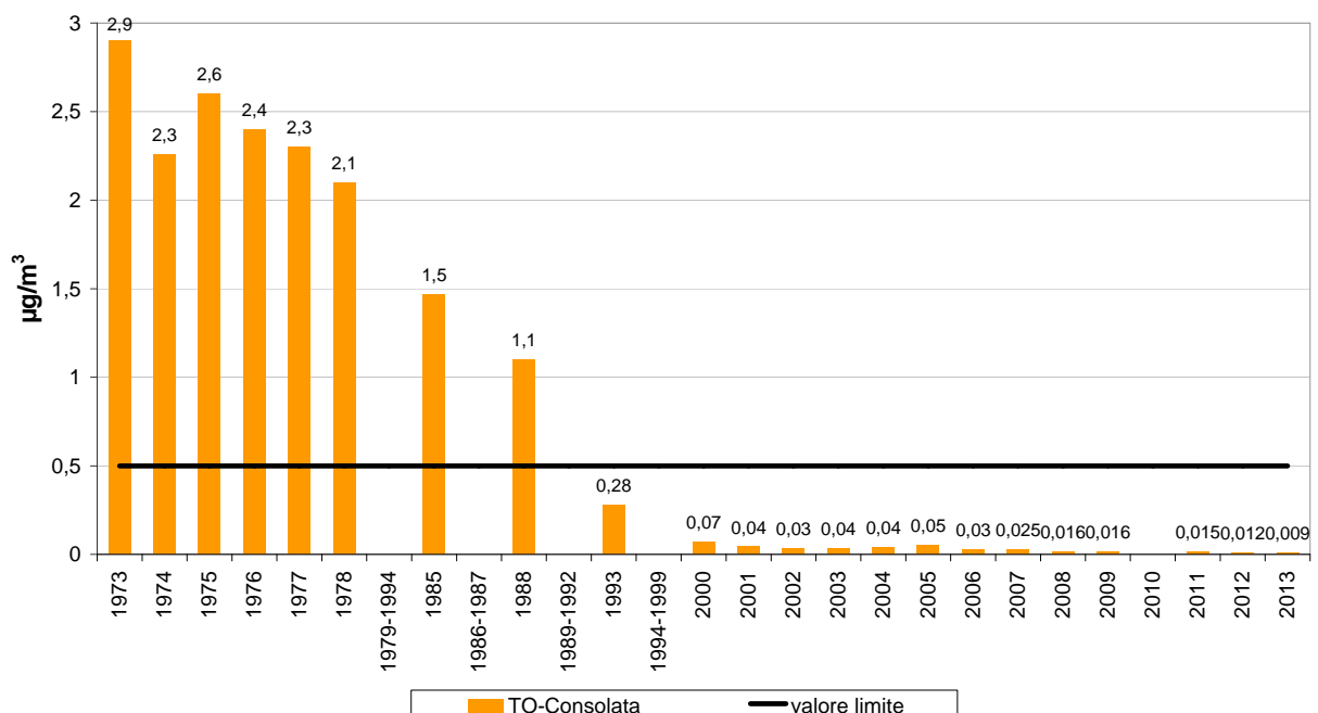
CONCENTRAZIONI MEDIE ANNUE DI PIOMBO 1973 - 2013
