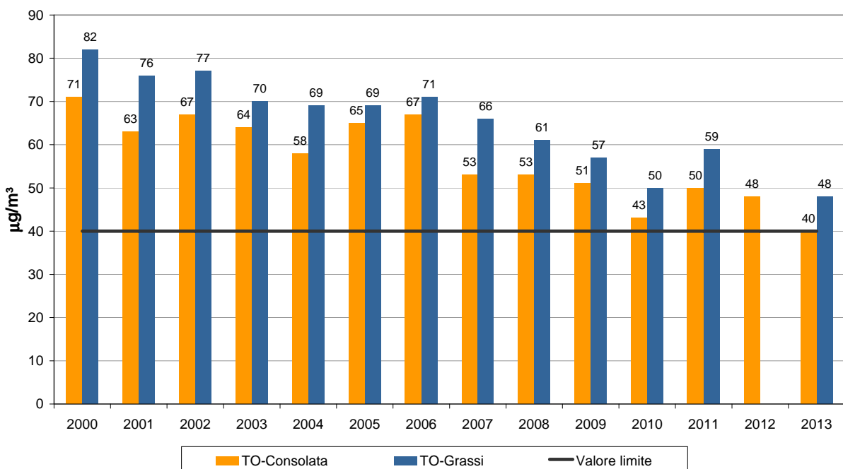
PM10 - ANDAMENTO STORICO DEL VALORE MEDIO ANNUALE 2000 - 2013
