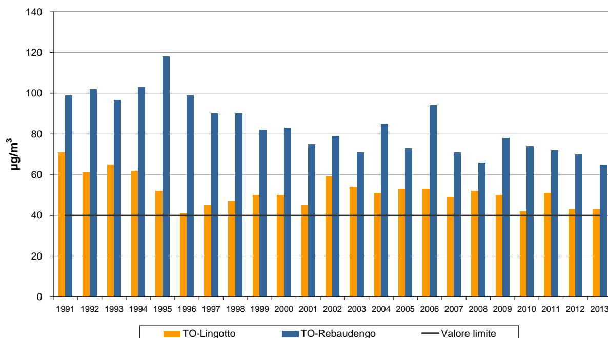
CONCENTRAZIONI MEDIE ANNUE DI \text{NO}_2 1991-2013
