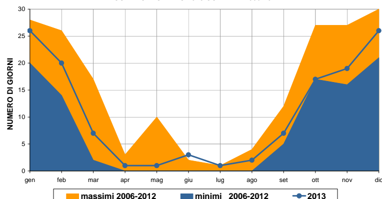
NUMERO DI GIORNI FAVOREVOLI ALL'ACCUMULO DI PM10 AGGLOMERATO TORINESE ANDAMENTO MENSILE CONFRONTO ANNO 2013 CON ANNI 2006-2012
