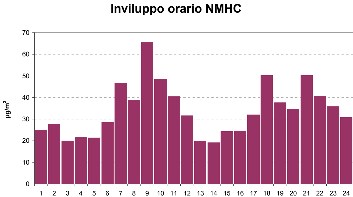
Figura 14: inviluppo orario NMHC
