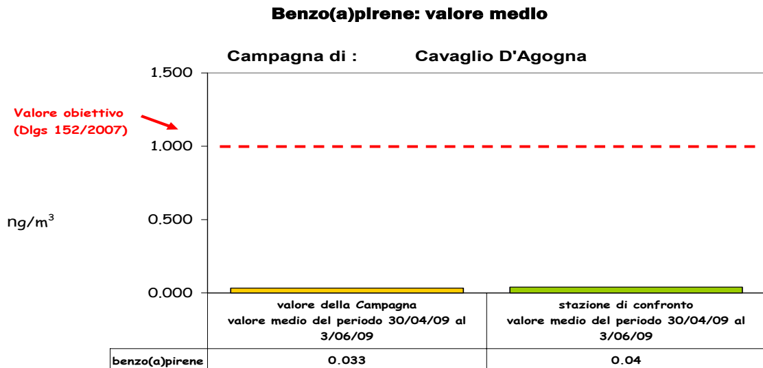
Figura 26: confronto tra il sito di monitoraggio e la stazione fissa di Novara dei valori medi nel periodo
