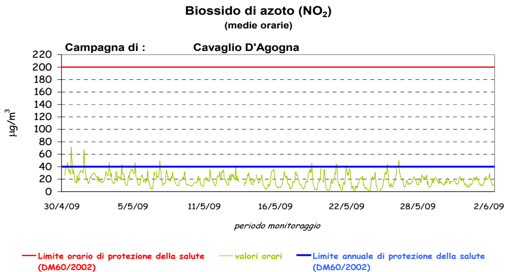
Figura 7: medie orarie Biossido di Azoto.
