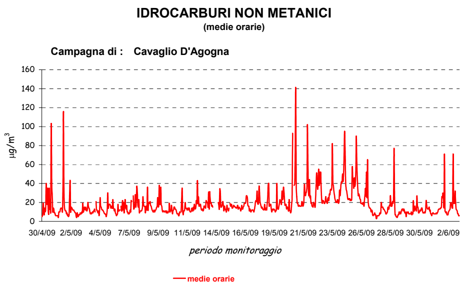
Figura 13: medie orarie idrocarburi non metanici (NMHC)
