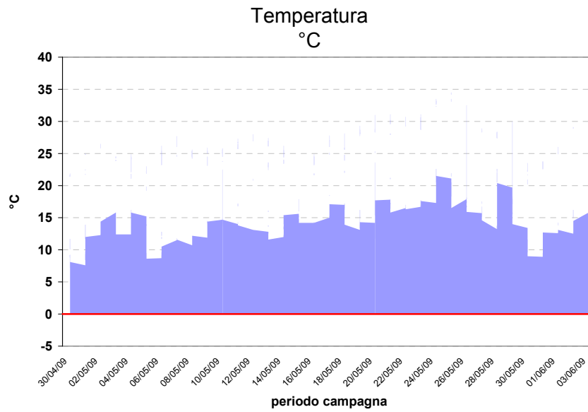
Figura 31: Temperatura media
