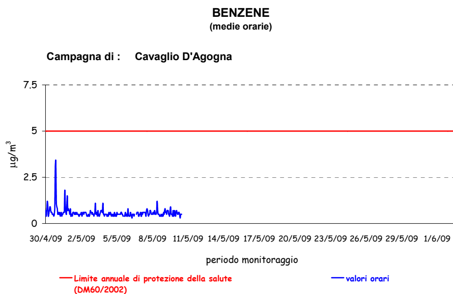
Figura 16: Benzene – valori orari
