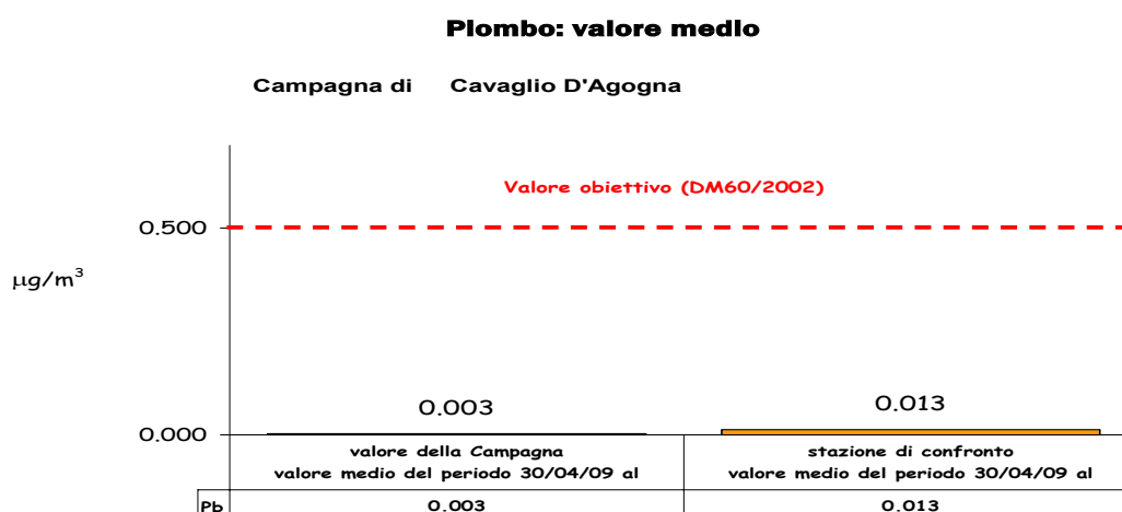
Figura 24: confronto tra il sito di monitoraggio e la stazione fissa di Novara dei valori medi nel periodo
