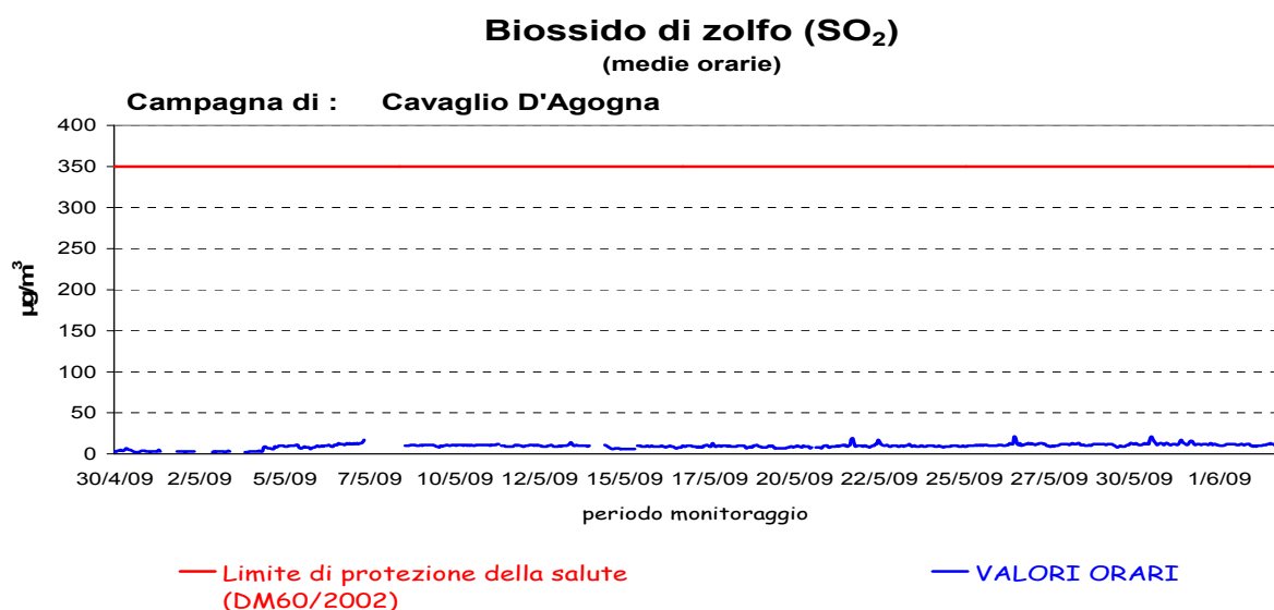
Figura 2: medie orarie Biossido di Zolfo
