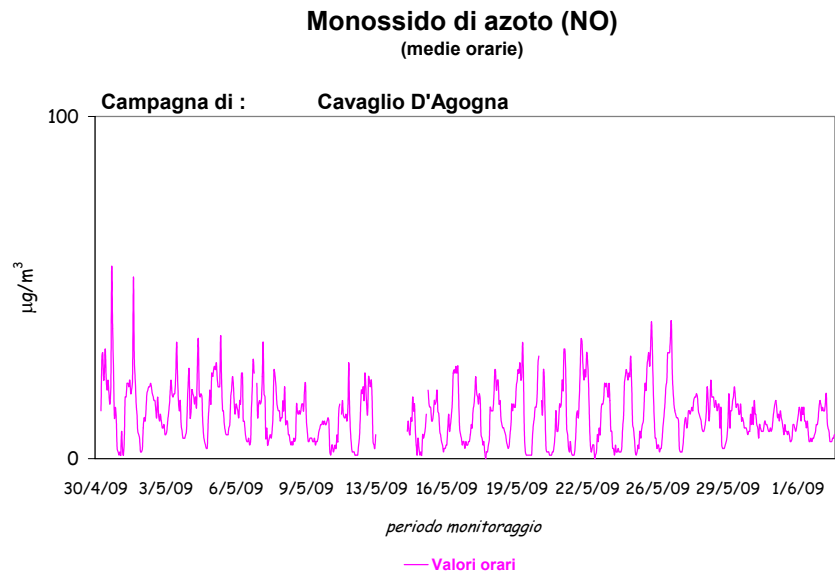
Figura 12: medie orarie Monossido di Azoto.
