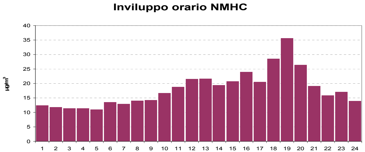
Figura 14: inviluppo orario NMHC
