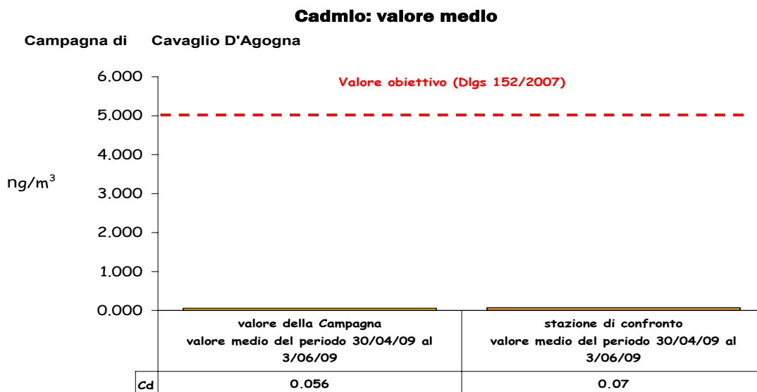
Figura 20: confronto tra il sito di monitoraggio e la stazione fissa di Novara dei valori medi nel periodo
