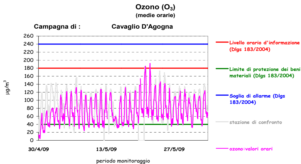
Figura 9: medie orarie ozono
