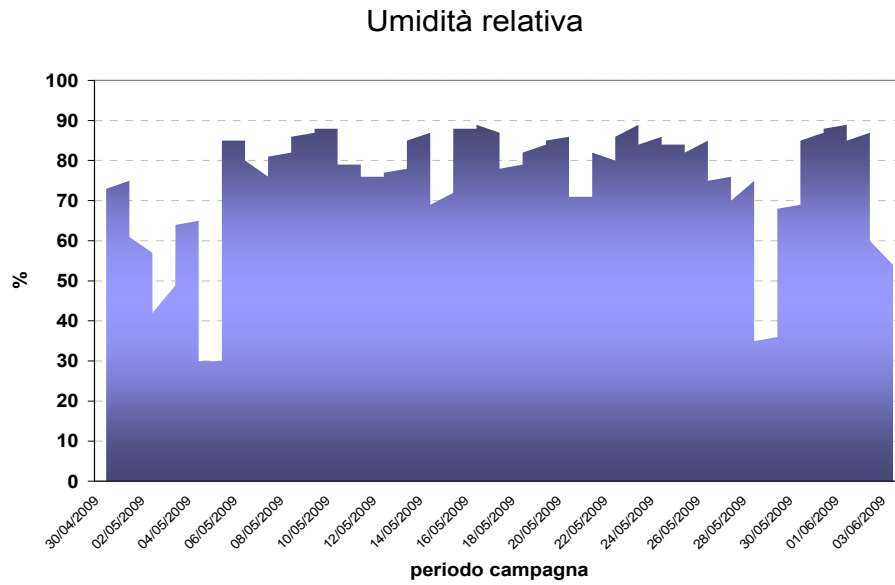
Figura 28: valori giornalieri di umidità relativa
