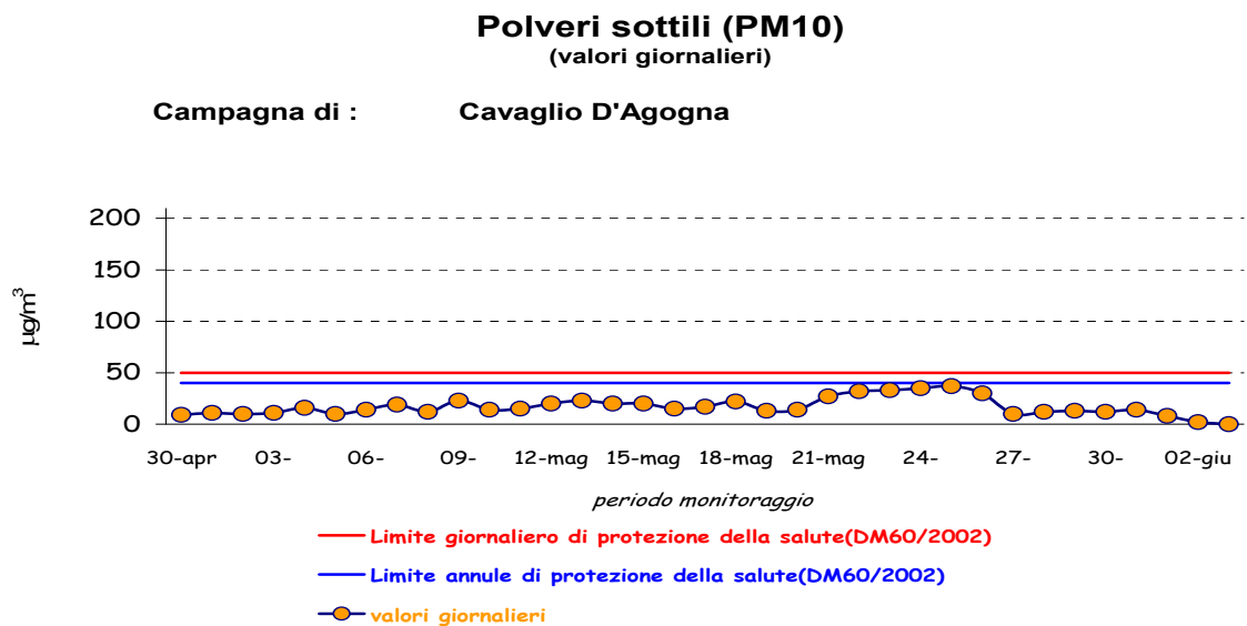
Figura 17: valori giornalieri di PM10
