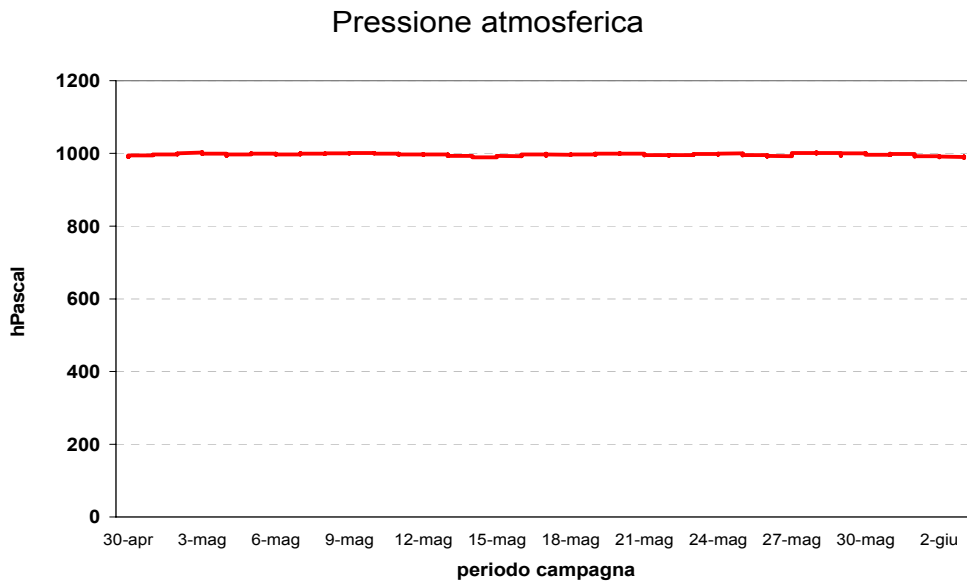
Figura 29: valori giornalieri di pressione atmosferica
