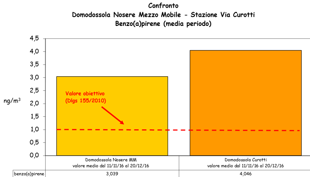
Figura 39: confronto tra Domodossola Nosere Mezzo Mobile e Stazione di Via Curotti
