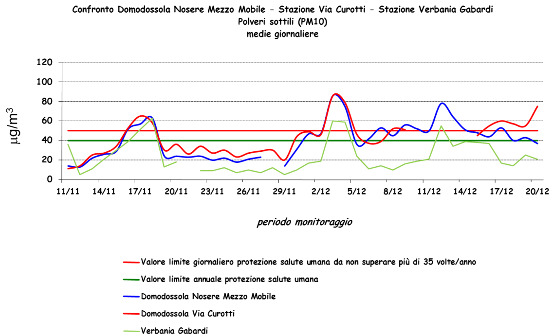
Figura 28: valori giornalieri di PM10
