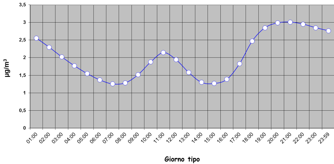
Figura 25: Benzene – giorno tipo
