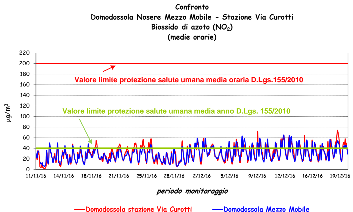
Figura 16: confronto delle medie orarie di Biossido di Azoto
