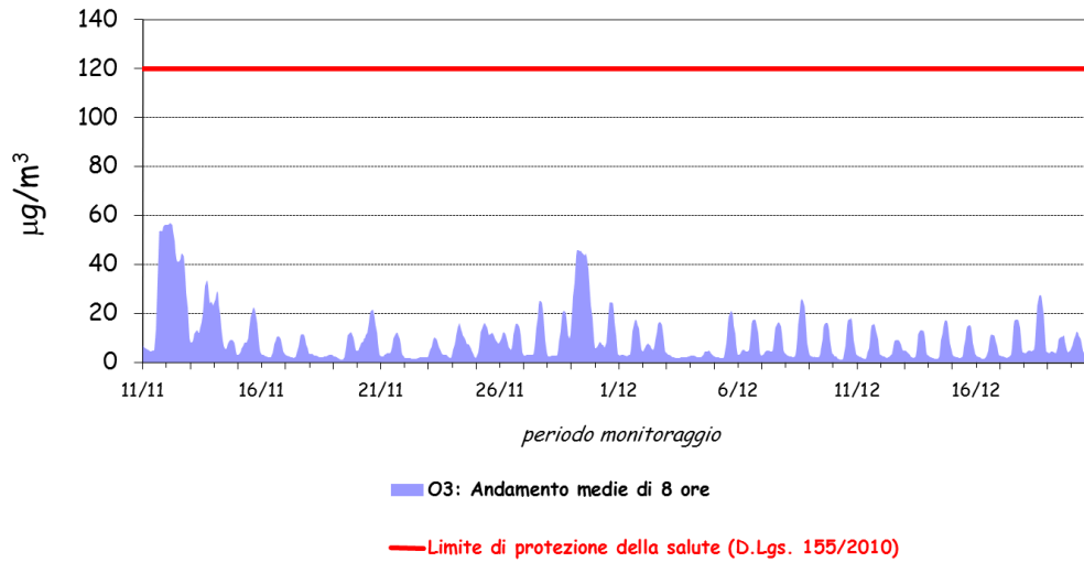
Figura 21: medie mobili otto ore Ozono
