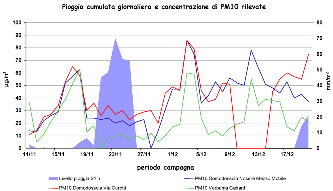
Figura 30: pioggia cumulata giornaliera e concentrazione di PM10 rilevata nelle stazioni di interesse
