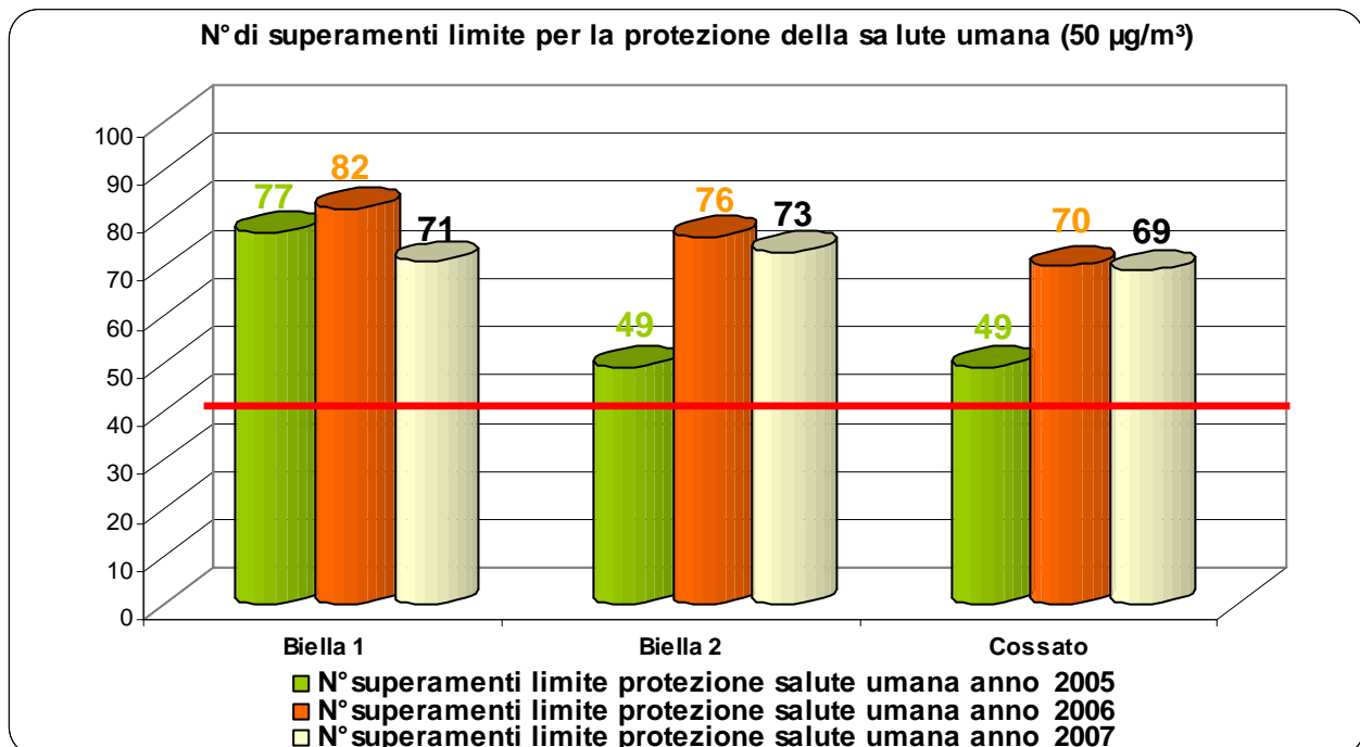
Figura 22: Numero di superamenti del valore limite della protezione della salute umana rilevati nel 2005, 2006 e 2007
