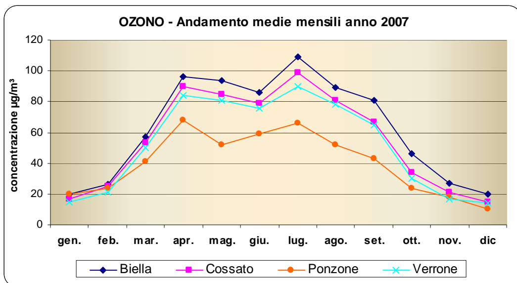
Figura 16: Andamento delle medie mensili rilevate nel corso del 2007
