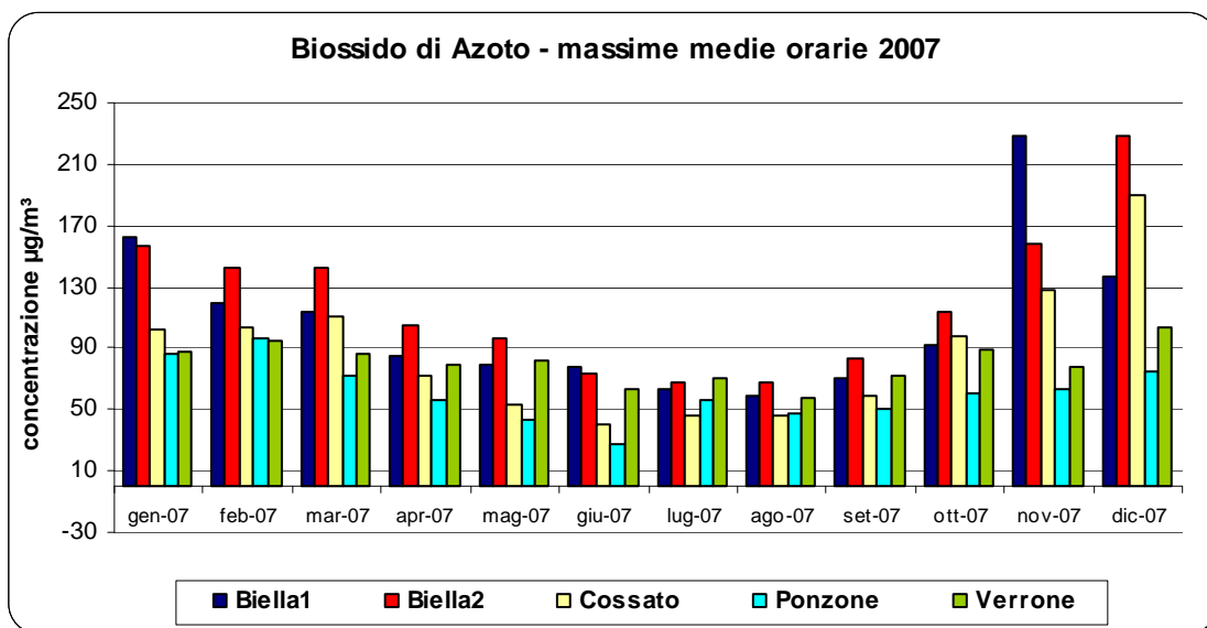
Figura 13: Andamento dei massimi delle medie orarie rilevate nel corso del 2007
