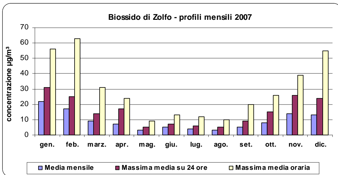
Figura 7: Andamento delle medie mensili rilevate nel corso del 2007
