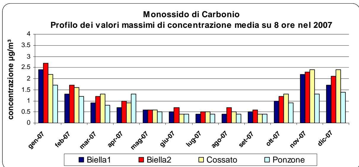
Figura 10: Andamento dei massimi di concentrazione della media mobile su otto ore registrate nel corso del 2007
