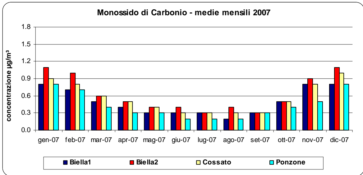
Figura 9: Medie mensili registrate nel corso del 2007
