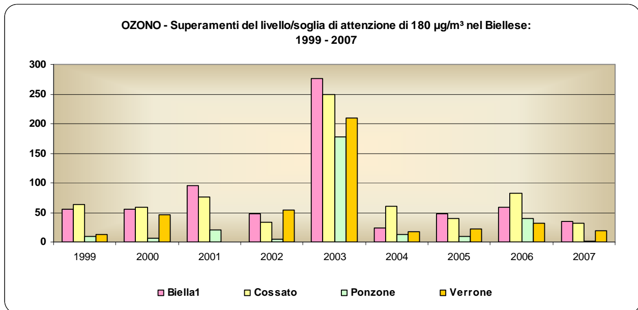
Figura 19: Numero di superamenti del livello/soglia di attenzione di 180 µg/m 3 dal 1999 al 2007
