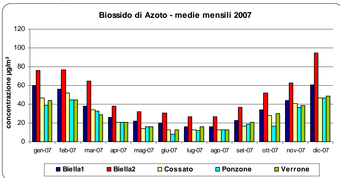
Figura 14: Andamento delle medie mensili rilevate nel corso del 2007
