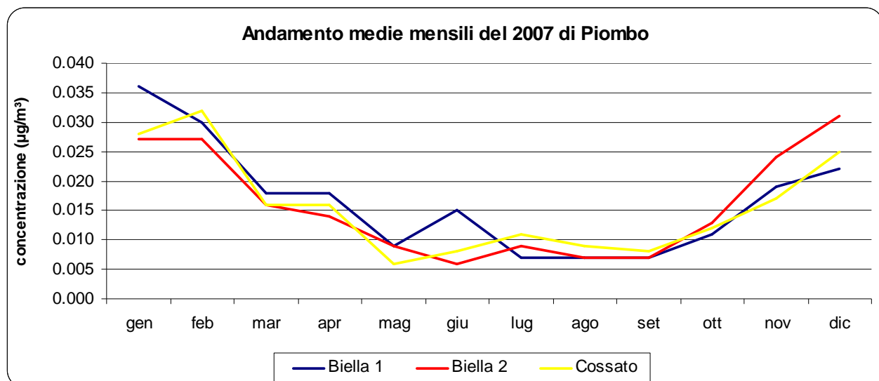
Figura 26: Andamento delle medie mensili di Piombo rilevate nel 2007
