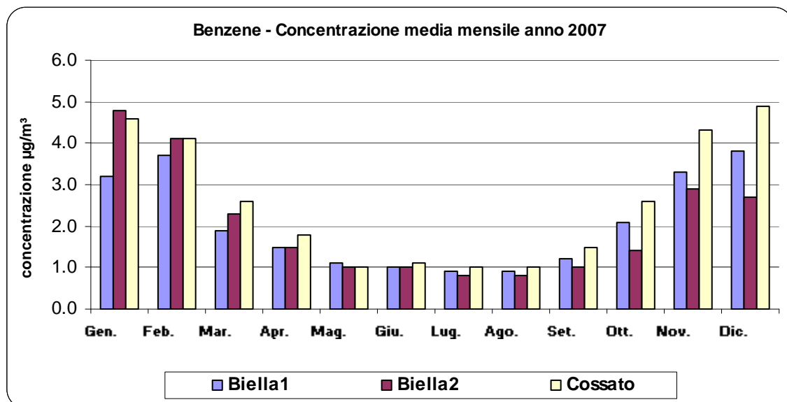
Figura 11: Andamento delle concentrazioni medie mensili registrate nel corso del 2007
