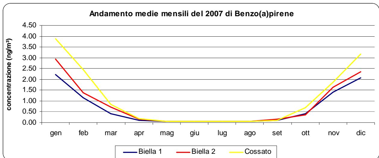
Figura 24: Andamento delle medie mensili di Benzo[a]pirene rilevate nel 2007
