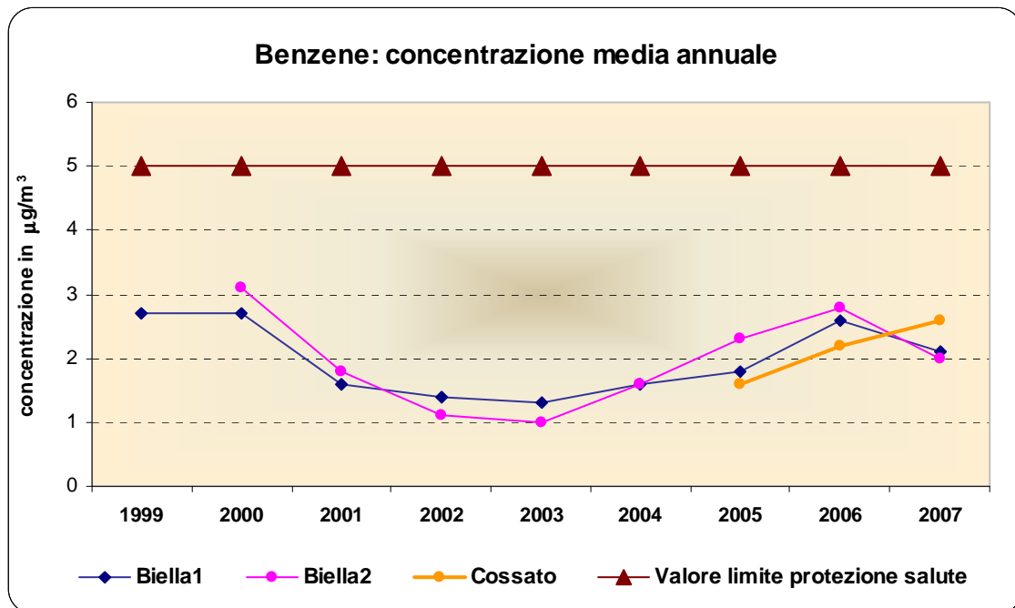
Figura 12: Andamento delle concentrazioni medie annuali rilevate dal 1999 al 2007
