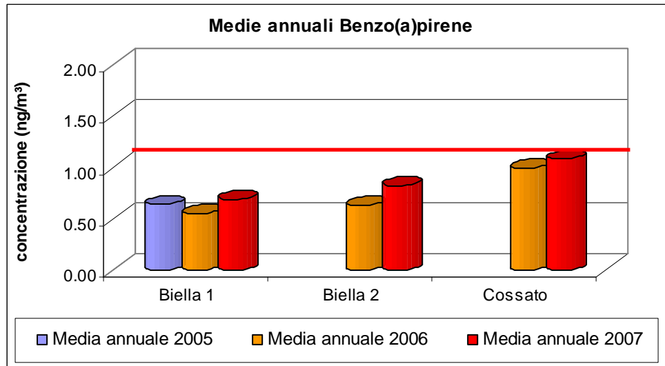
Figura 25: Andamento delle medie annuali di Benzo[a]pirene rilevate nel 2005, 2006 e 2007
