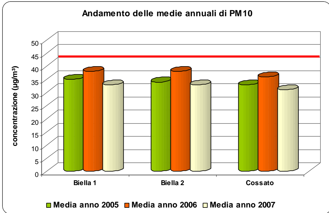
Figura 23: Andamento delle medie annuali di PM10
