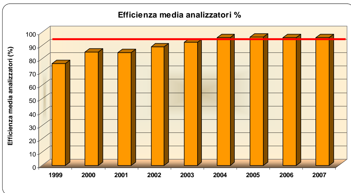
Figura 28: Efficienza annuale media degli analizzatori dal 1999 al 2007
