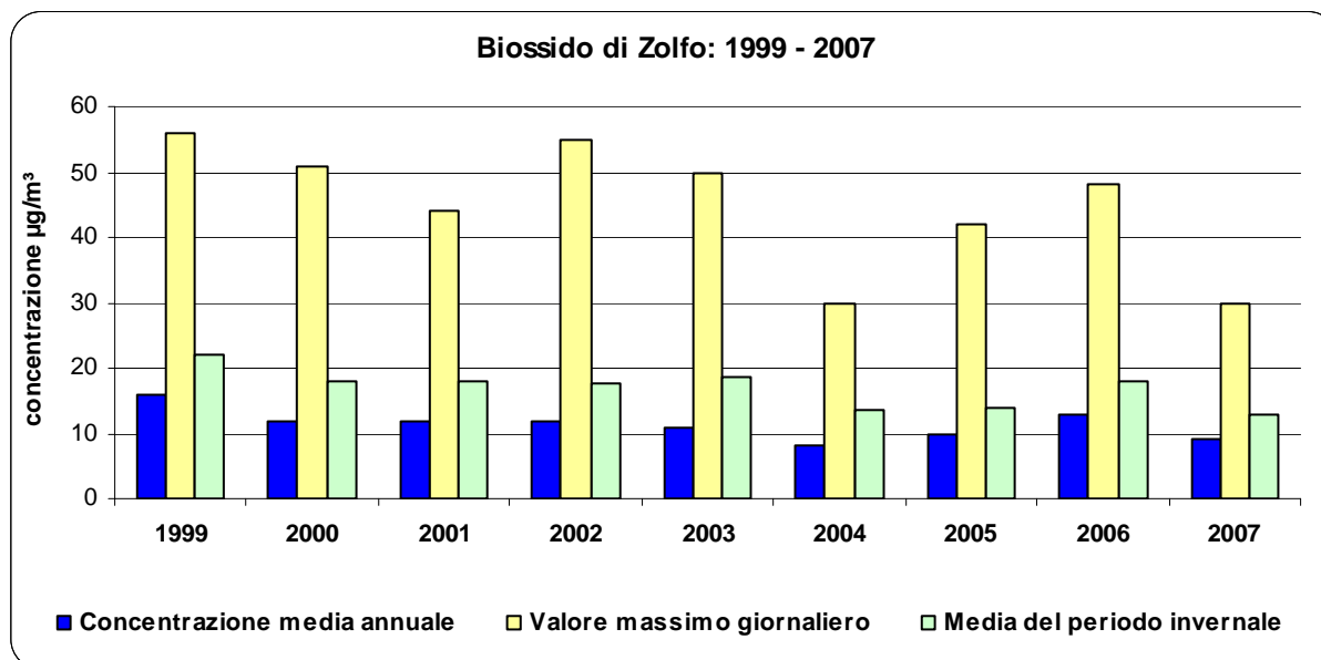
Figura 8: Valori massimi giornalieri, medi del periodo invernale e medie annuali dal 1999 al 2007
