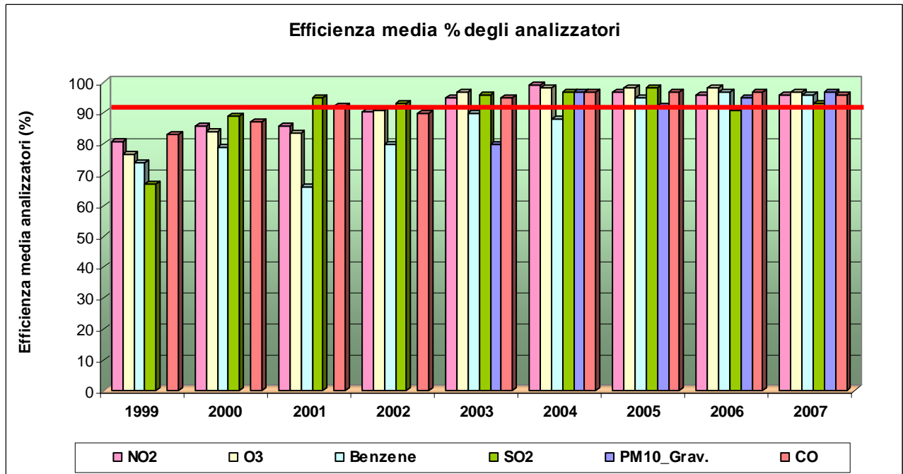
Figura 29: Efficienza annuale media di ciascun analizzatore dal 1999 al 2007
