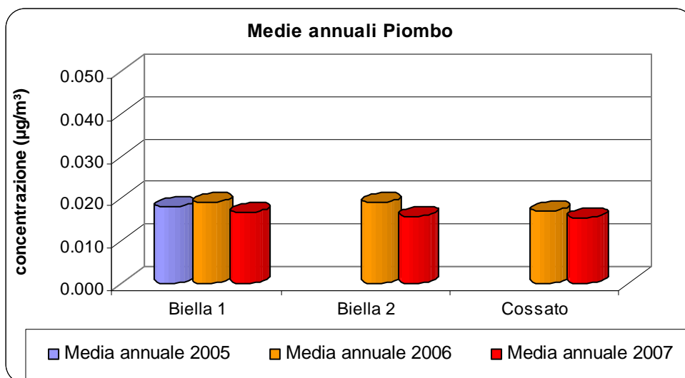
Figura 27: Andamento delle medie annuali di Piombo rilevate nel 2005, 2006 e 2007
