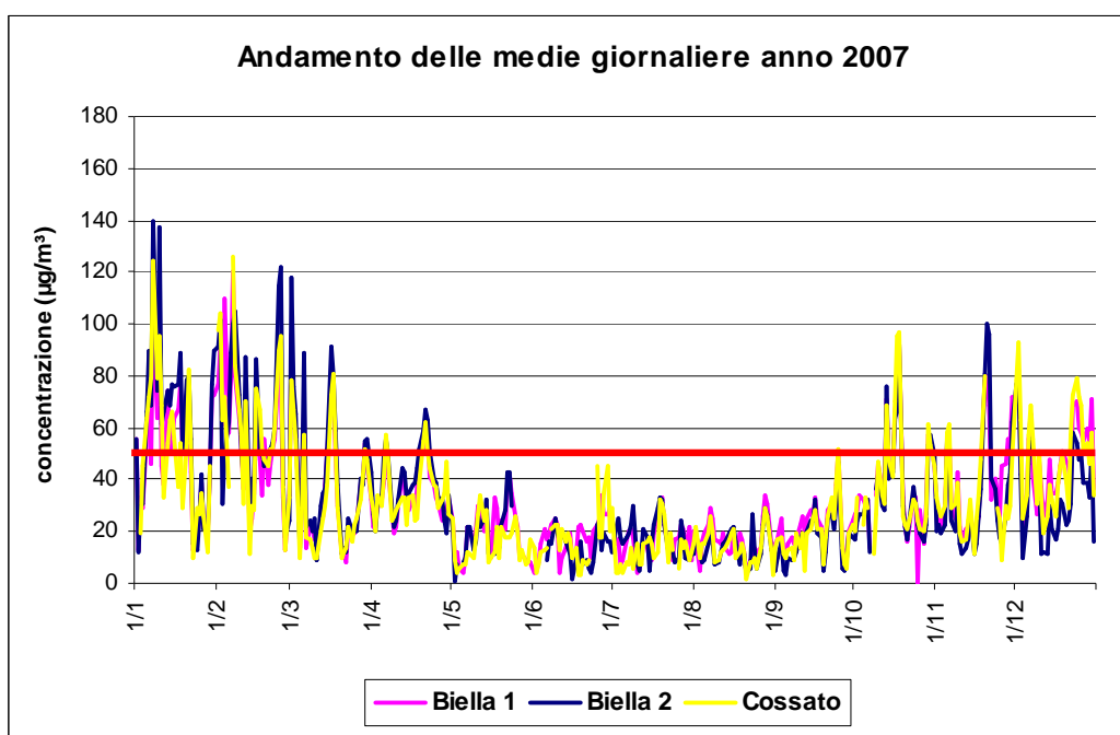
Figura 21: Andamento delle medie giornaliere di PM10 rilevate nel 2007
