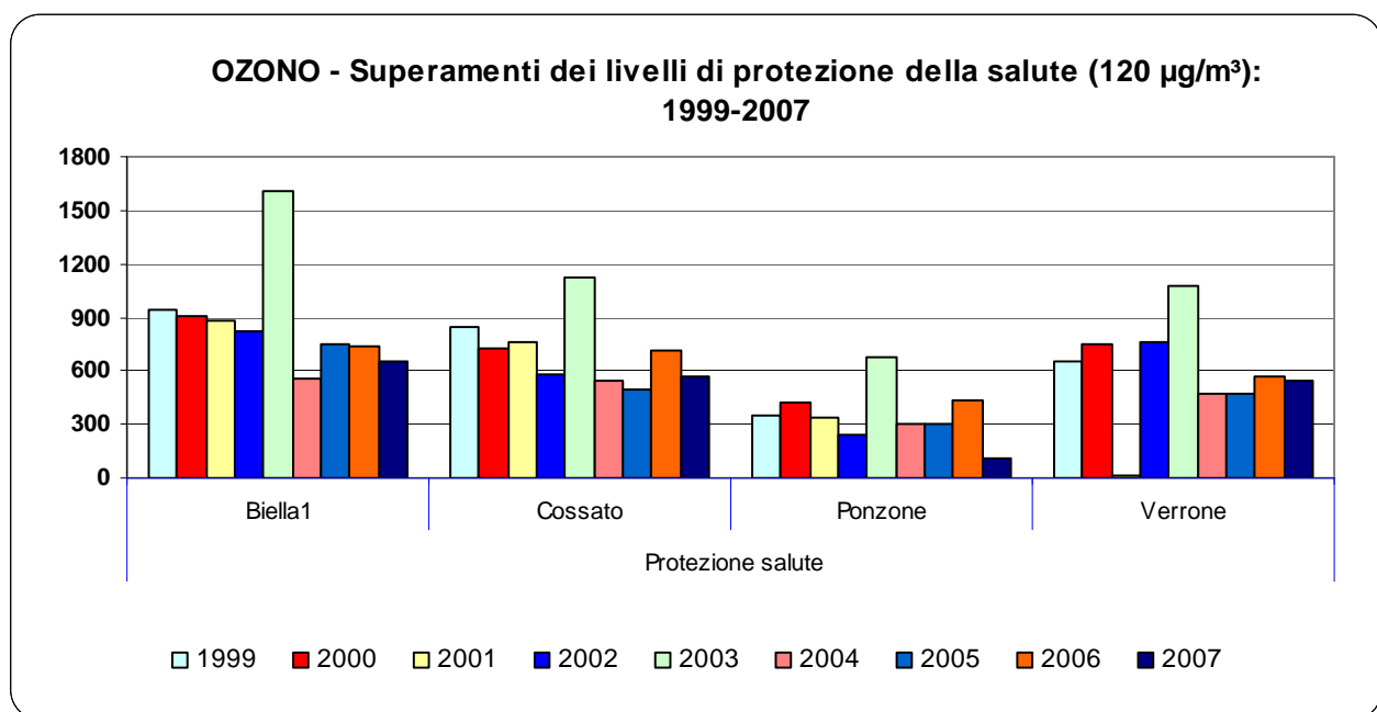
Figura 20: Numero di superamenti del livello protezione della salute su medie di 8 ore di 120 \mu\text{g}/\text{m}^3 dal 1999 al 2007
