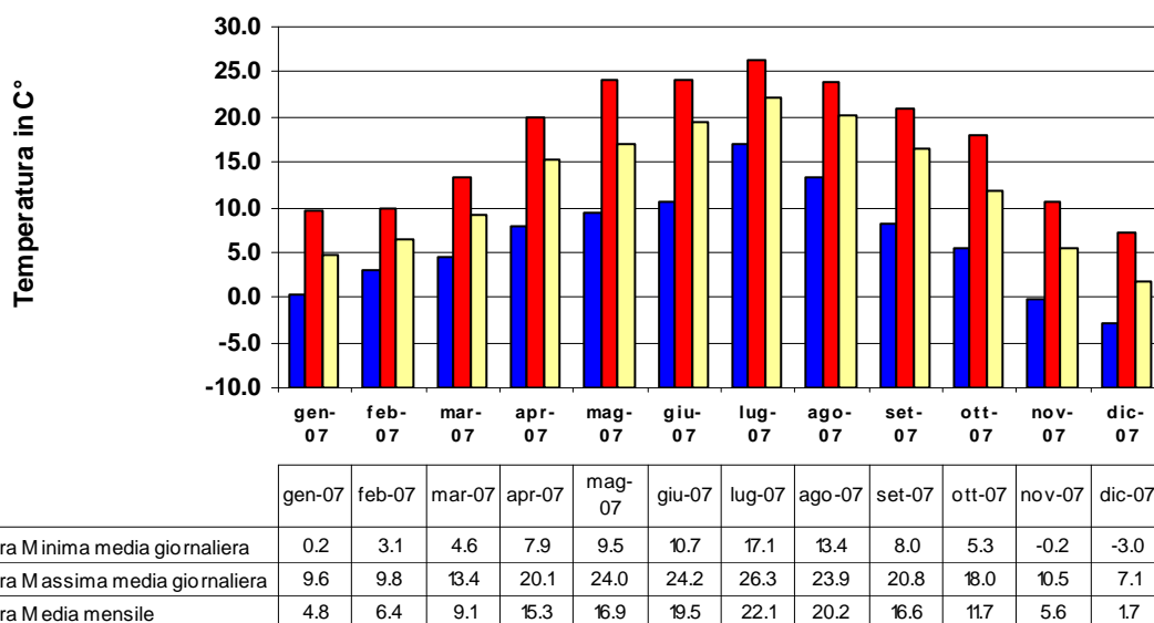
Temperatura dell'Aria media, minima e massima nella Provincia di Biella nel 2007
