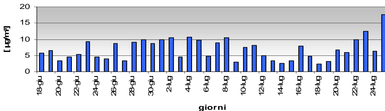
Biossido di Zolfo Media giornaliera del periodo
