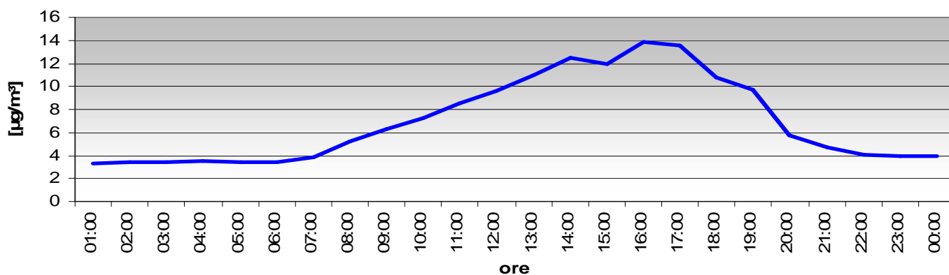
Andamento giorno medio - Biossido di Zolfo
