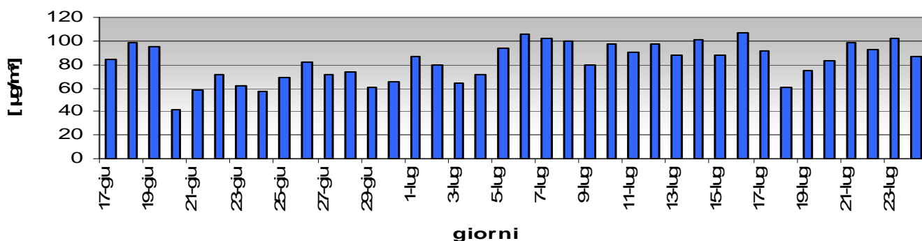
Ozono Media giornaliera del periodo
