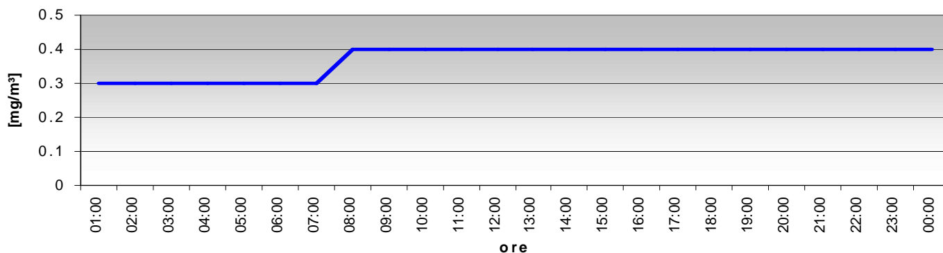
Andamento giorno medio - Monossido di Carbonio
