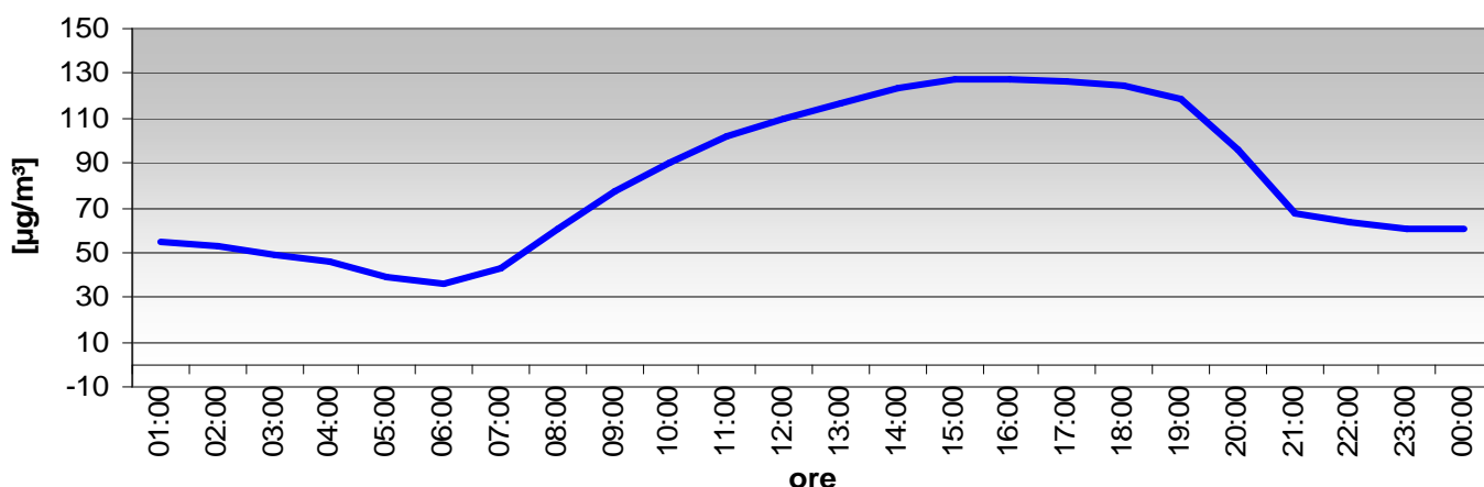
Andamento giorno medio - Ozono
