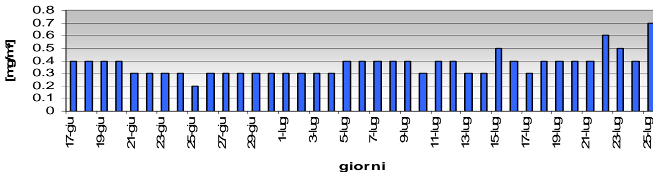
Monossido di Carbonio Media giornaliera del periodo
