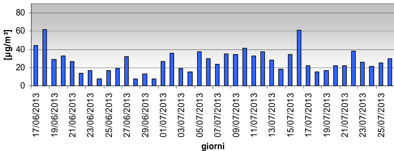
Andamento giornaliero PM10
