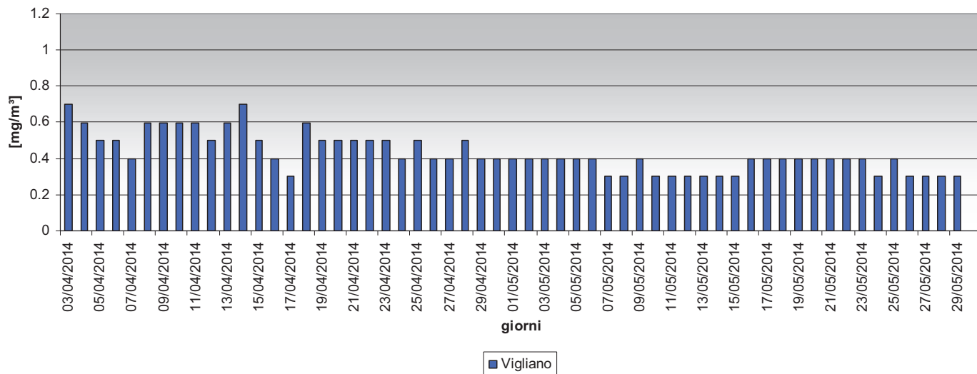
Monossido di Carbonio Media giornaliera del periodo
