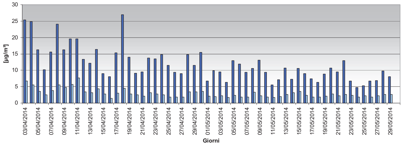
Ossidi di Azoto Media giornaliera del periodo
