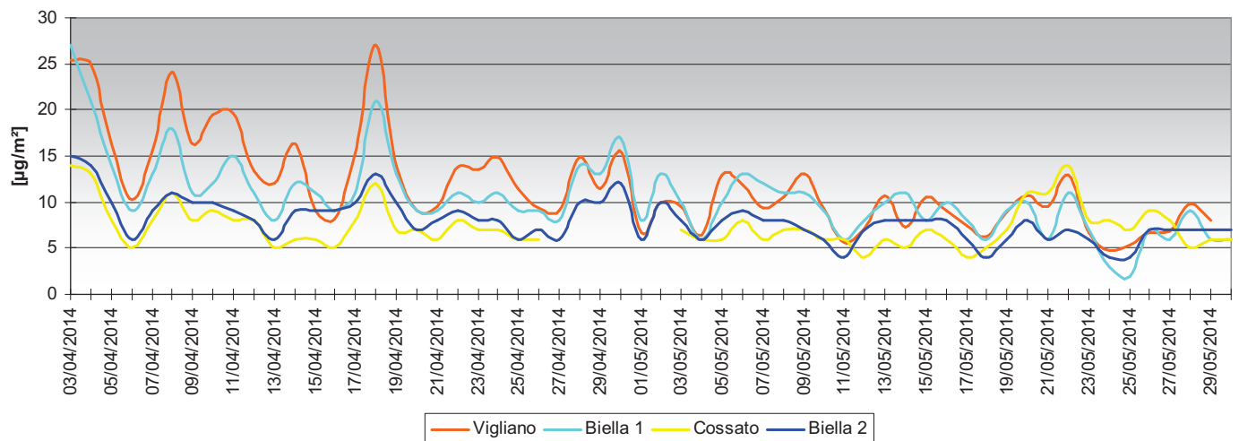
Ossidi di Azoto Confronto tra MM e altre stazioni
