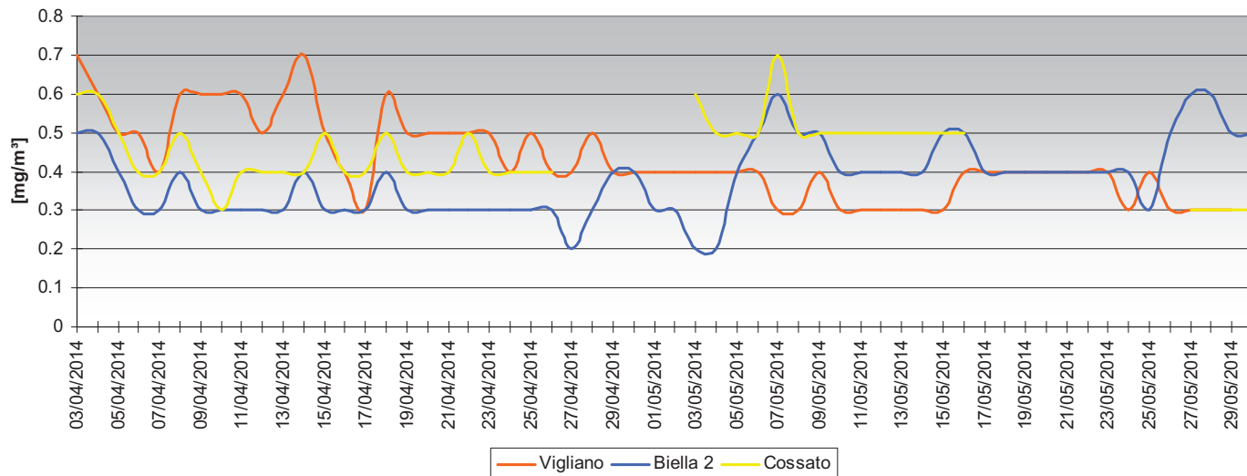
Monossido di Carbonio Confronto MM e altre stazioni
