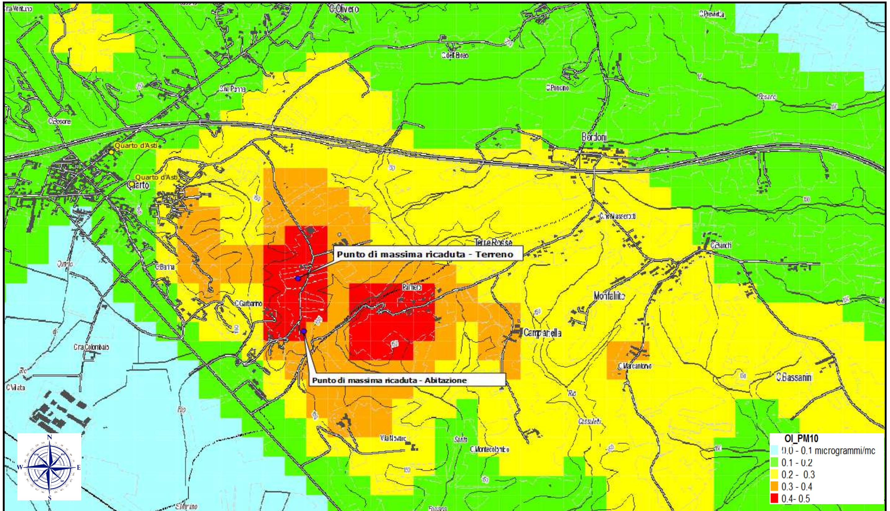
Dettaglio distribuzione delle concentrazioni medie annue PM10 ( \mu\text{g}/\text{m}^3 )
