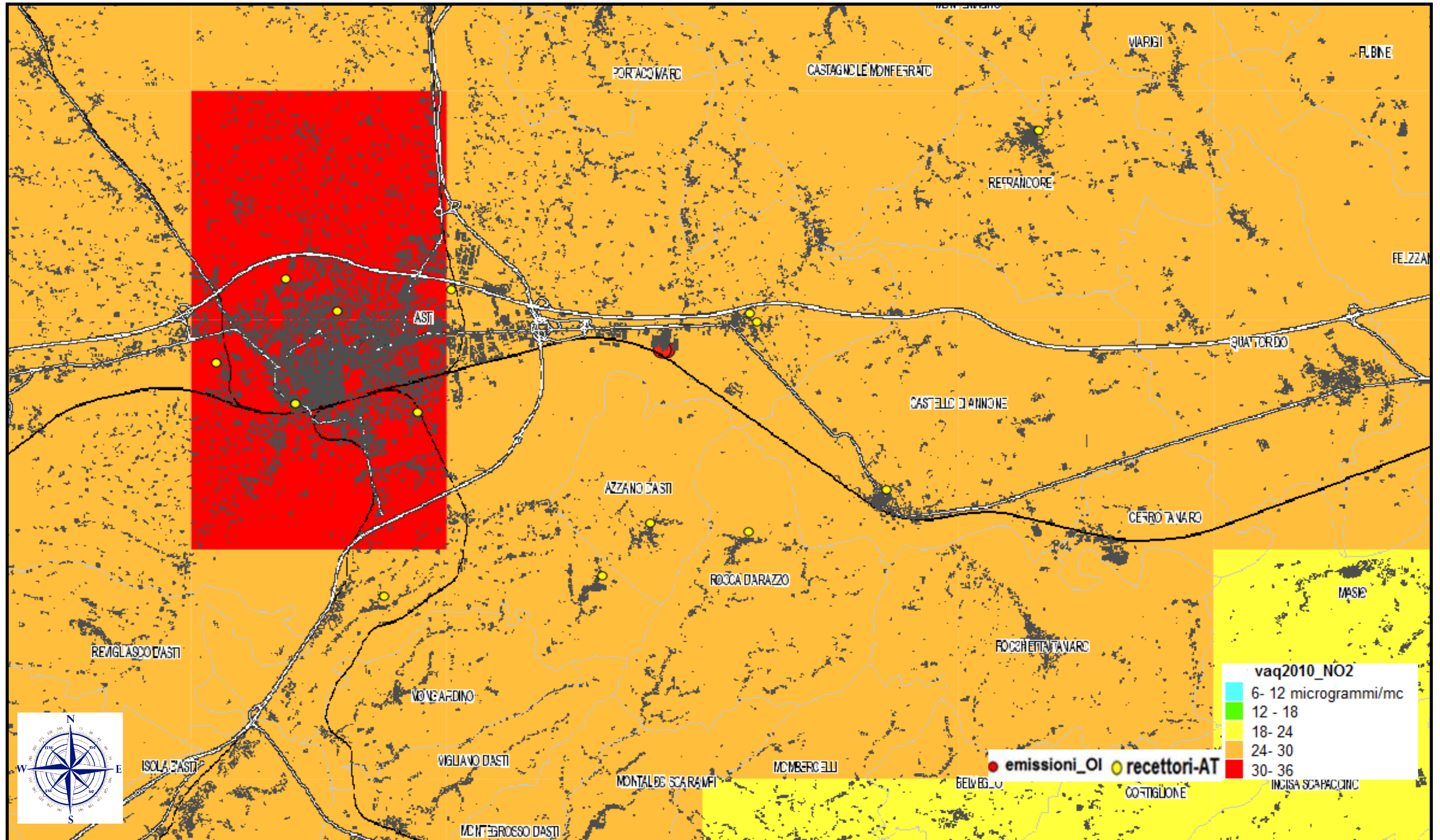
Distribuzione delle concentrazioni medie annue NO 2 (µg/m 3 ) – VAQ2010
