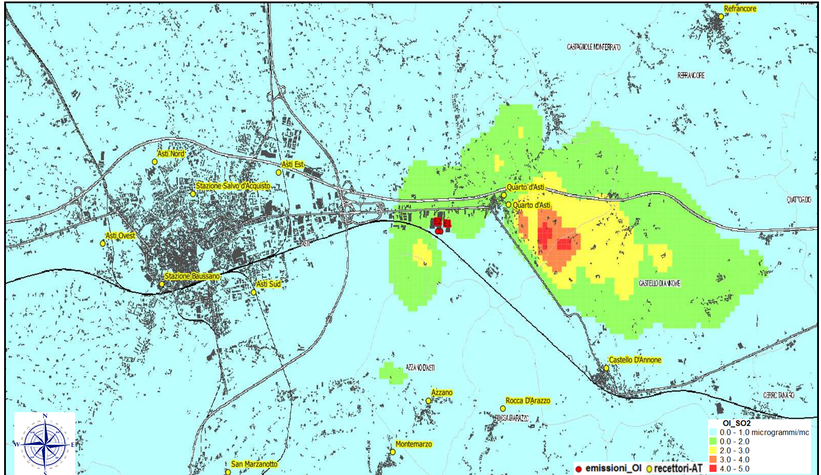
Distribuzione delle concentrazioni medie annue SO 2 (µg/m 3 )
