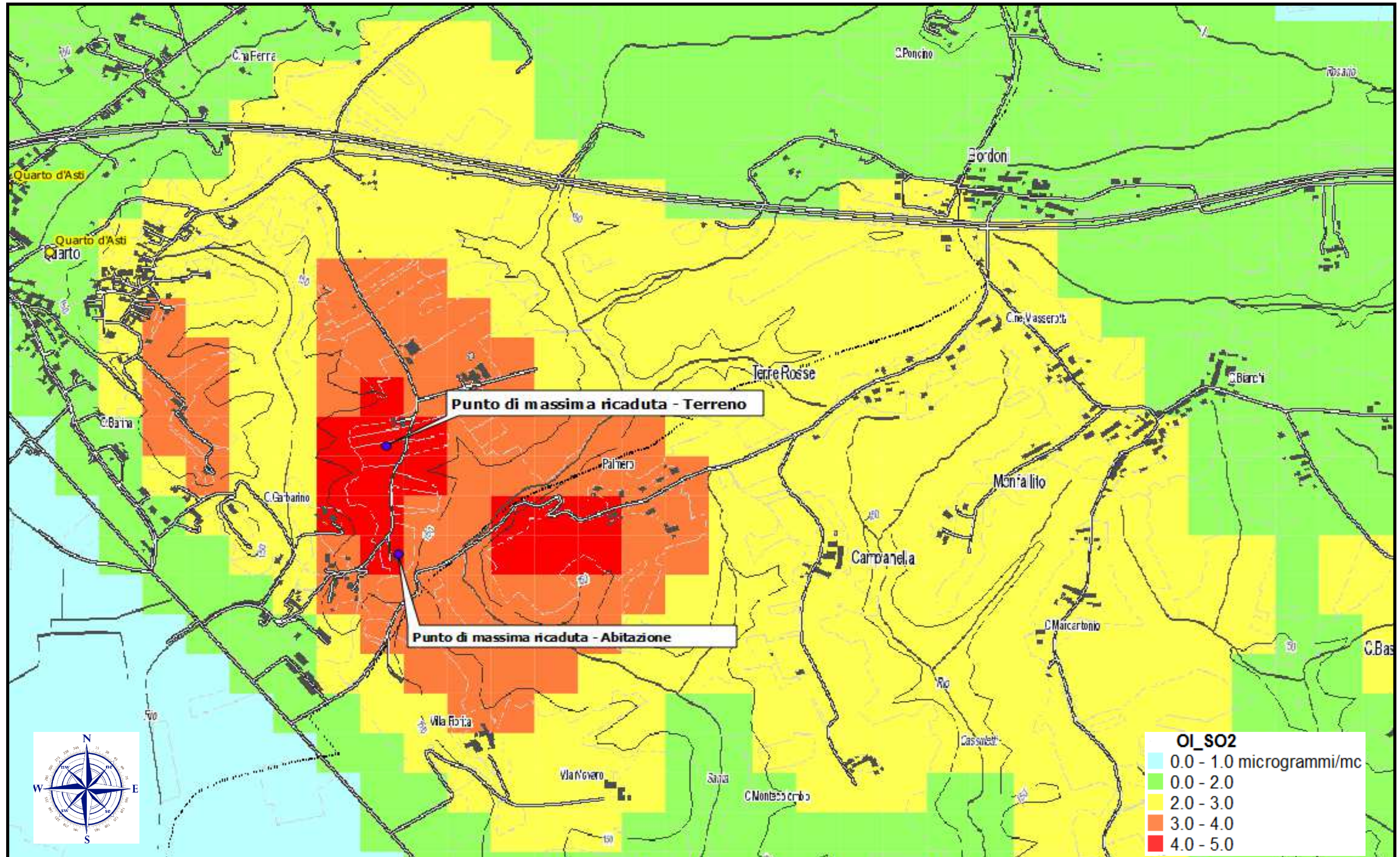
Dettaglio distribuzione delle concentrazioni medie annue SO 2 (µg/m 3 )
