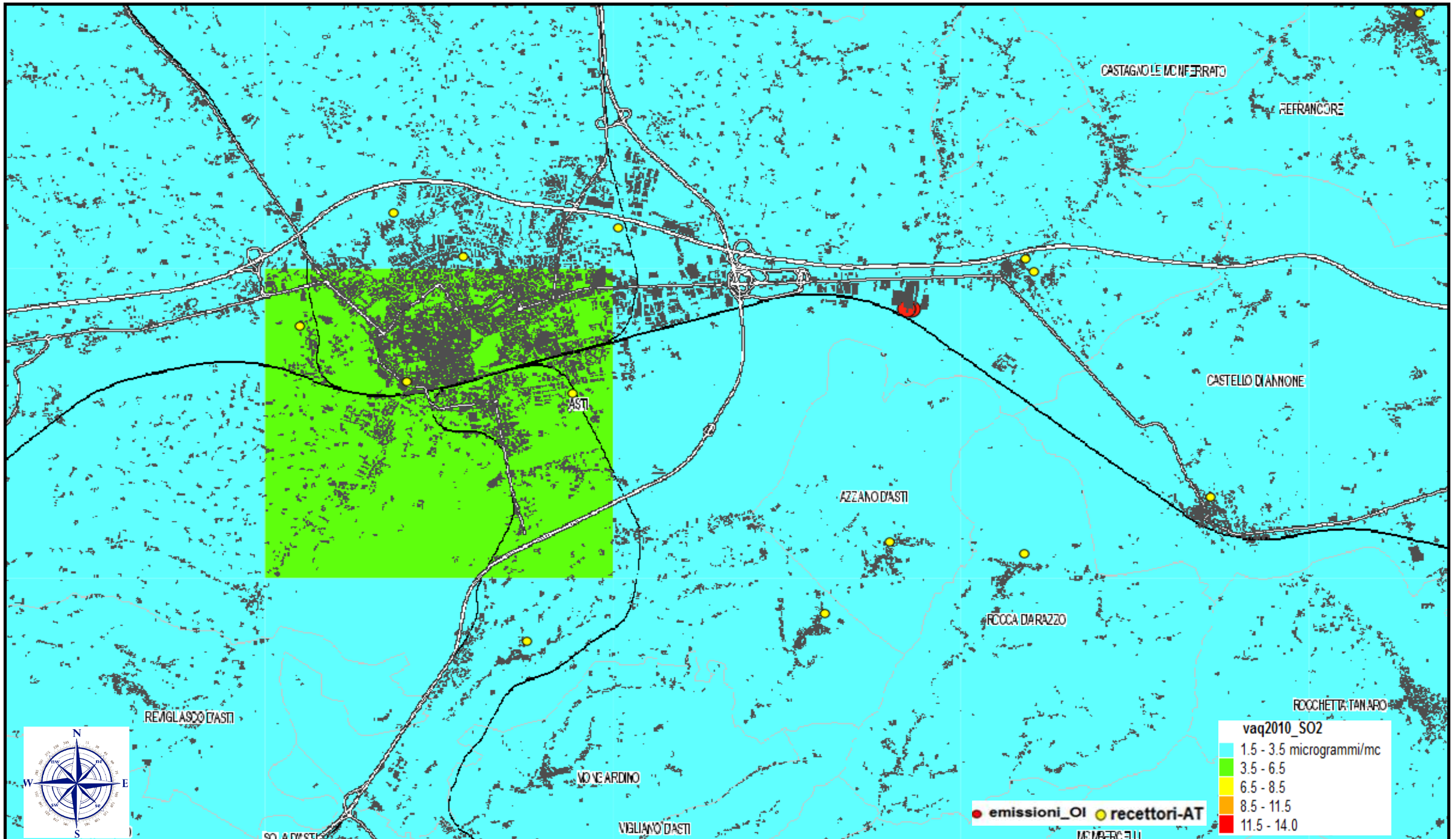
Distribuzione delle concentrazioni medie annue SO 2 (µg/m 3 ) – VAQ2010
