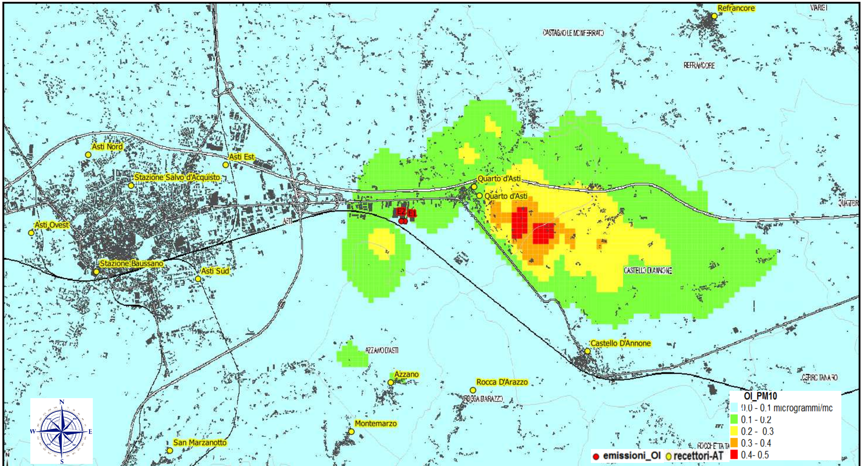
Distribuzione delle concentrazioni medie annue PM10 ( \mu\text{g}/\text{m}^3 )
