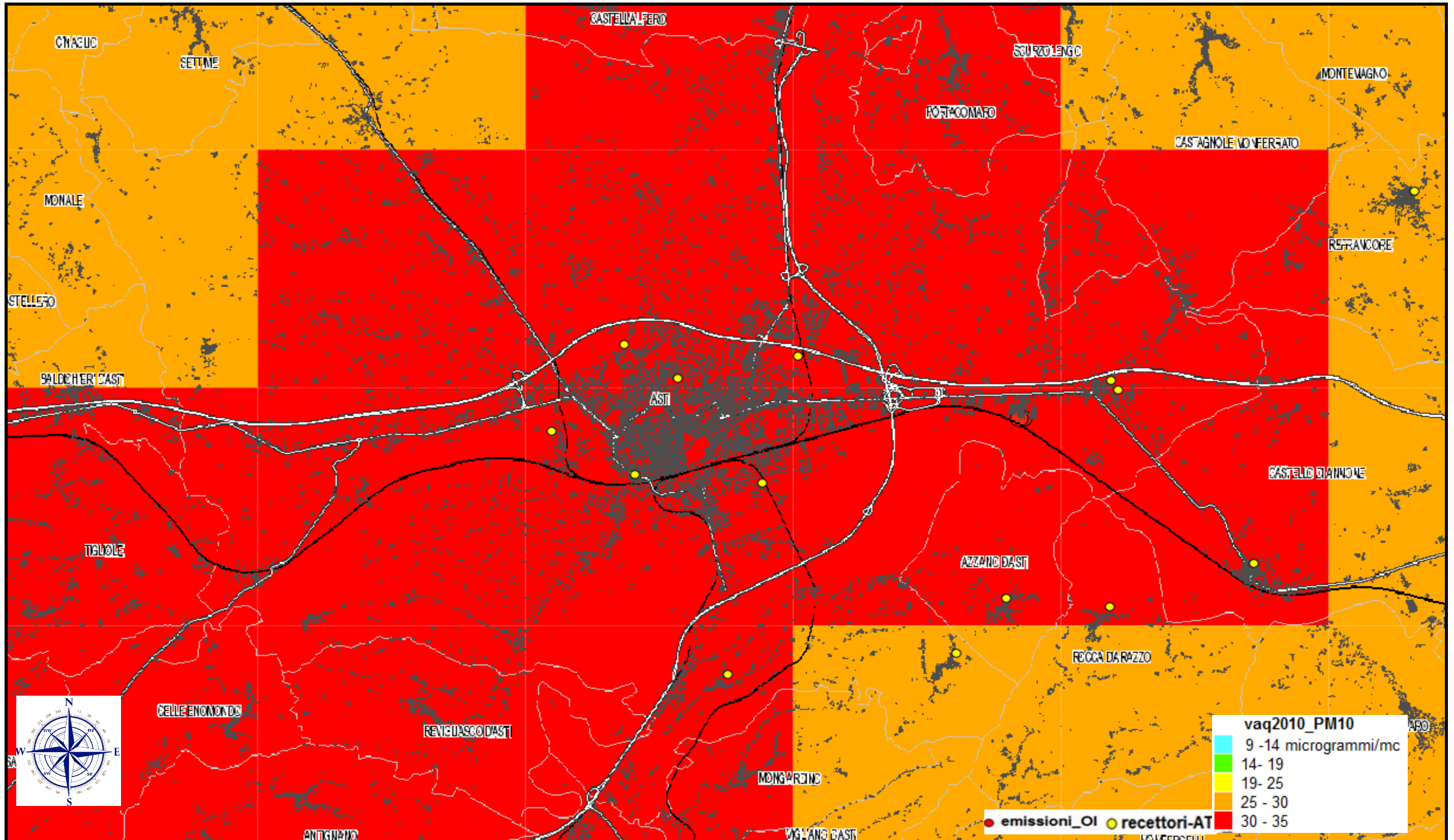
Distribuzione delle concentrazioni medie annue PM10 ( \mu\text{g}/\text{m}^3 ) – VAQ2010
