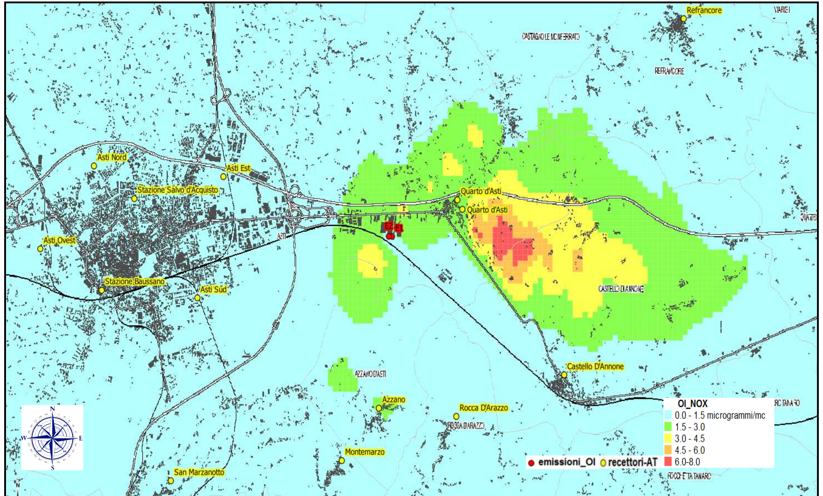
Distribuzione delle concentrazioni medie annue NO 2 (µg/m 3 )
