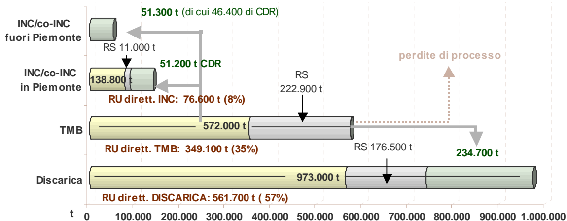
Figura 4 – Destinazione dei rifiuti urbani indifferenziati – schema di flusso principale
