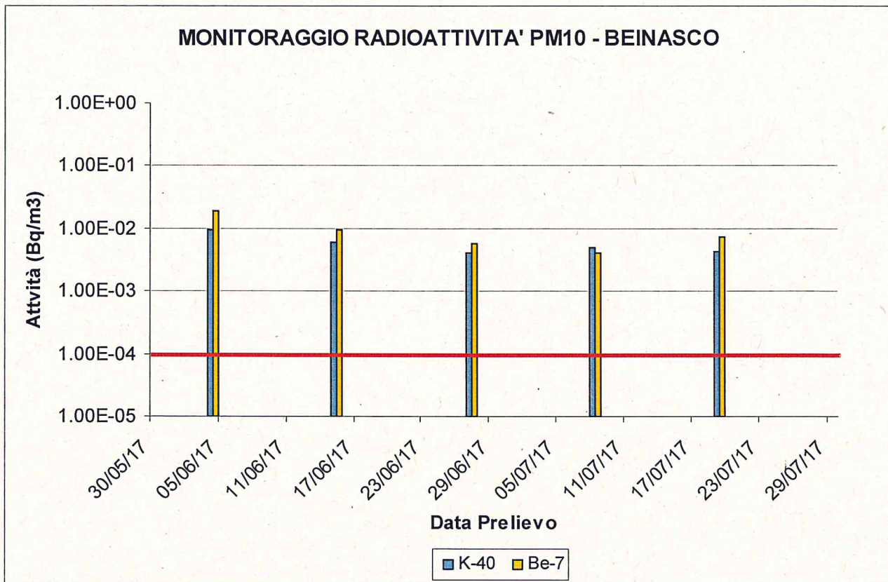
Figura 2. Concentrazioni di attività dei radionuclidi naturali ^{40}\text{K} e ^7\text{Be} rilevate nelle tre aliquote di filtri campionati nel periodo 31 maggio – 25 luglio nella stazione di monitoraggio di Beinasco. La linea rossa rappresenta il valore indicativo del livello minimo di rilevabilità della catena di misura
