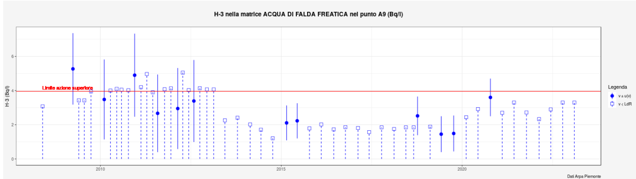
Figura 5.12. Andamento della concentrazione di H-3 nell'acqua di falda superficiale campionata nel punto A9 (Bq/l) – La linea rossa rappresenta il limite di azione pertinente.
