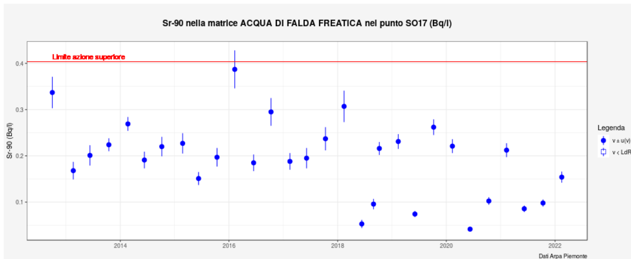
Figura 5.8. Andamento della concentrazione di Sr-90 nell'acqua di falda superficiale campionata nel punto SO17 (Bq/l) – La linea rossa rappresenta il limite di azione pertinente.
