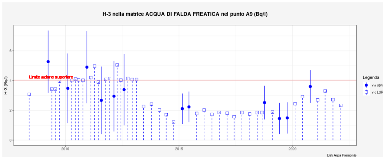
Figura 5.12. Andamento della concentrazione di H-3 nell'acqua di falda superficiale campionata nel punto A9 (Bq/l) – La linea rossa rappresenta il limite di azione pertinente.
