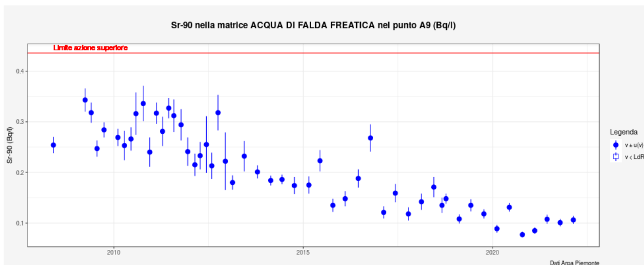
Figura 5.9. Andamento della concentrazione di Sr-90 nell'acqua di falda superficiale campionata nel punto A9 (Bq/l) – La linea rossa rappresenta il limite di azione pertinente.
