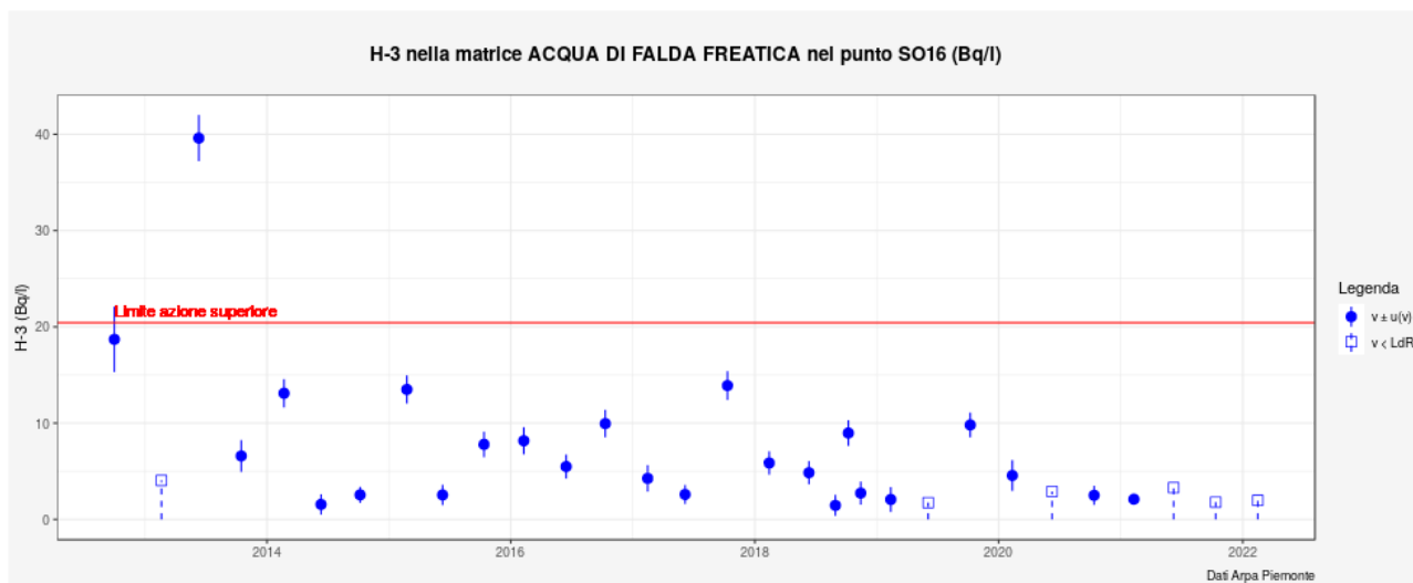
Figura 5.11. Andamento della concentrazione di H-3 nell'acqua di falda superficiale campionata nel punto SO16 (Bq/l) – La linea rossa rappresenta il limite di azione pertinente.
