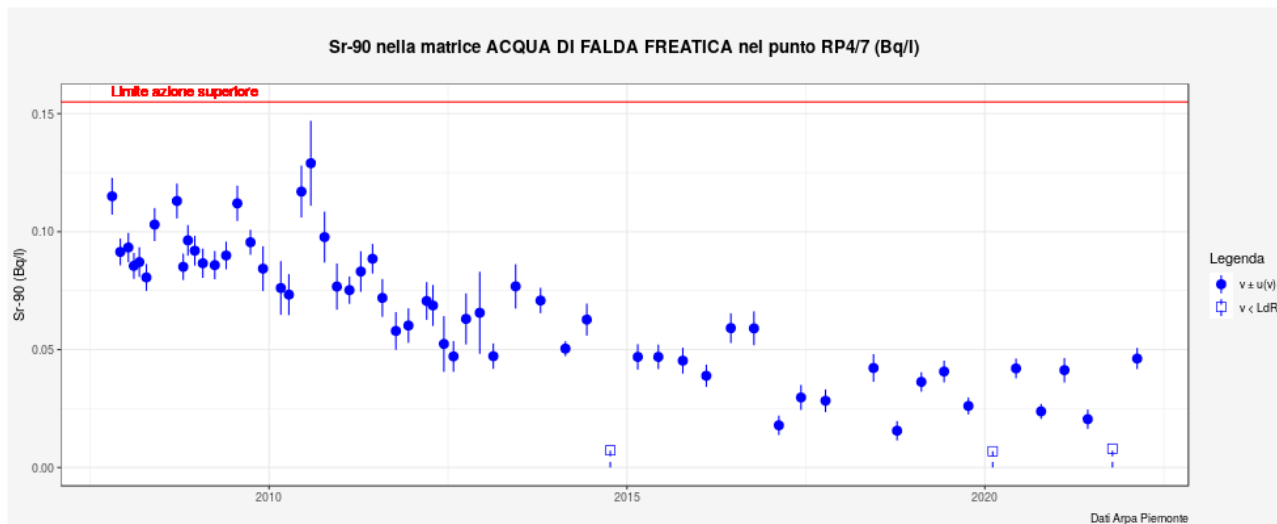
Figura 5.2. Andamento della concentrazione di Sr-90 nell'acqua di falda superficiale campionata nel punto RP4/7 (Bq/l) – La linea rossa rappresenta il limite di azione pertinente.
