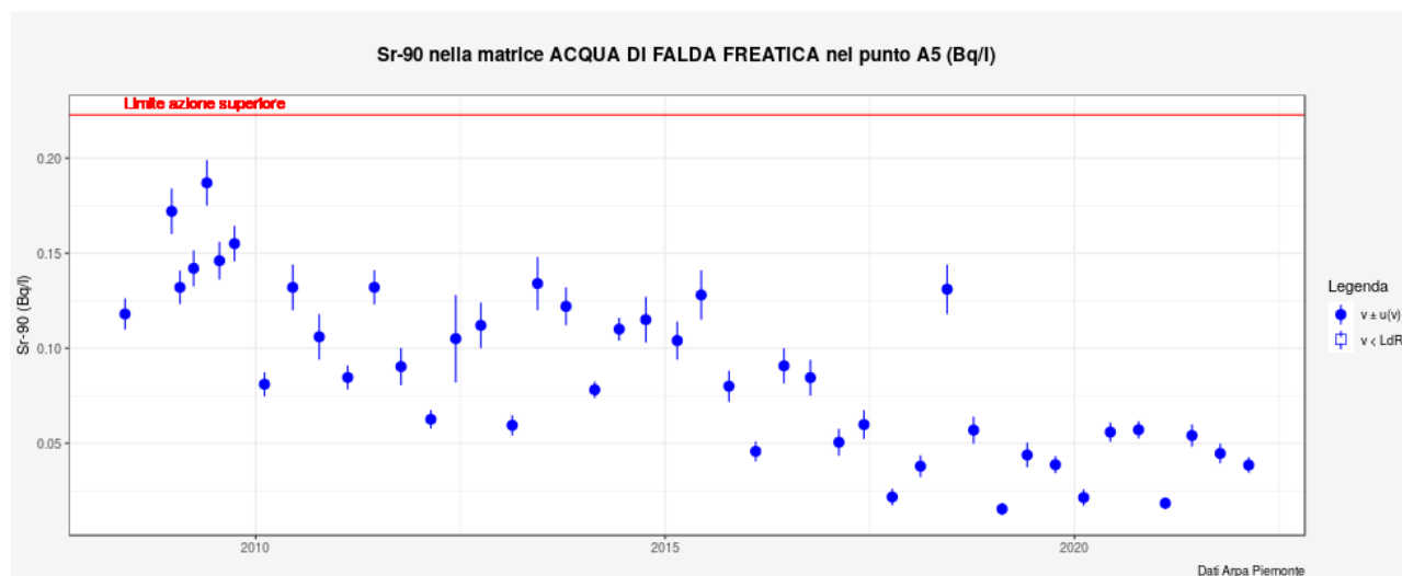
Figura 5.7. Andamento della concentrazione di Sr-90 nell'acqua di falda superficiale campionata nel punto A5 (Bq/l) – La linea rossa rappresenta il limite di azione pertinente.
