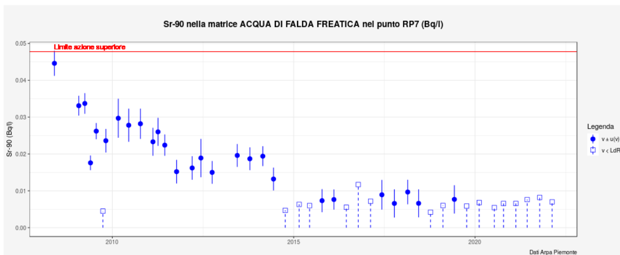
Figura 5.3. Andamento della concentrazione di Sr-90 nell'acqua di falda superficiale campionata nel punto RP7 (Bq/l) – La linea rossa rappresenta il limite di azione pertinente.
