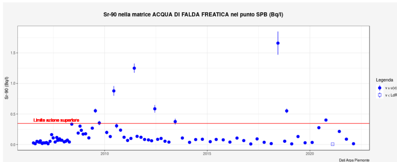
Figura 5.4. Andamento della concentrazione di Sr-90 nell'acqua di falda superficiale campionata nel punto SPB (Bq/l) – La linea rossa rappresenta il limite di azione pertinente.
