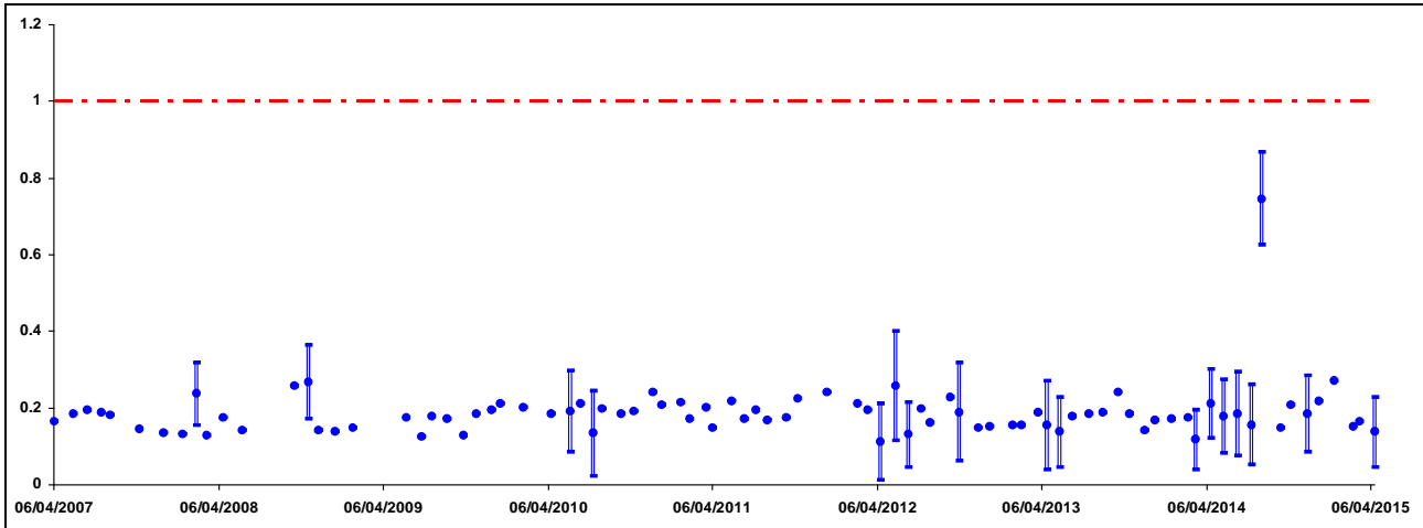
Figura 5.2 Andamento della concentrazione Beta totale nell'acqua potabile prelevata nel punto SQ05 (Bq/l) – La linea tratteggiata rossa indica il valore di screening fissato da World Health Organization
