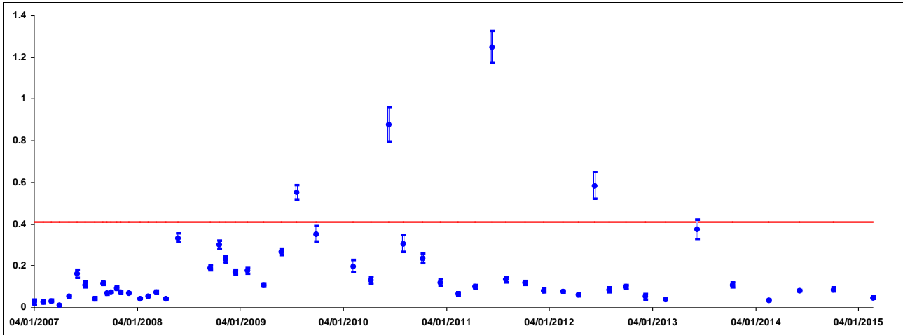
Figura 5.6 Andamento della concentrazione di Sr-90 nell'acqua di falda superficiale prelevata nel punto SPB (Bq/l) – La linea rossa rappresenta il Limite di Azione pertinente.
