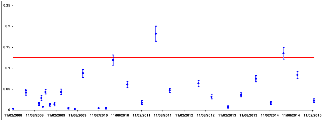
Figura 5.8 Andamento della concentrazione di Cs-137 nell'acqua di falda superficiale prelevata nel punto E5/6 (Bq/l) – La linea rossa rappresenta il Limite di Azione pertinente.
