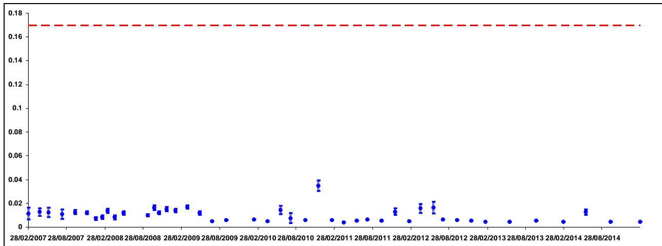
Figura 5.3 Andamento della concentrazione di Sr-90 nell'acqua di falda superficiale prelevata nel punto SP01 (Bq/l) – La linea tratteggiata rossa indica il valore soglia per la non rilevanza radiologica.
