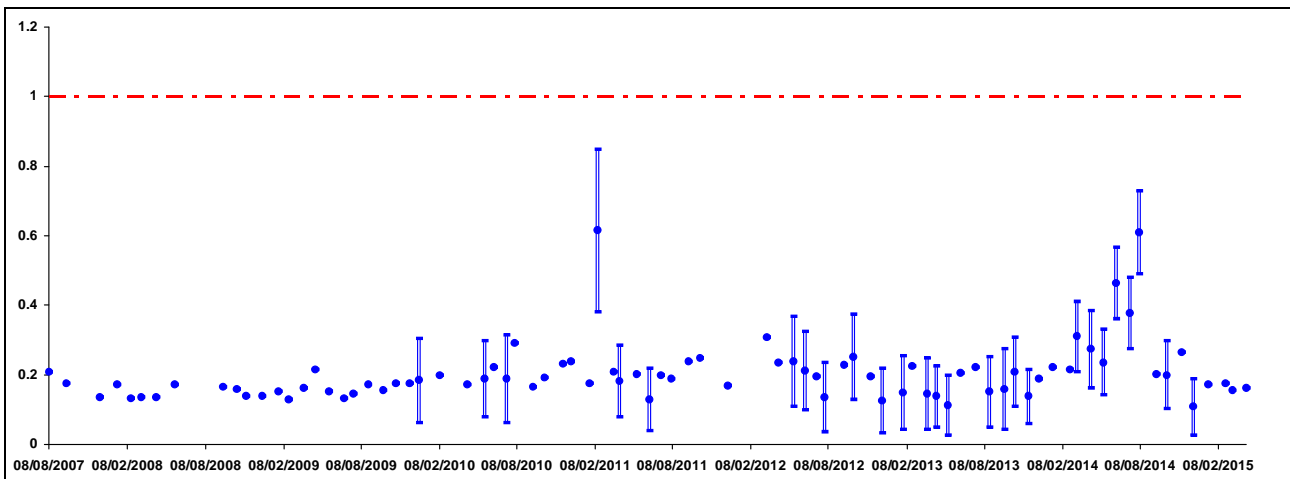
Figura 5.5 Andamento della concentrazione Beta totale nell'acqua di falda superficiale prelevata nel punto S4.1/7 (Bq/l) – La linea tratteggiata rossa indica il valore di screening fissato da World Health Organization.
