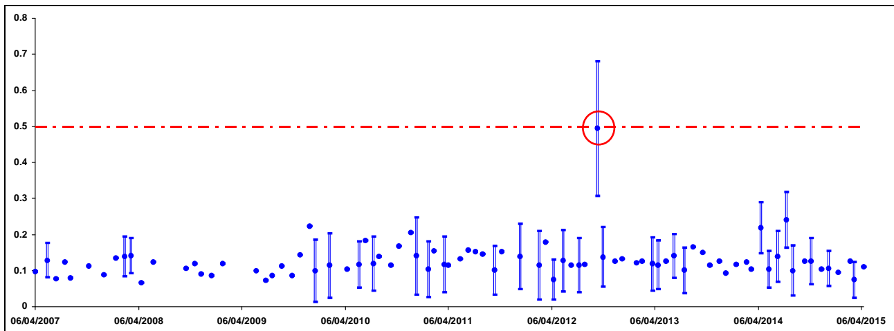
Figura 5.1 Andamento della concentrazione Alfa totale nell'acqua potabile prelevata nel punto SQ05 (Bq/l) – La linea tratteggiata rossa indica il valore di screening fissato da World Health Organization.
