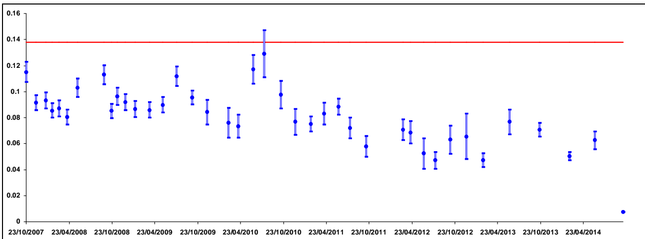
Figura 5.11 Andamento della concentrazione di Sr-90 nell'acqua di falda superficiale prelevata nel punto RP4/7 (Bq/l) – La linea rossa rappresenta il Limite di Azione pertinente.
