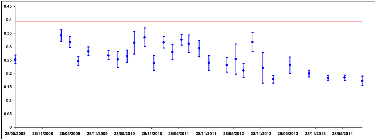
Figura 5.10 Andamento della concentrazione di Sr-90 nell'acqua di falda superficiale prelevata nel punto A9 (Bq/l) – La linea rossa rappresenta il Limite di Azione pertinente.
