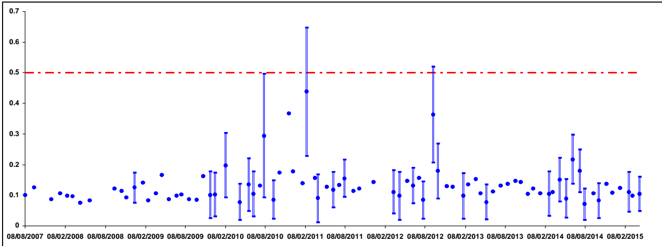
Figura 5.4 Andamento della concentrazione Alfa totale nell'acqua di falda superficiale prelevata nel punto S4.1/7 (Bq/l) – La linea tratteggiata rossa indica il valore di screening fissato da World Health Organization.
