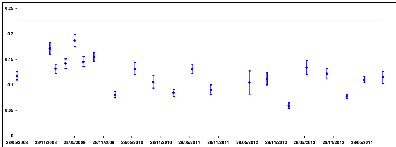
Figura 5.9 Andamento della concentrazione di Sr-90 nell'acqua di falda superficiale prelevata nel punto A5 (Bq/l) – La linea rossa rappresenta il Limite di Azione pertinente.
