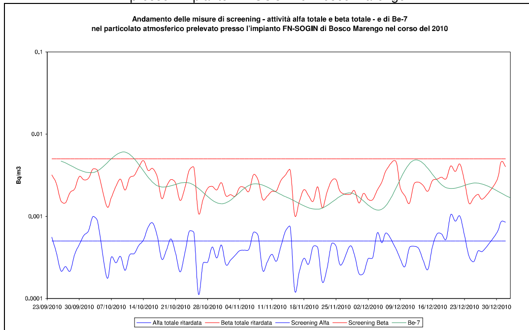
Figura 9.4 Andamento delle misure di screening e di Be-7 sui campioni di particolato atmosferico prelevati presso l'impianto FN-SOGIN di Bosco Marengo.
