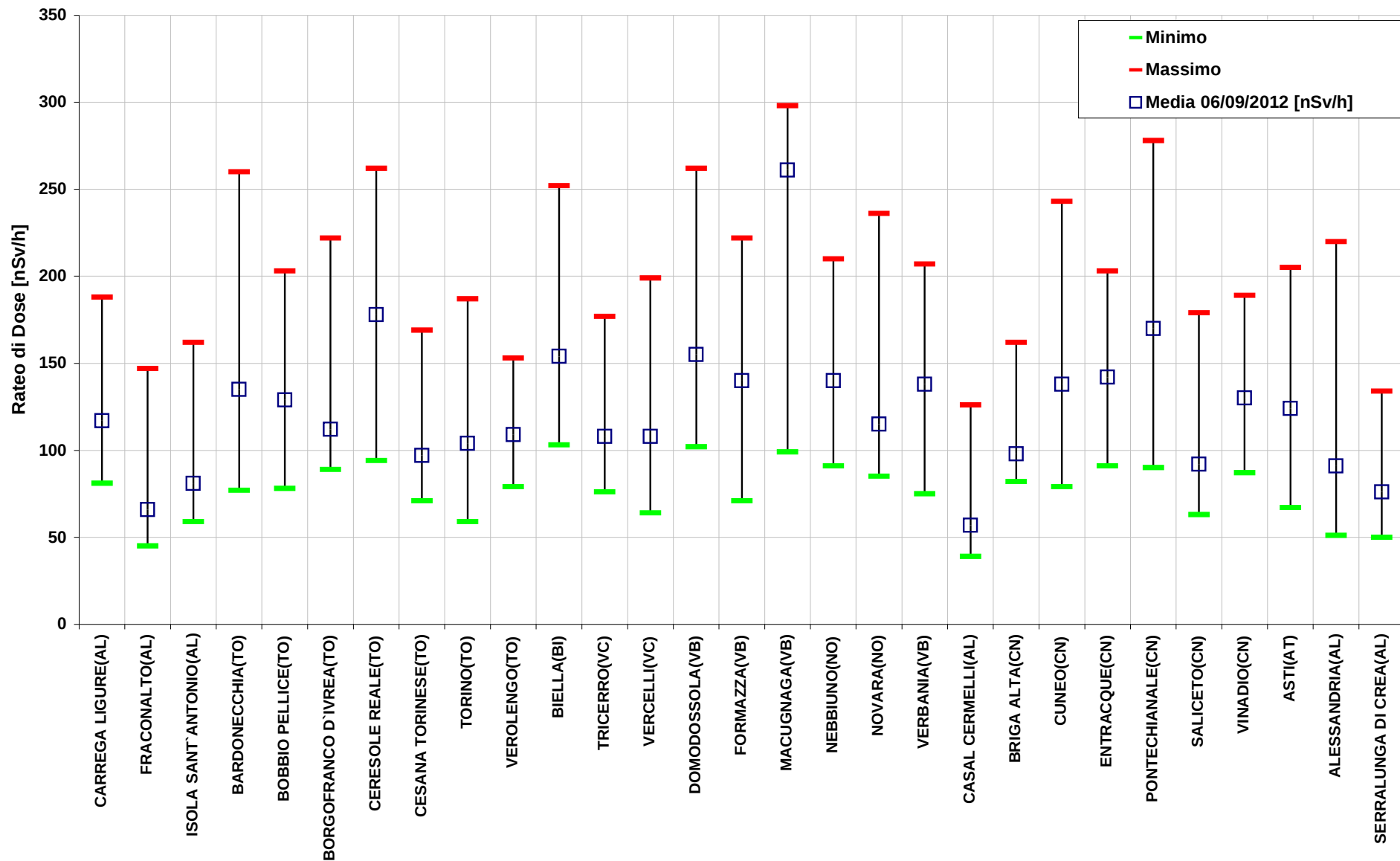
Gráfico 1). Rateo di dose gamma misurato nelle stazioni di rilevamento della rete di ARPA Piemonte nella giornata del 06 settembre 2012.
