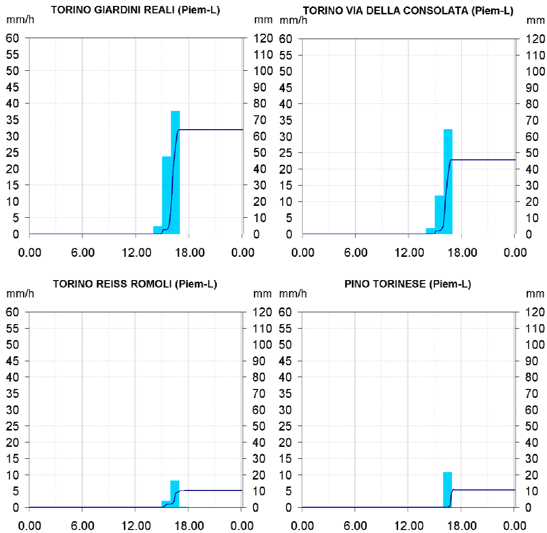
Figura 9. Ietogrammi di pioggia oraria e cumulata registrati il 20 giugno 2007 nelle stazioni pluviometriche più significative.
