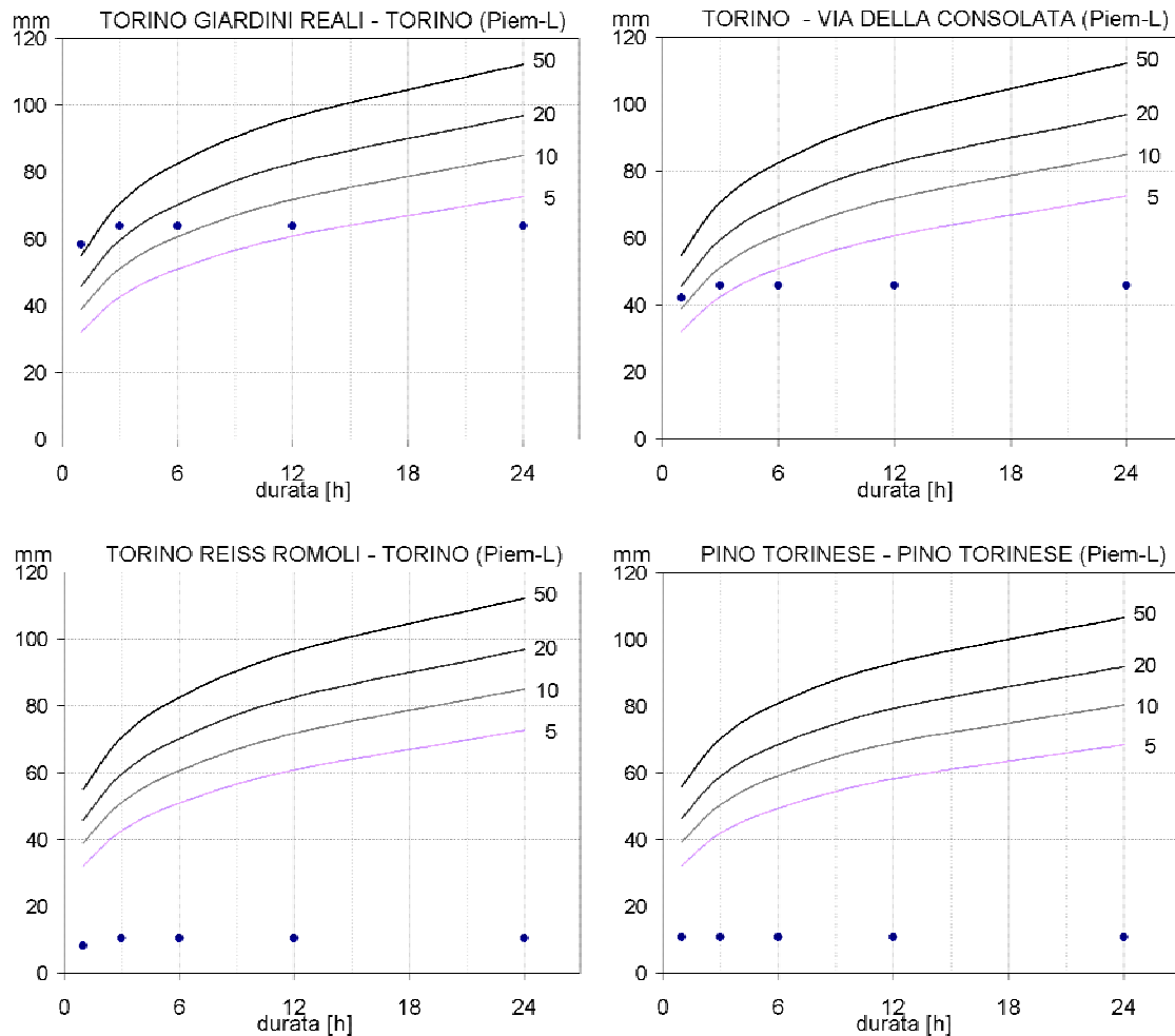
Figura 9. Confronto delle massime altezze di pioggia dell'evento con le curve di possibilità pluviometriche relative ai tempi di ritorno di 5, 10, 20 e 50 anni.
