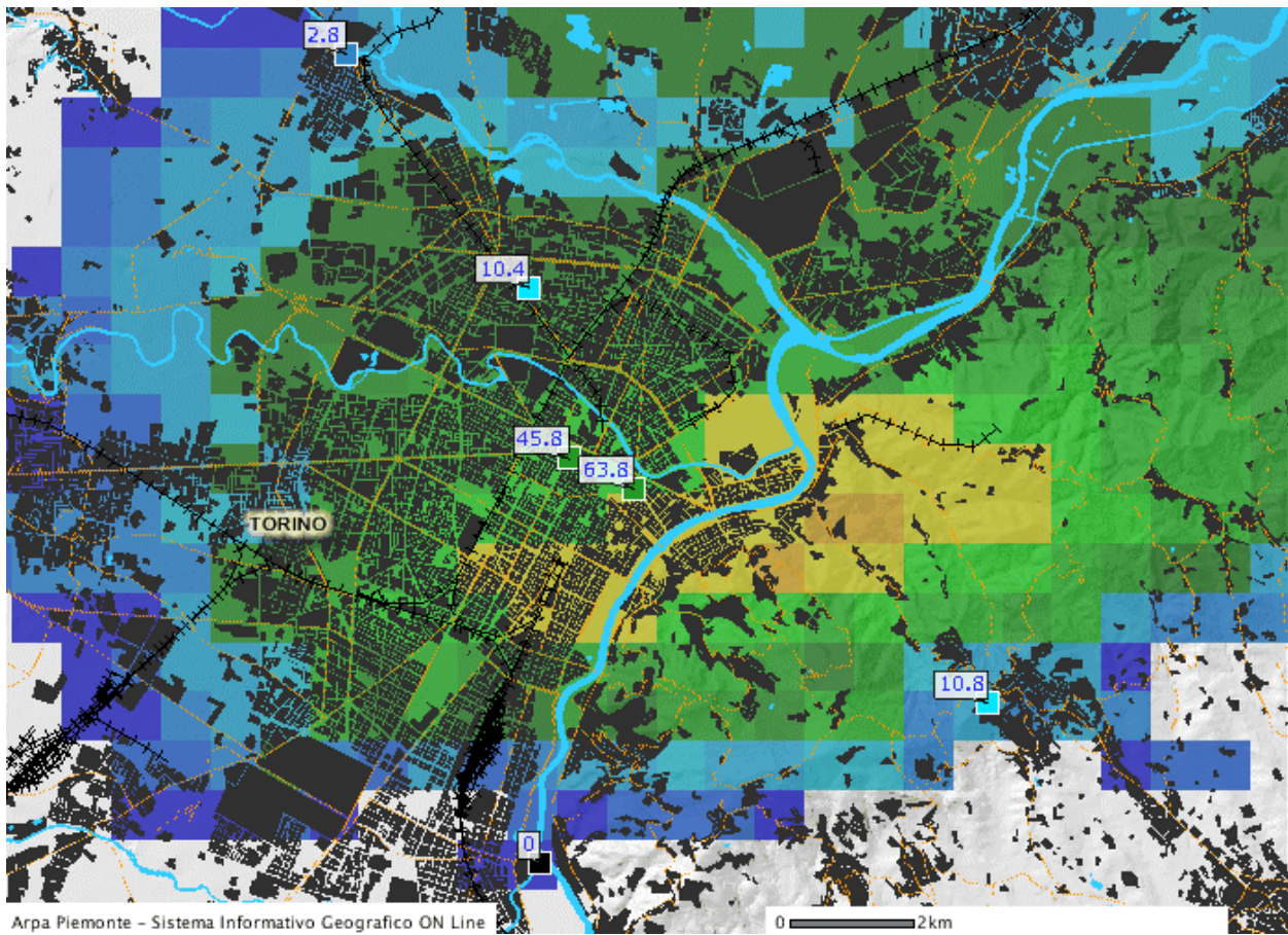
Figura 11. Precipitazione cumulata, stimata da radar di Bric della Croce, tra le 12:00 e le 18:00 UTC. I valori in arancione corrispondono ad una precipitazione compresa tra 90 e 110 mm.
