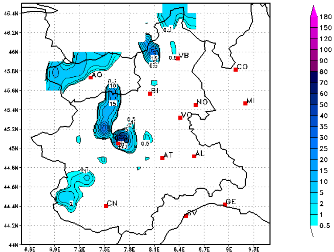
Figura 6: Precipitazione cumulata su 6 ore dall 13 alle 19 UTC del 20/06/2007
