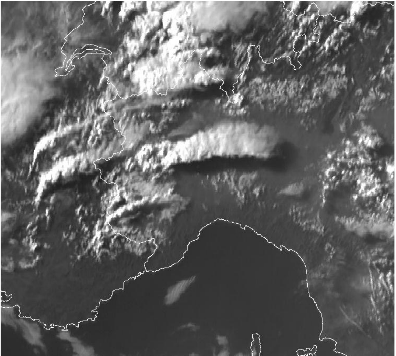
Figura 5: immagine satellitare nel canale del visibile delle 16:45 UTC
