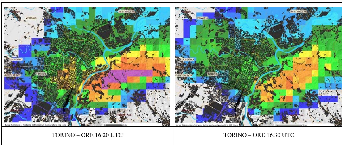
Figura 10. Mappe della precipitazione istantanea su Torino rilevate dal radar meteorologico di Bric della Croce. In arancio sono indicate precipitazioni istantanee comprese tra 40 ed i 70 mm/h, in viola precipitazioni istantanee superiori ai 100 mm/h e presenza di grandine.
