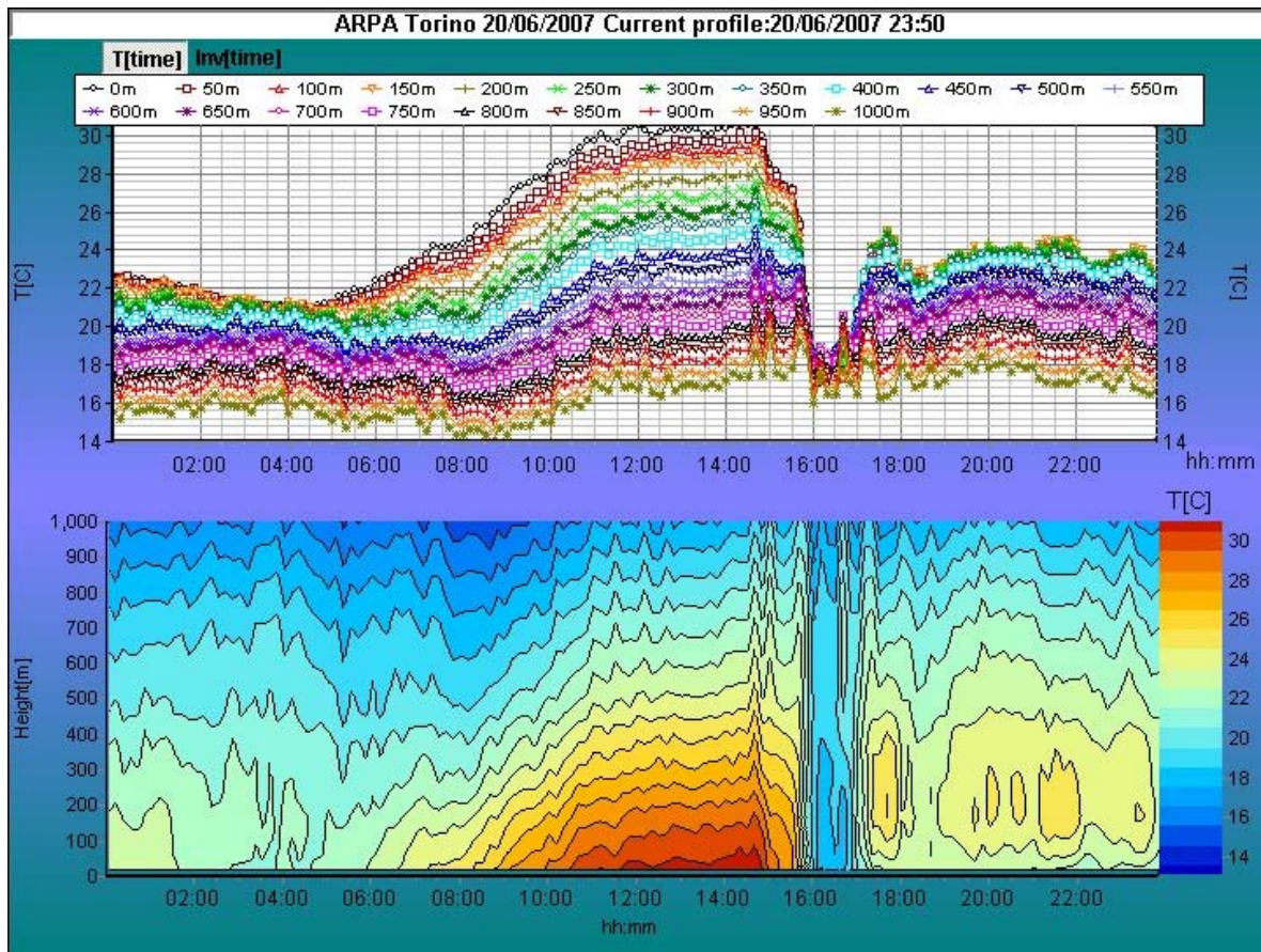
Figura 7: profili verticali di temperatura a Torino il 20/06/2007
