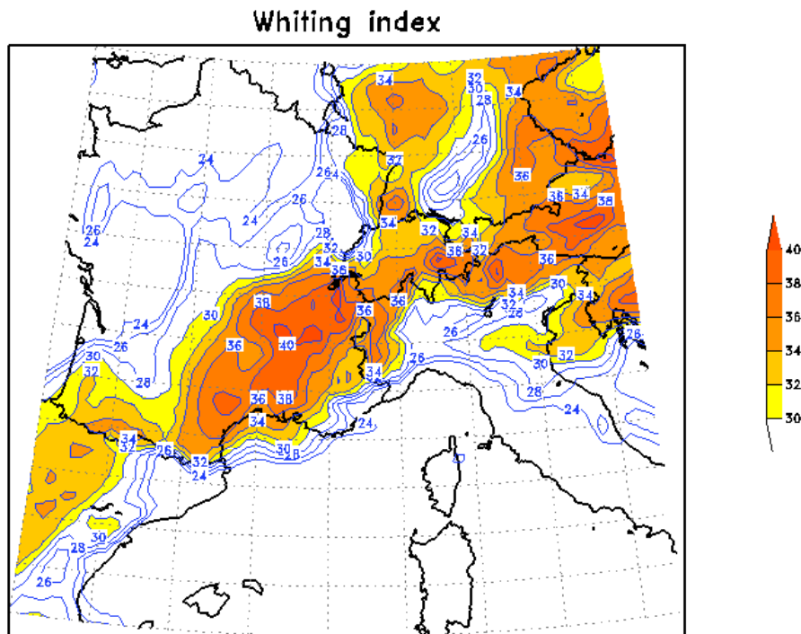
Figura 3: Valori del Whiting Index alle 18 UTC del 20/06/2007
