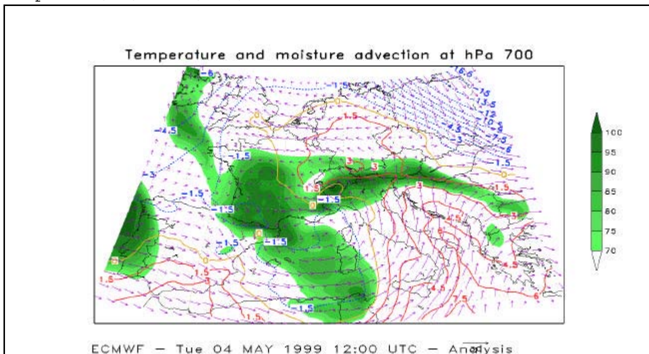
Figura 21: Analisi delle 12 UTC del 4/5/99 dei campi di umidità relativa (livelli di colore), temperatura (linee) e vento (freccette) a 700 hPa
