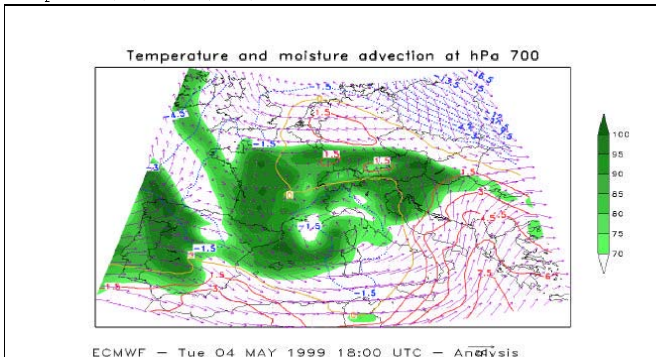
Figura 22: Analisi delle 18 UTC del 4/5/99 dei campi di umidità relativa (livelli di colore), temperatura (linee) e vento (freccette) a 700 hPa
