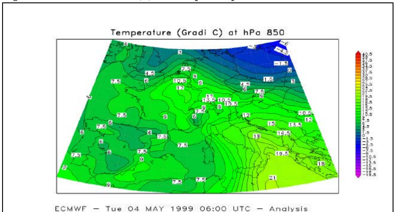
Figura 16 :Analisi delle 6 UTC del 4/5/99 del campo di temperatura a 850 hPa
