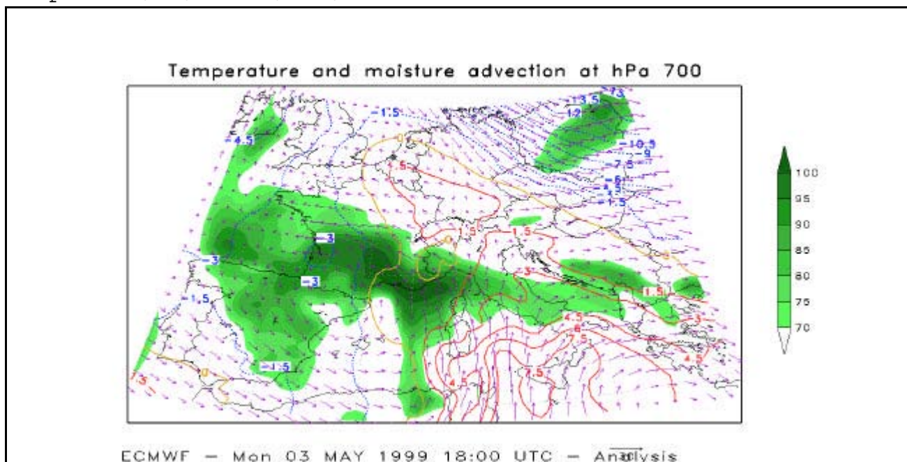
Figura 3: Analisi delle 18 UTC del 3/5/99 dei campi di umidità relativa (livelli di colore), temperatura (linee) e vento (freccette) a 700 hPa
