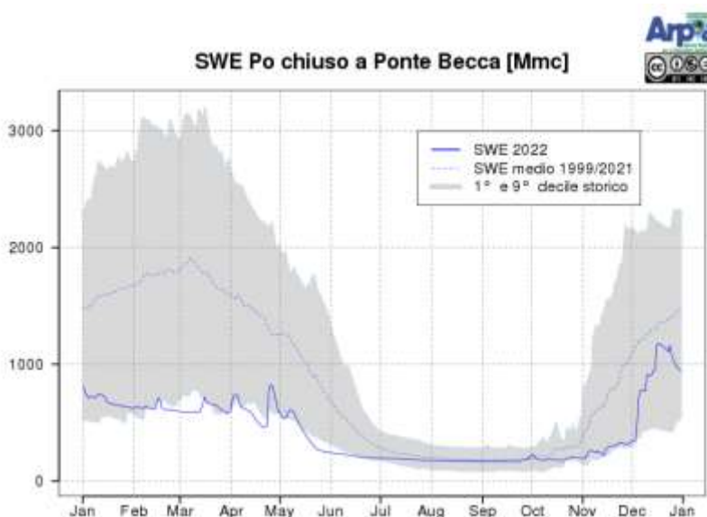
Figura 8. Andamento giornaliero dello SWE nel corso del 2022 e confronto con i dati storici.
