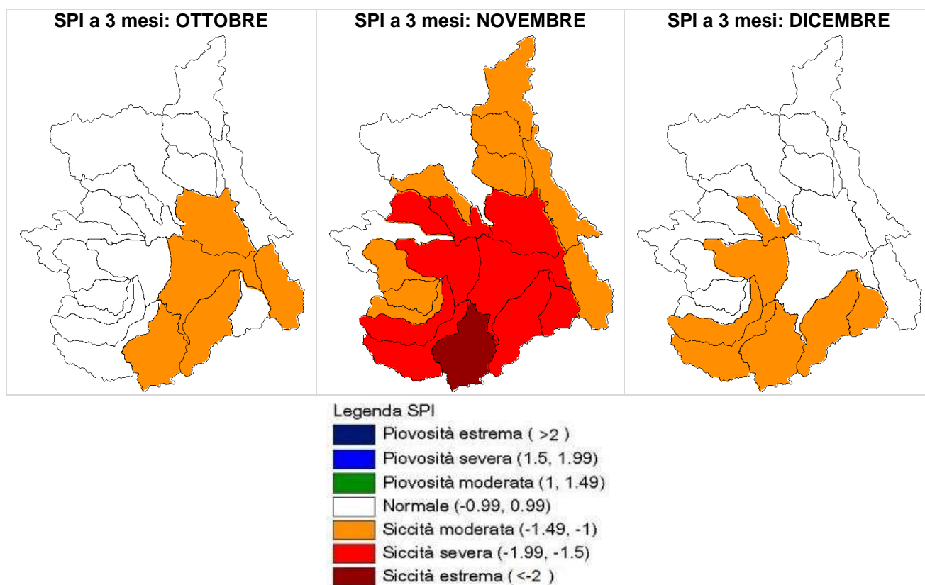
Figura 6. Severità della siccità meteorologica registrata sui bacini idrografici.
