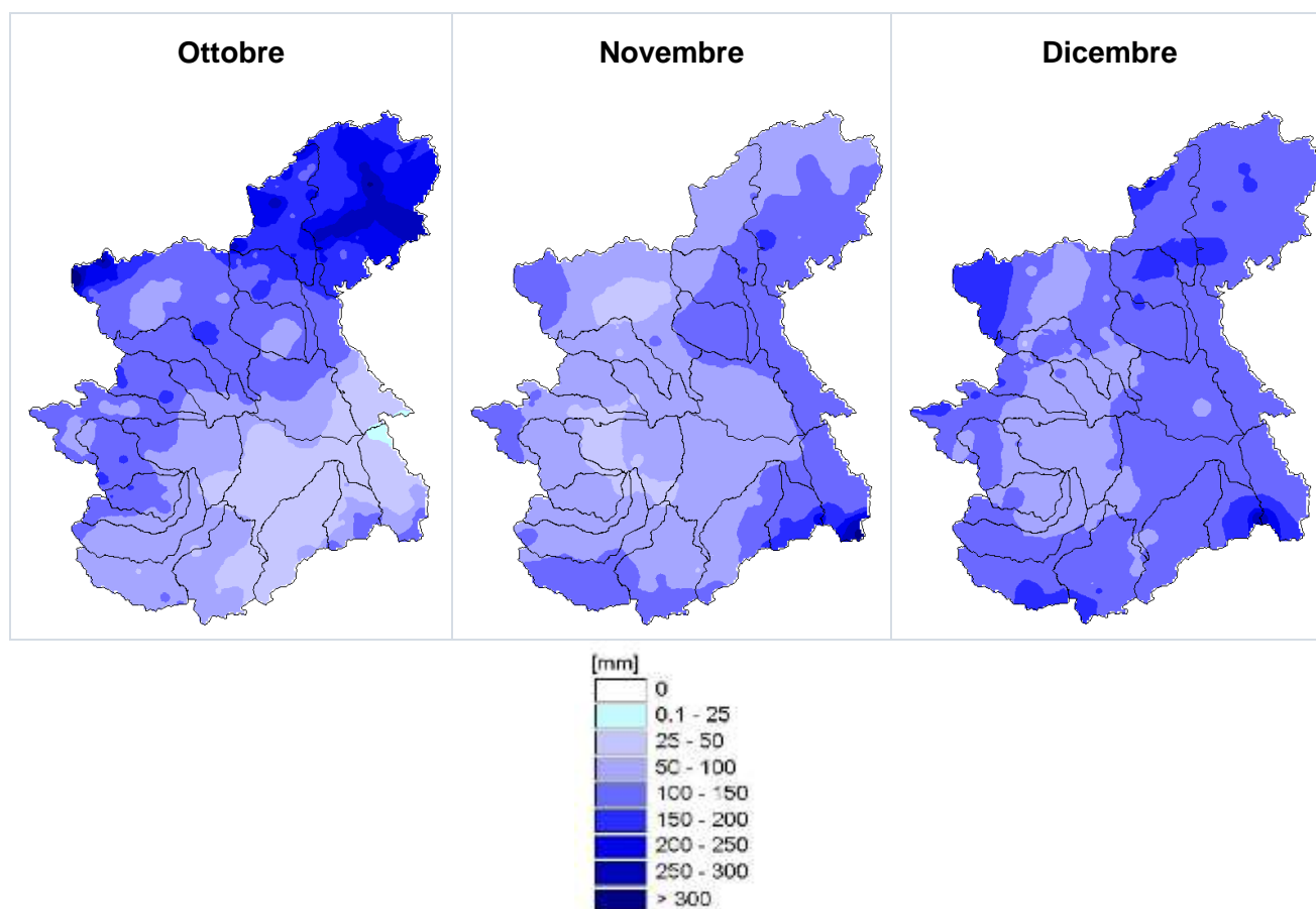
Figura 3. Precipitazioni mensili registrate nel 2022
