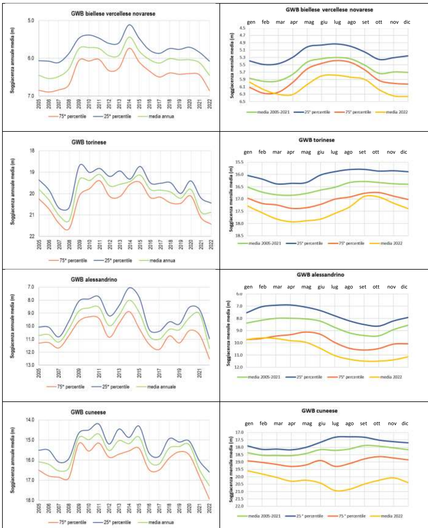
Figura 22 Andamento aggregato per GWB della soggiacenza media annua 2005-2022 (grafici a sinistra) e andamento aggregato per GWB della soggiacenza media mensile del 2022 rapportata a quella della serie 2005-2021 (grafici a destra).
