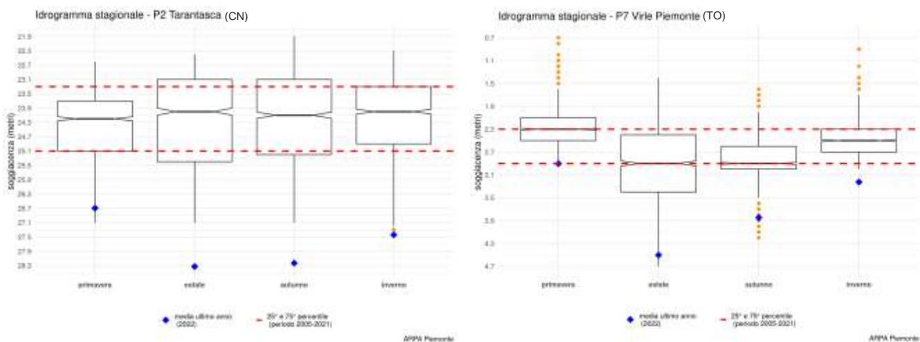
Figura 24 Boxplot delle medie stagionali 2022 in relazione alla serie storica 2005-2021
