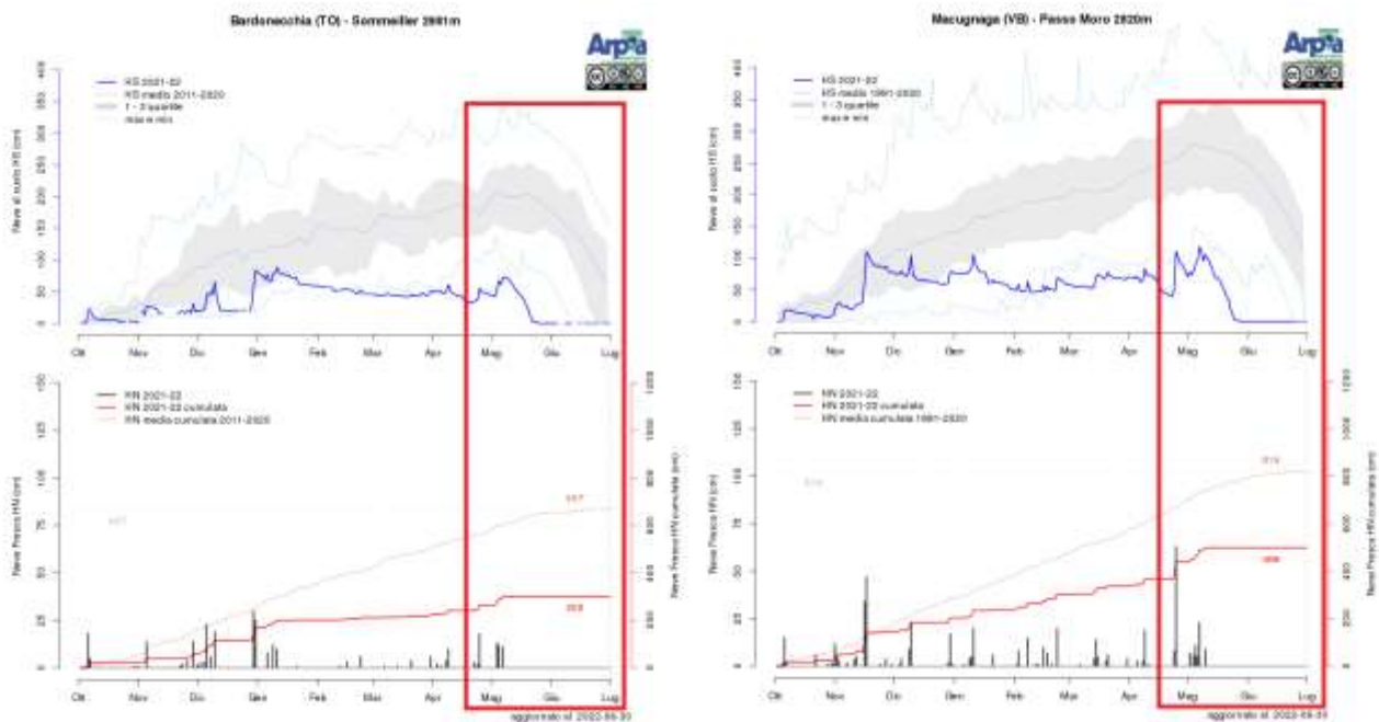
Figura 10: in ordine da sinistra a destra le stazioni nivometriche automatiche del Colle del Sommeiller – Bardonecchia (TO) e Passo del Moro – Macugnaga (VB) per la stagione 2021-2022. In alto l'andamento giornaliero della neve al suolo -HS- dove la linea blu spessa indica l'HS della stagione, la linea tratteggiata indica l'andamento medio dell'HS e l'area colorata in grigio indica +/- la deviazione standard rispetto alla media. In basso le nevicate -HN-: le barre nere indicano i singoli valori di neve fresca giornaliera (asse y di riferimento di sinistra), la linea spessa rossa indica la relativa cumulata, mentre la linea tratteggiata si riferisce alla cumulata media (queste ultime due linee fanno riferimento all'asse y di destra). I numeri riportano rispettivamente il totale di neve fresca della stagione e della media storica (rispettivamente del periodo 2011- 2020 e 1991-2020).
