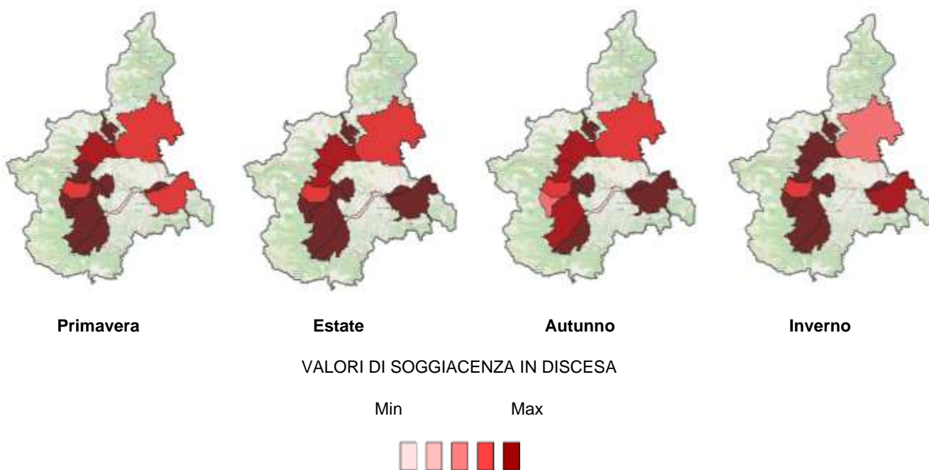
Figura 25 Grado di anomalia della soggiacenza 2022 rispetto alla fascia di fluttuazione dell'anno idrologico medio (serie di riferimento 2005-2021) nelle diverse stagioni.
