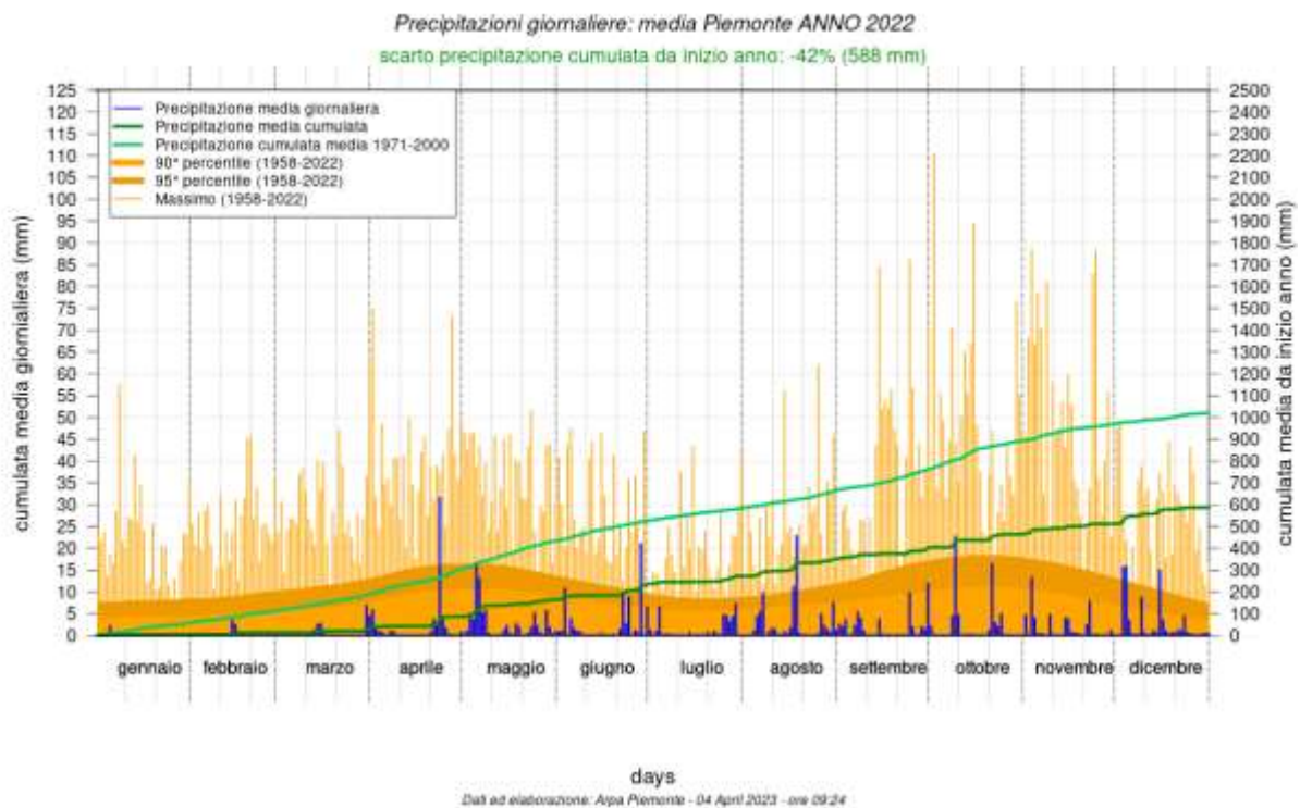
Figura 5. Precipitazione giornaliera registrata da gennaio a dicembre 2022 e confronto con i dati storici dell'ultimo trentennio (clima:1991-2020).
