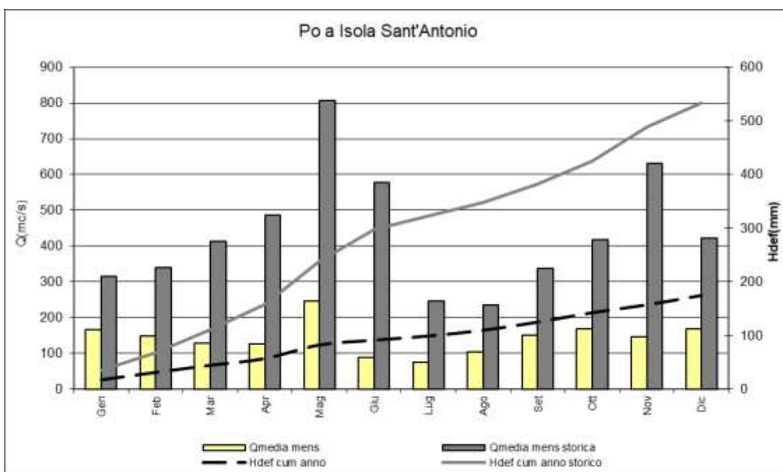
Figura 20. Confronto tra i valori di portata media mensile e deflusso annuo cumulato del 2022 rispetto al periodo storico di riferimento (anni di funzionamento della stazione) per l'idrometro sul Po a Isola Sant'Antonio.
