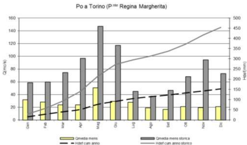
Figura 17. Confronto tra i valori di portata media mensile e deflusso annuo cumulato del 2022 rispetto al periodo storico di riferimento (anni di funzionamento della stazione) per l'idrometro sul Po a Torino.
