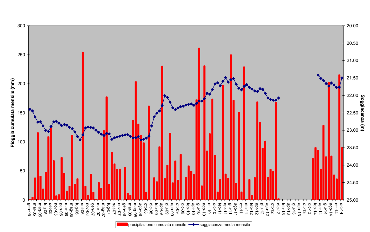
Figura 17. Piogge cumulate mensili e soggiacenza media mensile 2005-2014
