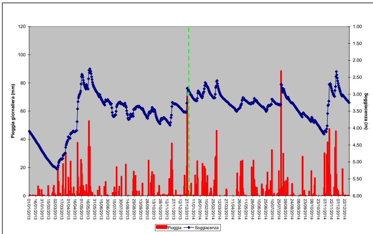
Figura 13. Piogge cumulate giornaliere e soggiacenza media giornaliera 2013-2014
