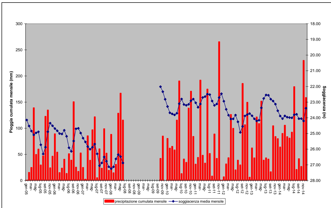
Figura 29. Piogge cumulate mensili e soggiacenza media mensile 2005-2014
