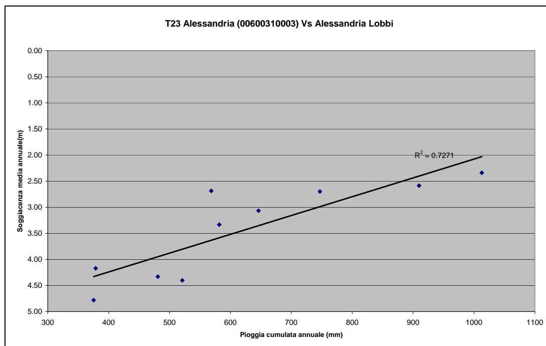
Figura 3. Correlazione tra piogge cumulate/anno e soggiacenza media/anno (2005-2014)
