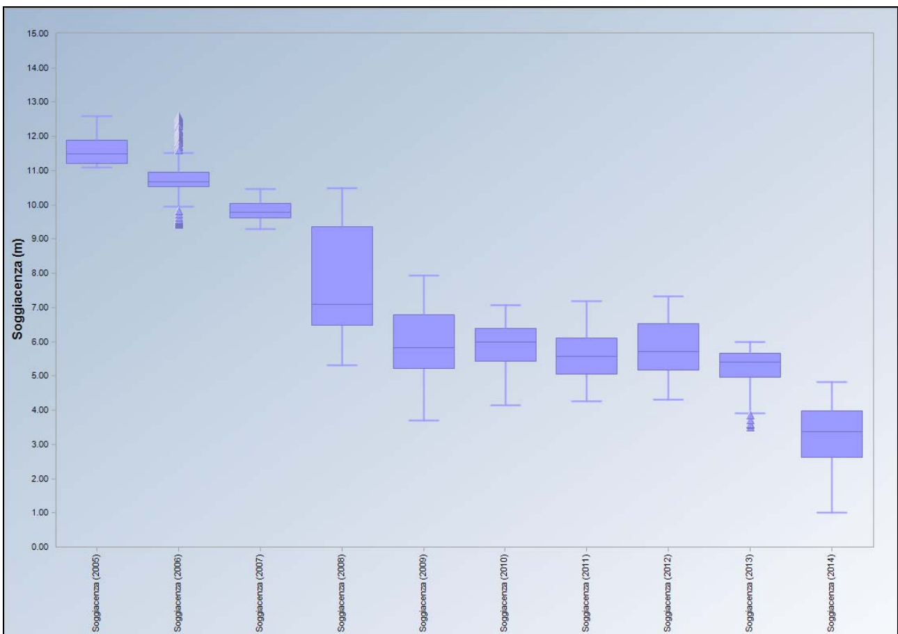
Figura 6. Box-plot soggiacenza media giornaliera 2005-2014
