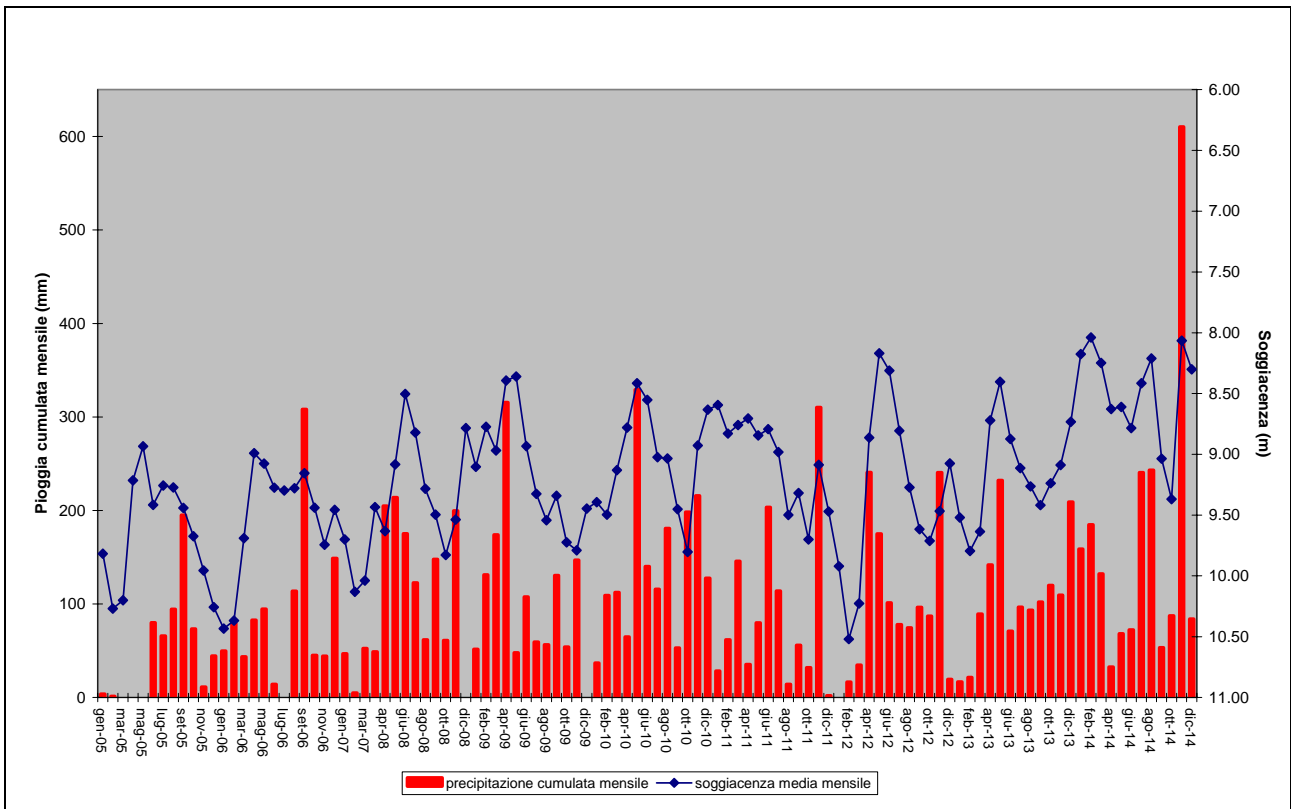
Figura 8. Piogge cumulate mensili e soggiacenza media mensile 2005-2014
