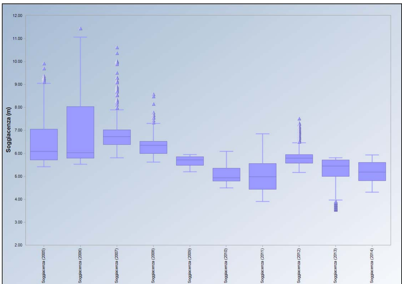
Figura 27. Box-plot soggiacenza media giornaliera 2005-2014
