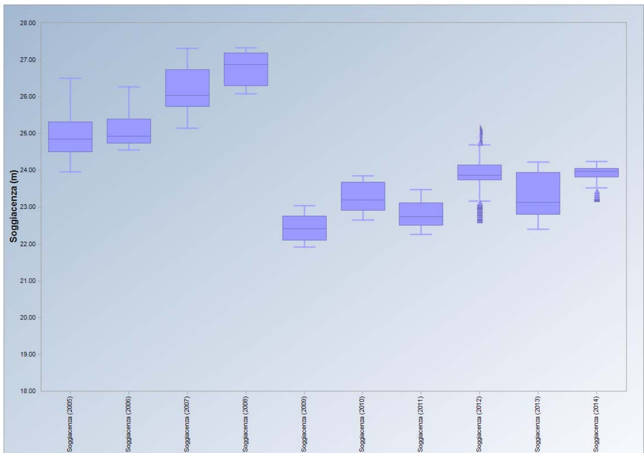
Figura 30. Box-plot soggiacenza media giornaliera 2005-2014
