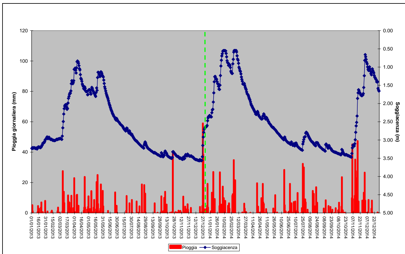
Figura 40. Piogge cumulate giornaliere e soggiacenza media giornaliera 2013-2014
