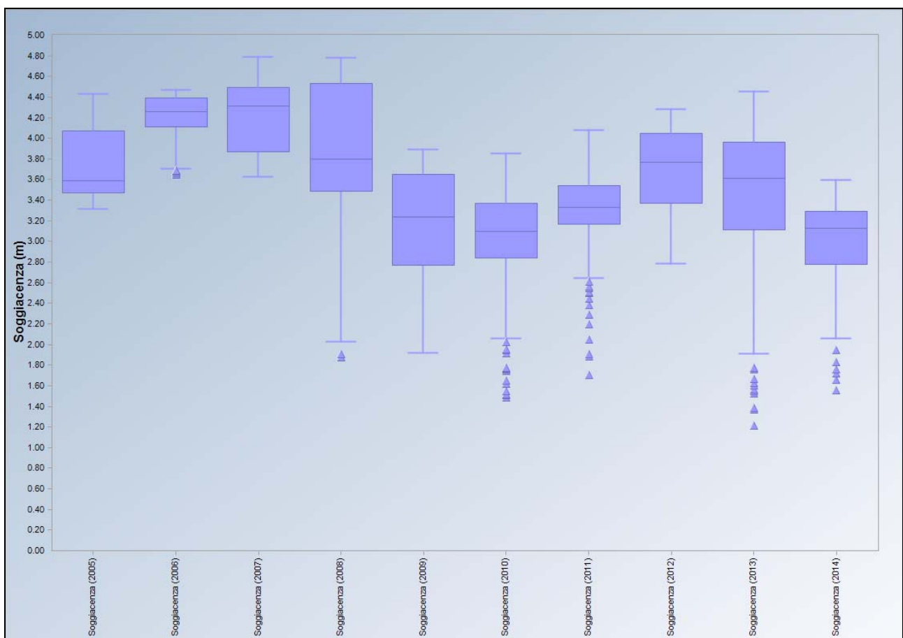
Figura 12. Box-plot soggiacenza media giornaliera 2005-2014
