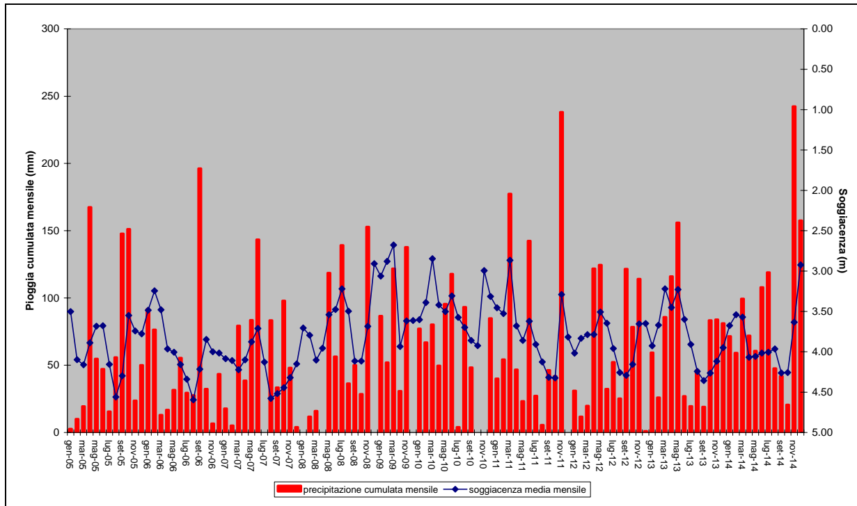
Figura 32. Piogge cumulate mensili e soggiacenza media mensile 2005-2014
