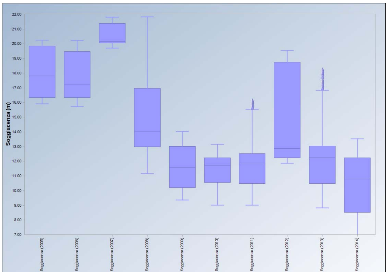
Figura 36. Box-plot soggiacenza media giornaliera 2005-2014
