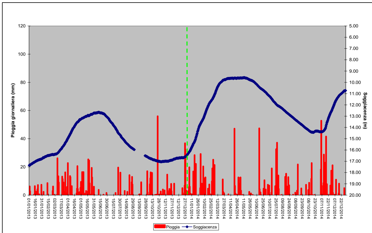
Figura 37. Piogge cumulate giornaliere e soggiacenza media giornaliera 2013-2014
