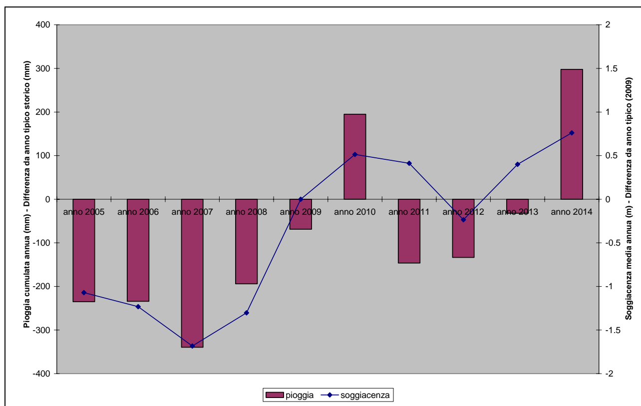
Figura 46. Scostamenti pioggia annua cumulata e soggiacenza media annua rispetto ai valori tipici del 2009
