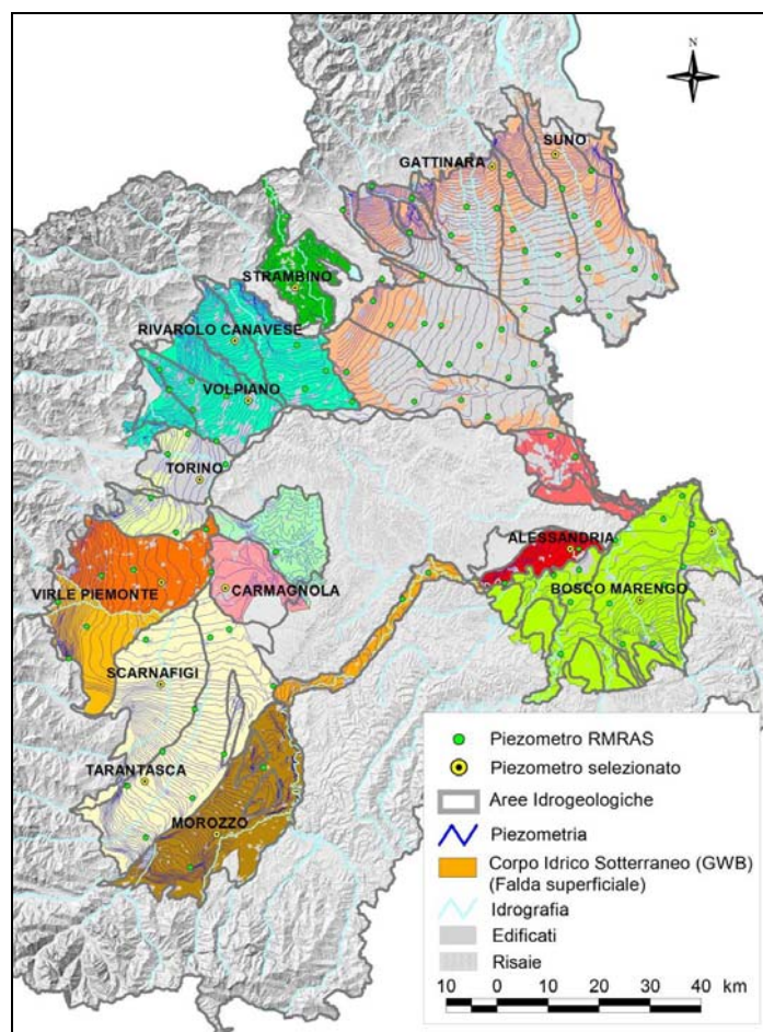
Figura 1. Ubicazione dei piezometri strumentati e identificazione di quelli selezionati ai fini dello studio, nella RMRAS
