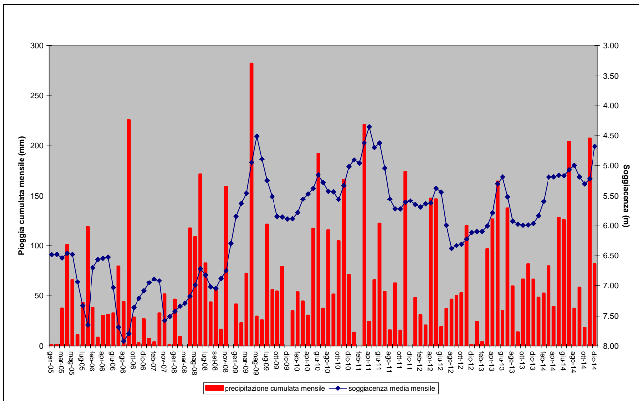
Figura 23. Piogge cumulate mensili e soggiacenza media mensile 2005-2014
