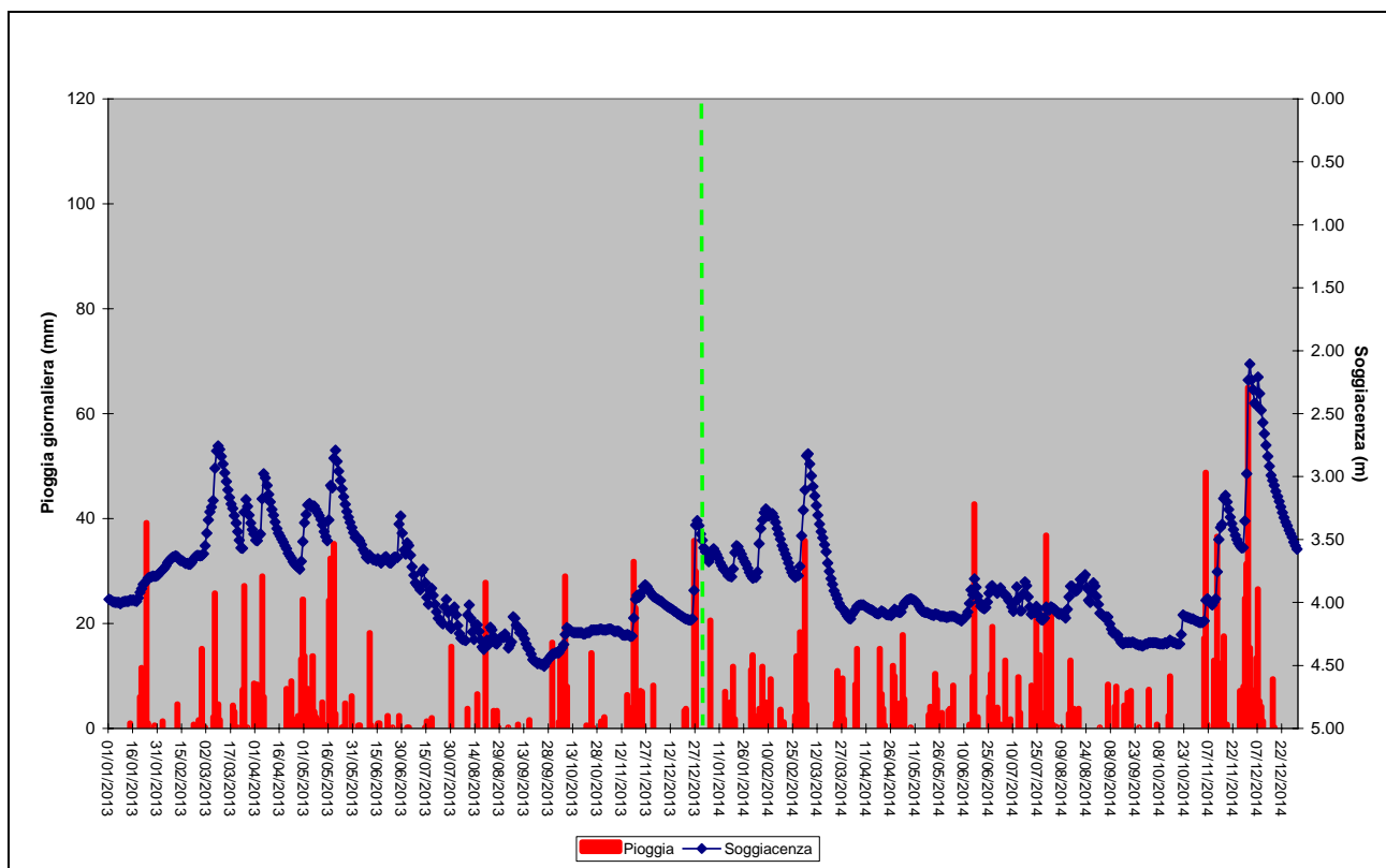
Figura 31. Piogge cumulate giornaliere e soggiacenza media giornaliera 2013-2014
