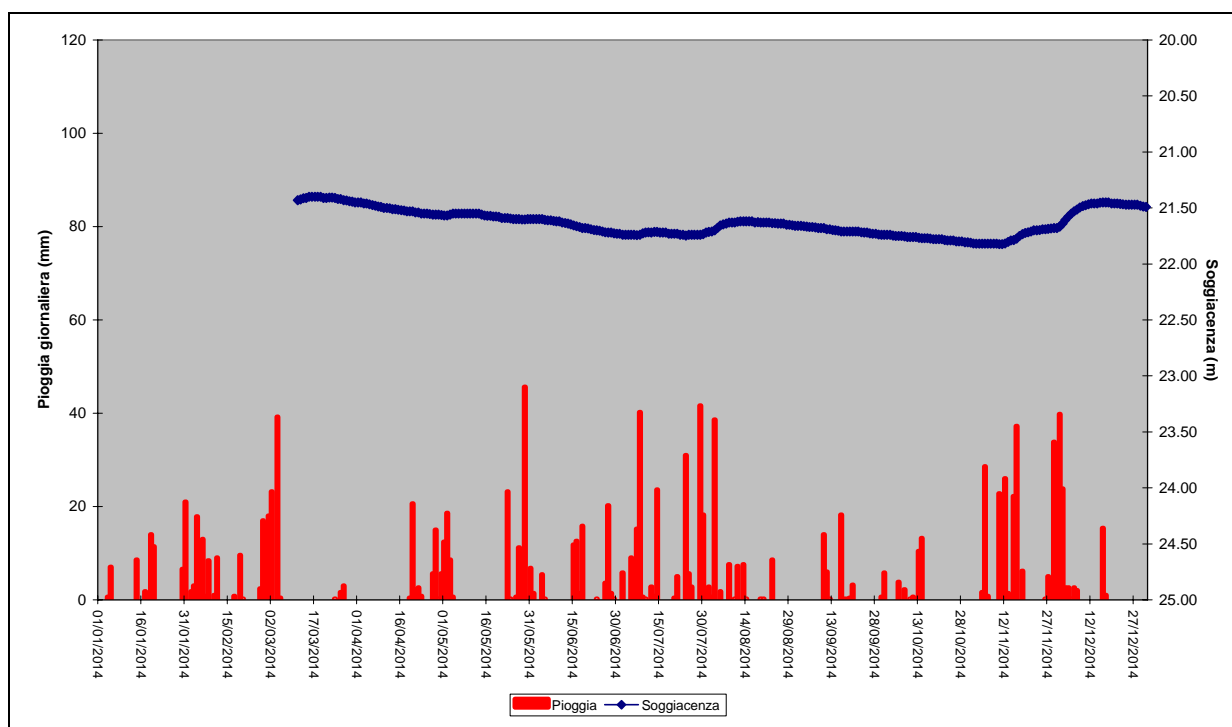
Figura 16. Piogge cumulate giornaliere e soggiacenza media giornaliera 2014
