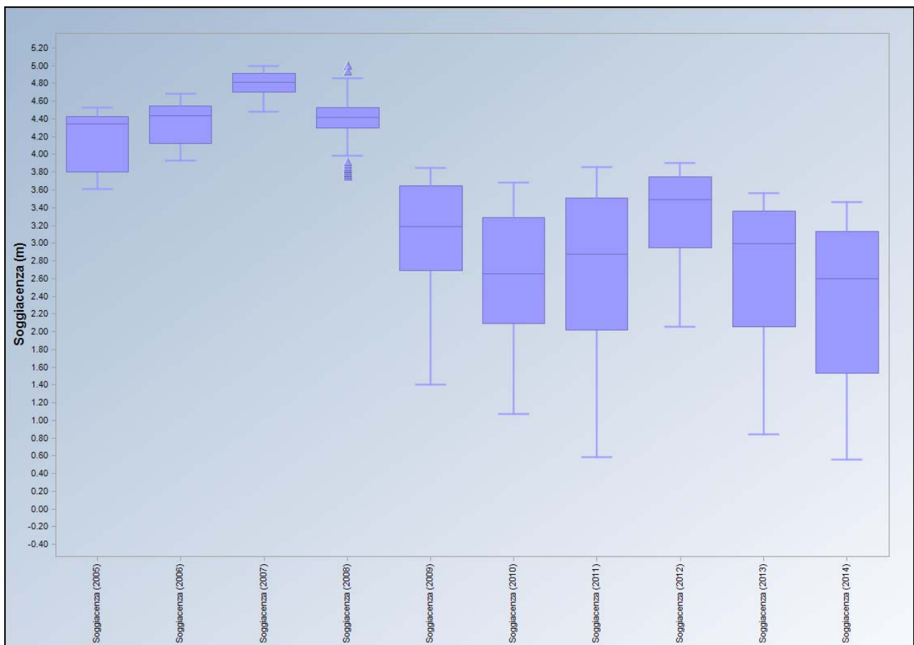
Figura 42. Box-plot soggiacenza media giornaliera 2005-2014
