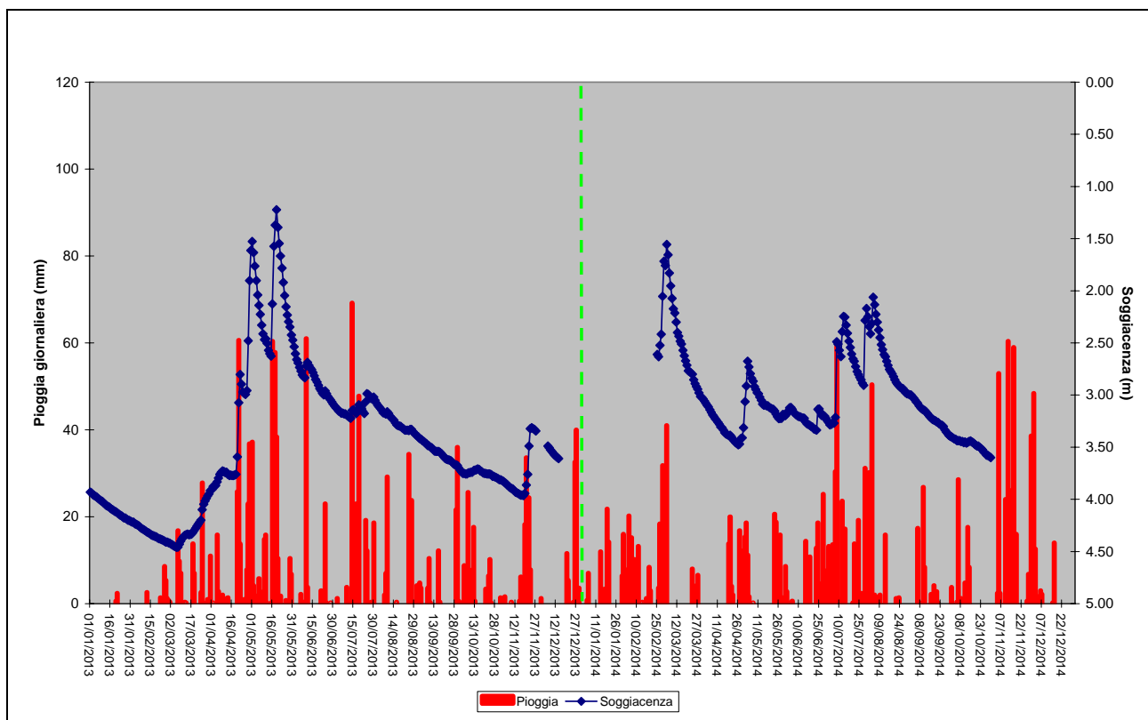
Figura 10. Piogge cumulate giornaliere e soggiacenza media giornaliera 2013-2014
