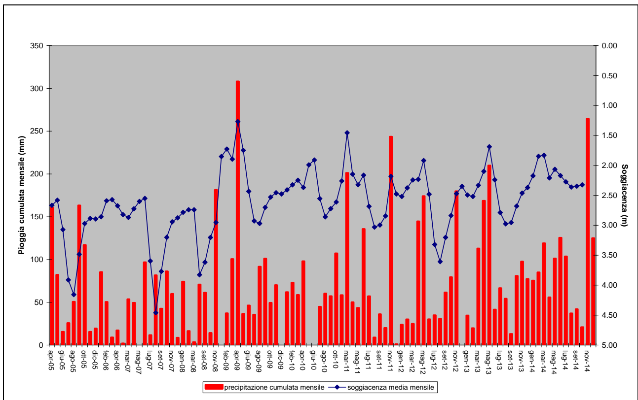
Figura 20. Piogge cumulate mensili e soggiacenza media mensile 2005-2014
