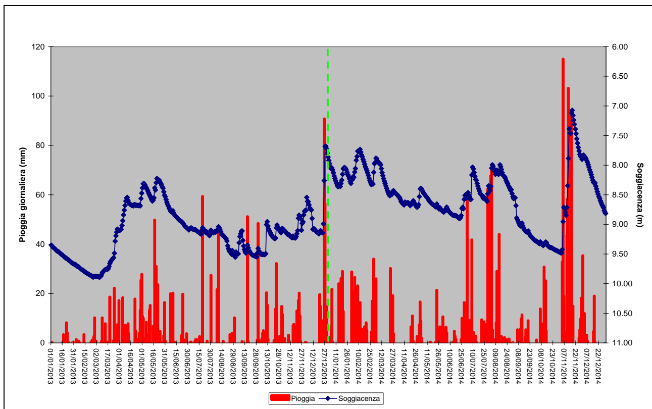
Figura 7. Piogge cumulate giornaliere e soggiacenza media giornaliera 2013-2014
