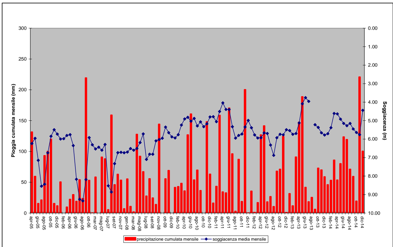
Figura 26. Piogge cumulate mensili e soggiacenza media mensile 2005-2014
