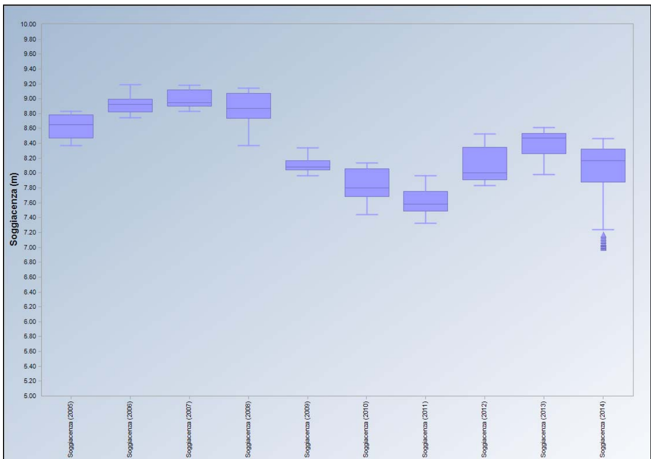
Figura 45. Box-plot soggiacenza media giornaliera 2005-2014
