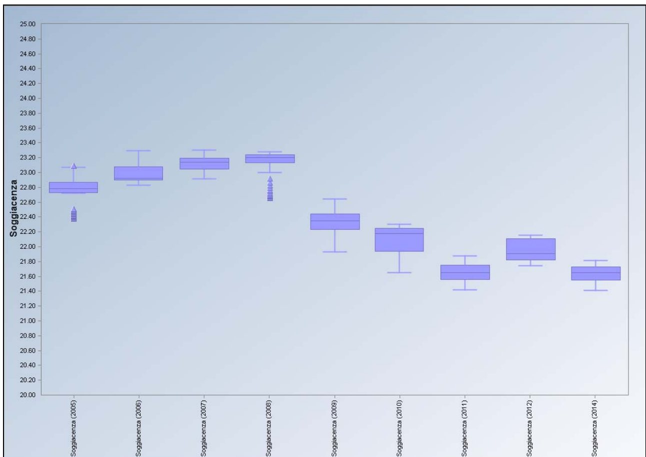
Figura 18. Box-plot soggiacenza media giornaliera 2005-2014
