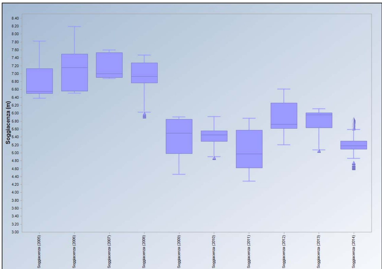
Figura 24. Box-plot soggiacenza media giornaliera 2005-2014
