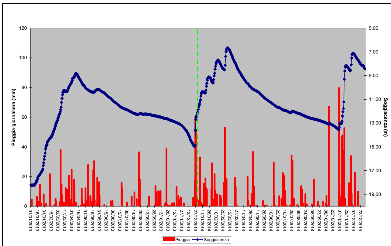
Figura 34. Piogge cumulate giornaliere e soggiacenza media giornaliera 2013-2014
