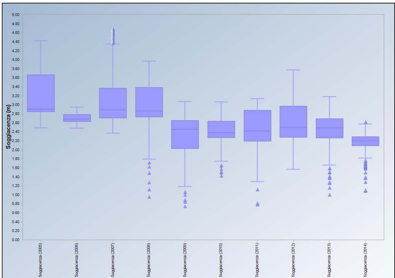
Figura 21. Box-plot soggiacenza media giornaliera 2005-2014
