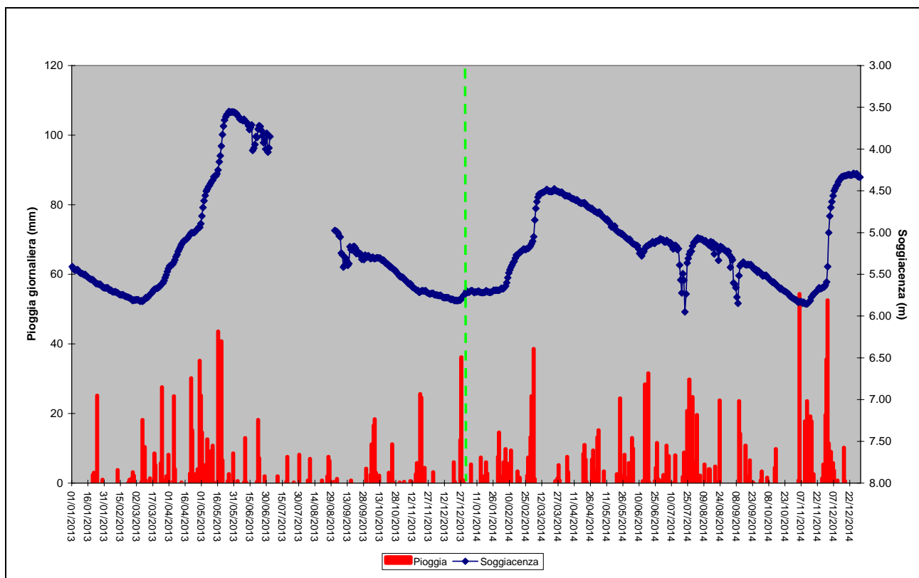
Figura 25. Piogge cumulate giornaliere e soggiacenza media giornaliera 2013-2014
