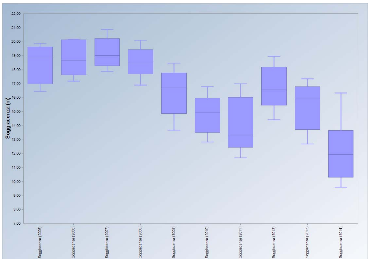
Figura 39. Box-plot soggiacenza media giornaliera 2005-2014
