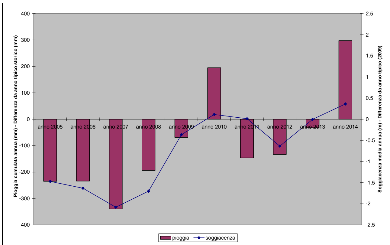
Figura 7. Scostamenti pioggia annua cumulata e soggiacenza media annua rispetto ai valori tipici del 2013
