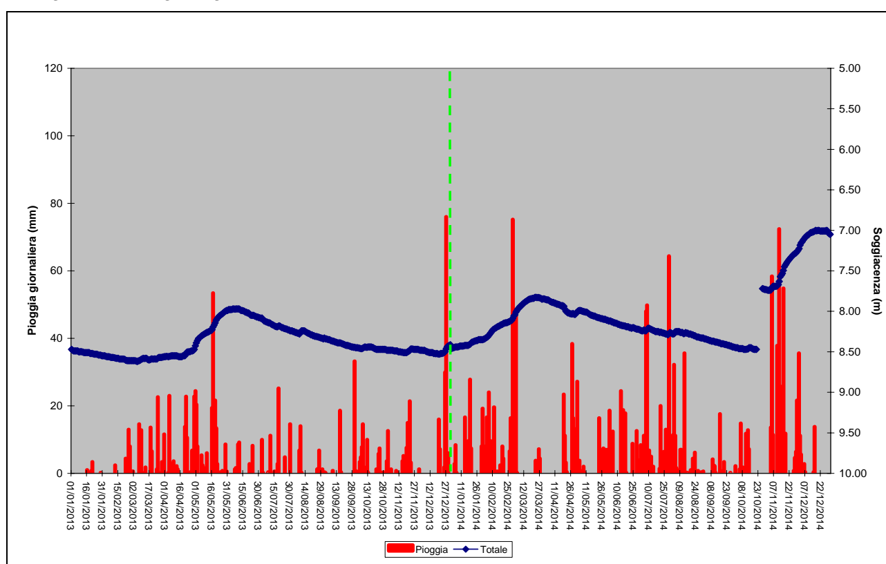
Figura 43. Piogge cumulate giornaliere e soggiacenza media giornaliera 2013-2014
