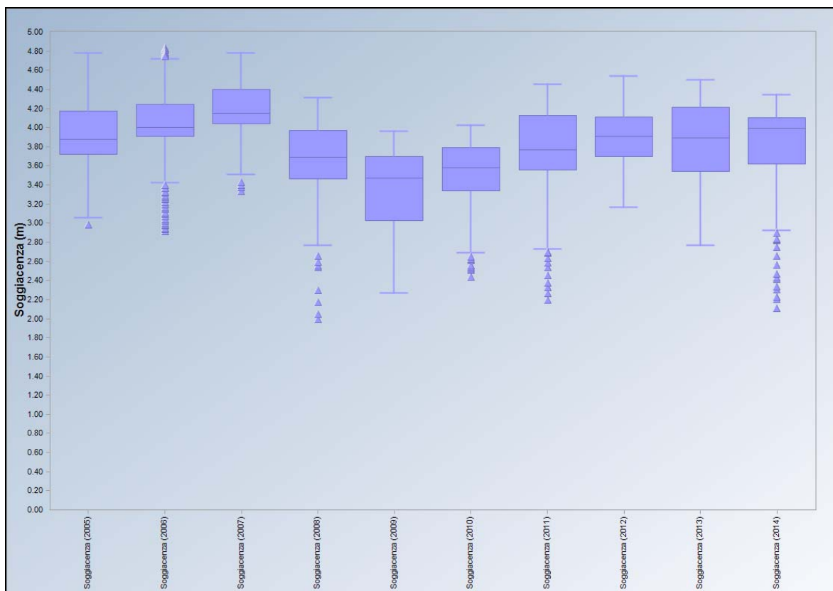
Figura 33. Box-plot soggiacenza media giornaliera 2005-2014
