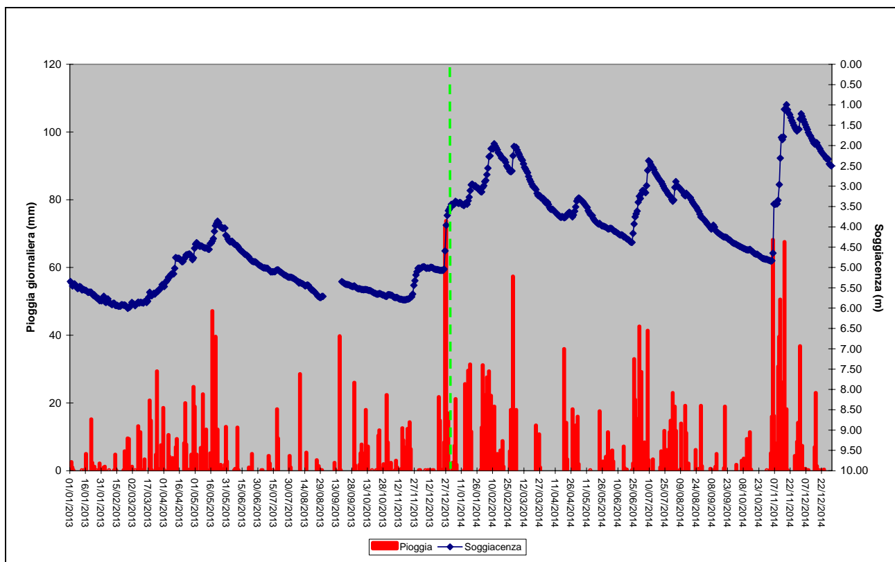
Figura 4. Piogge cumulate giornaliere e soggiacenza media giornaliera 2013-2014
