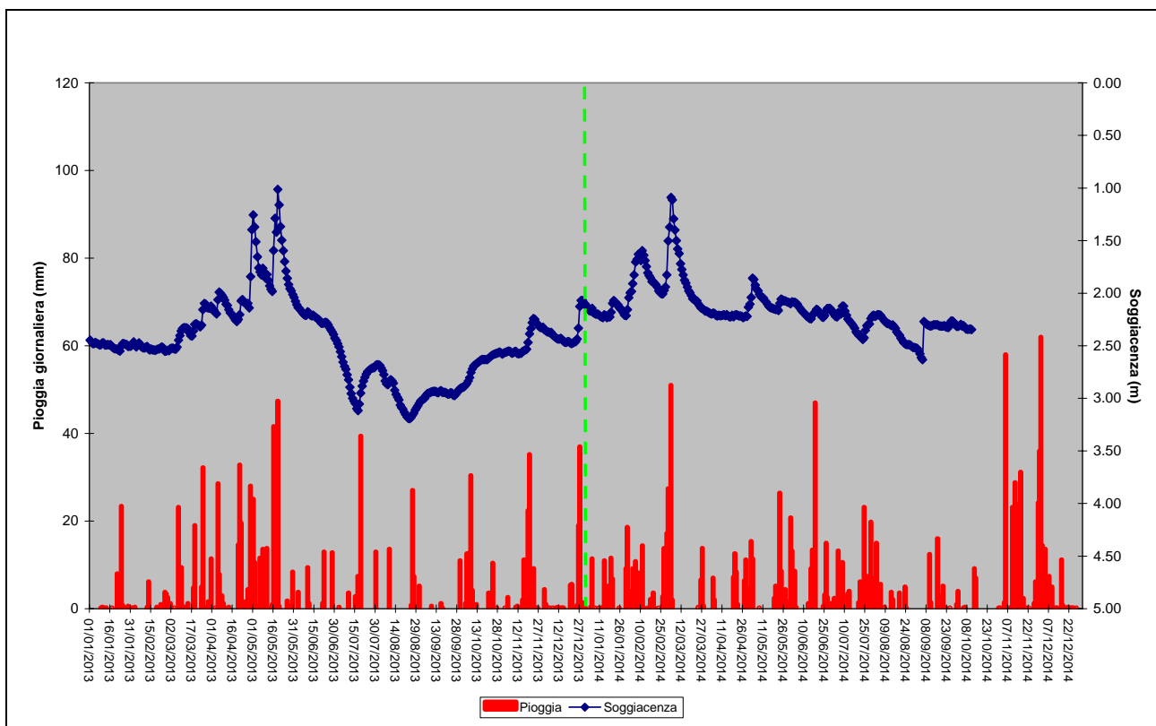
Figura 19. Piogge cumulate giornaliere e soggiacenza media giornaliera 2013-2014
