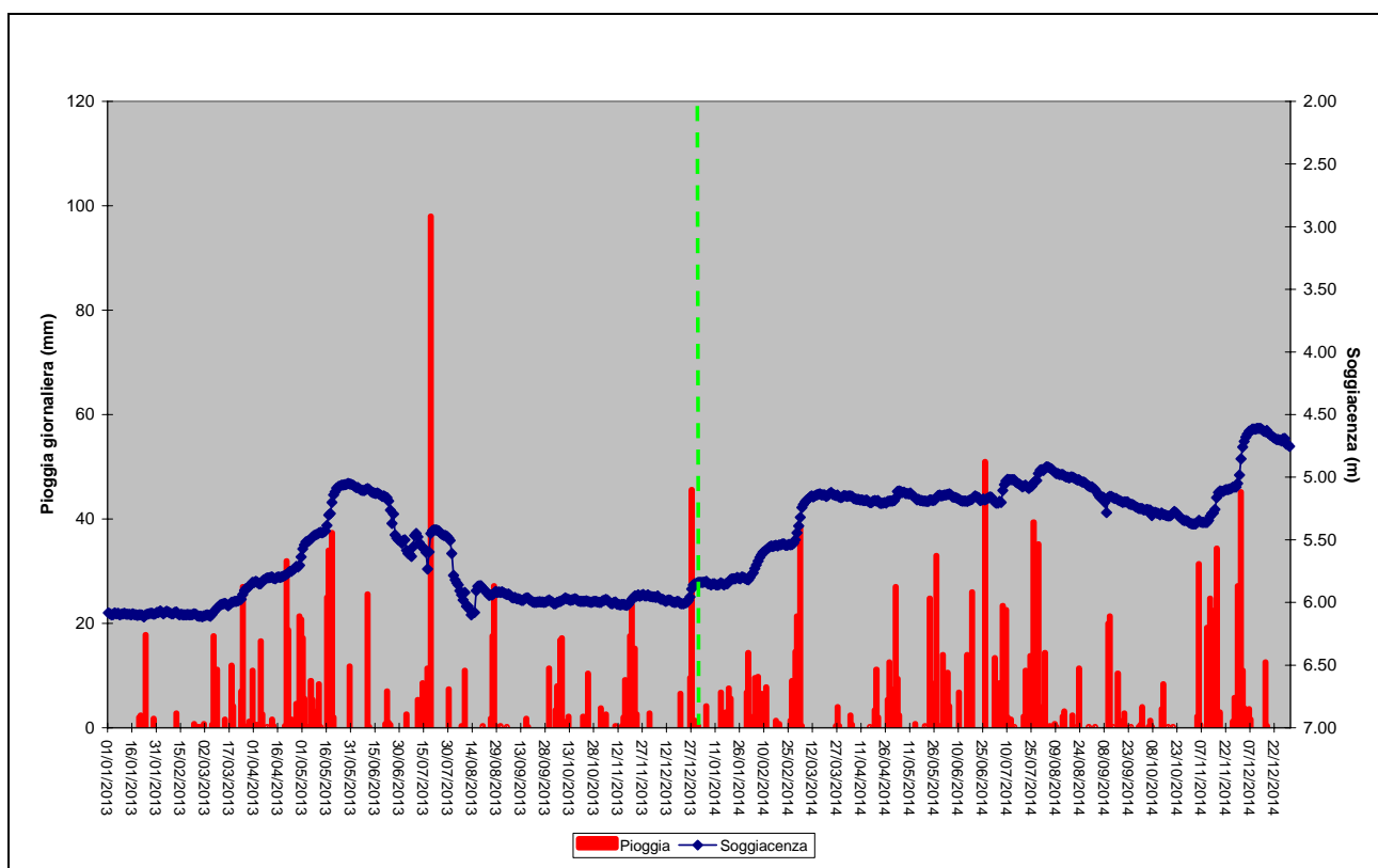
Figura 22. Piogge cumulate giornaliere e soggiacenza media giornaliera 2013-2014
