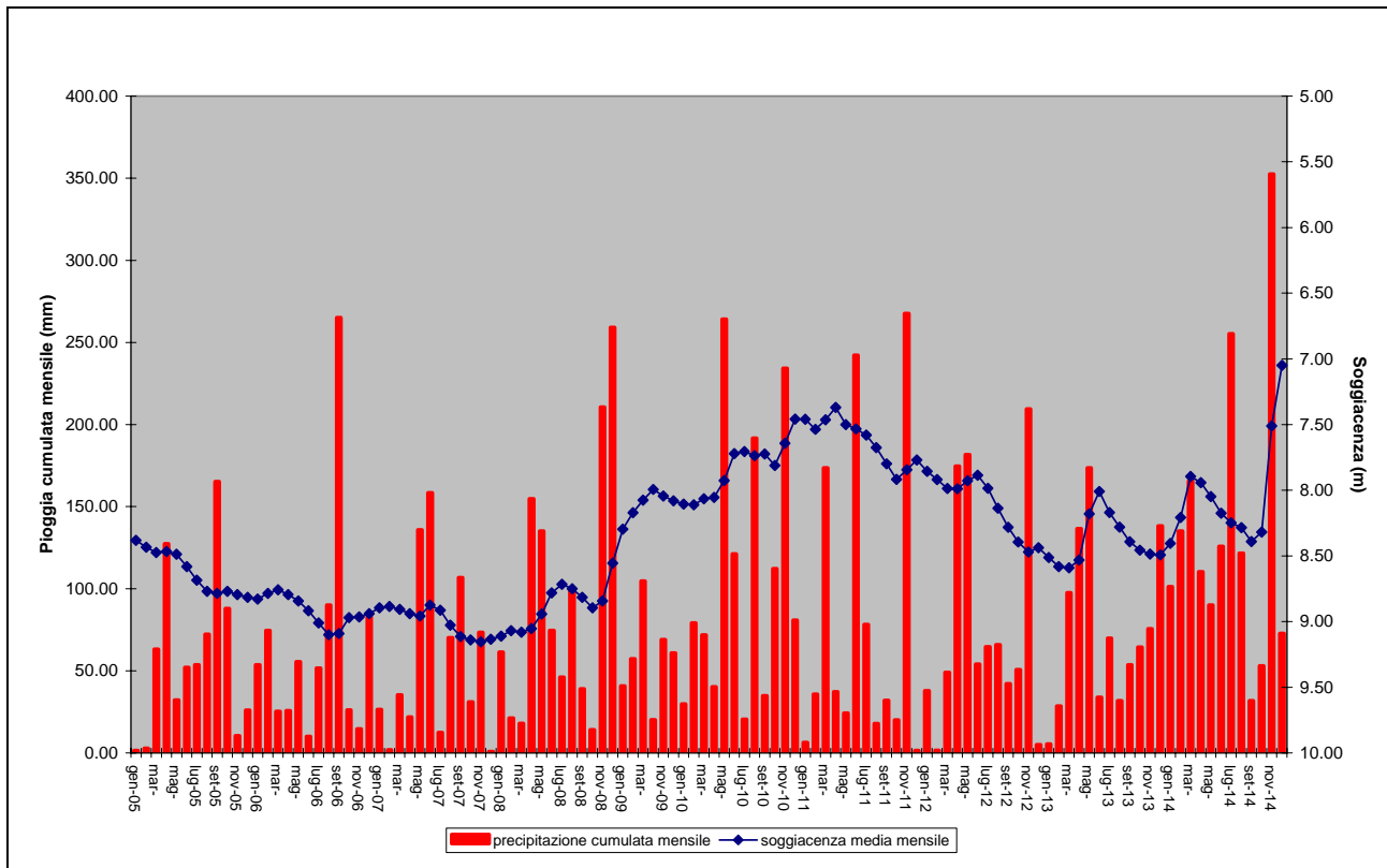
Figura 44. Piogge cumulate mensili e soggiacenza media mensile 2005-2014
