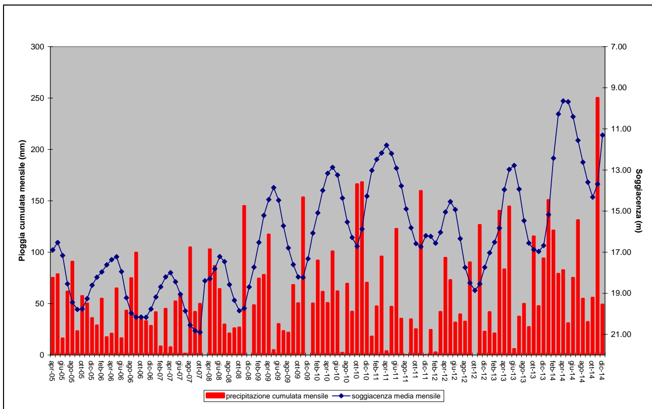
Figura 38. Piogge cumulate mensili e soggiacenza media mensile 2005-2014
