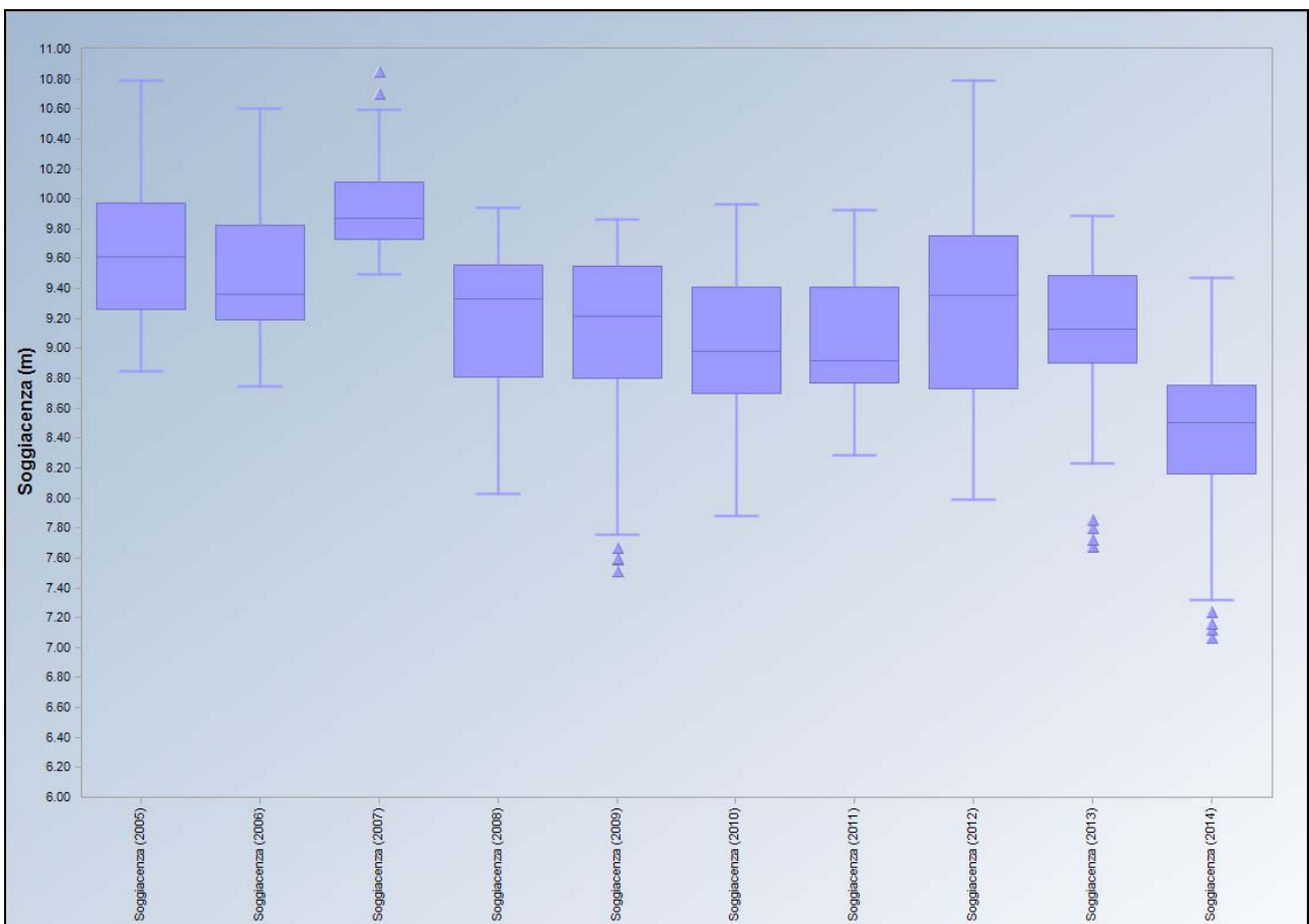
Figura 9. Box-plot soggiacenza media giornaliera 2005-2014
