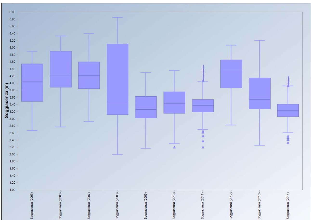
Figura 15. Box-plot soggiacenza media giornaliera 2005-2014
