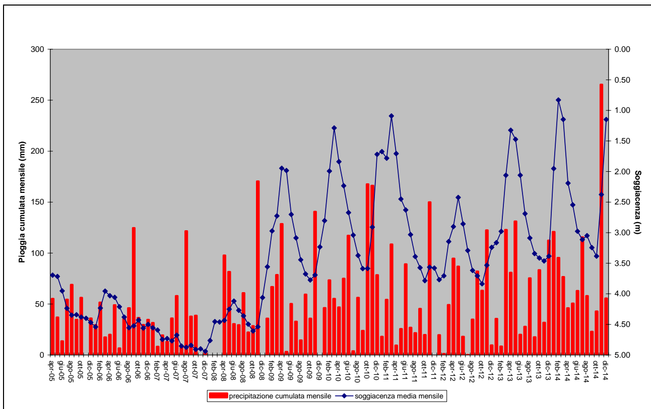
Figura 41. Pioggie cumulate mensili e soggiacenza media mensile 2005-2014
