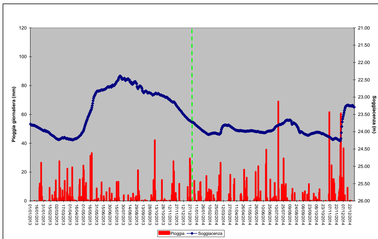
Figura 28. Pioggie cumulate giornaliere e soggiacenza media giornaliera 2013-2014
