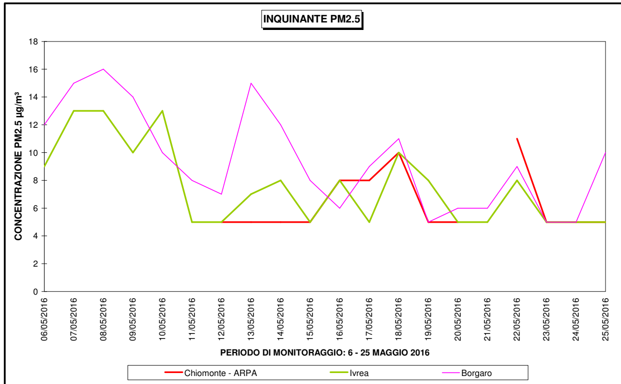
Figura 26 – Particolato sospeso PM 2.5
