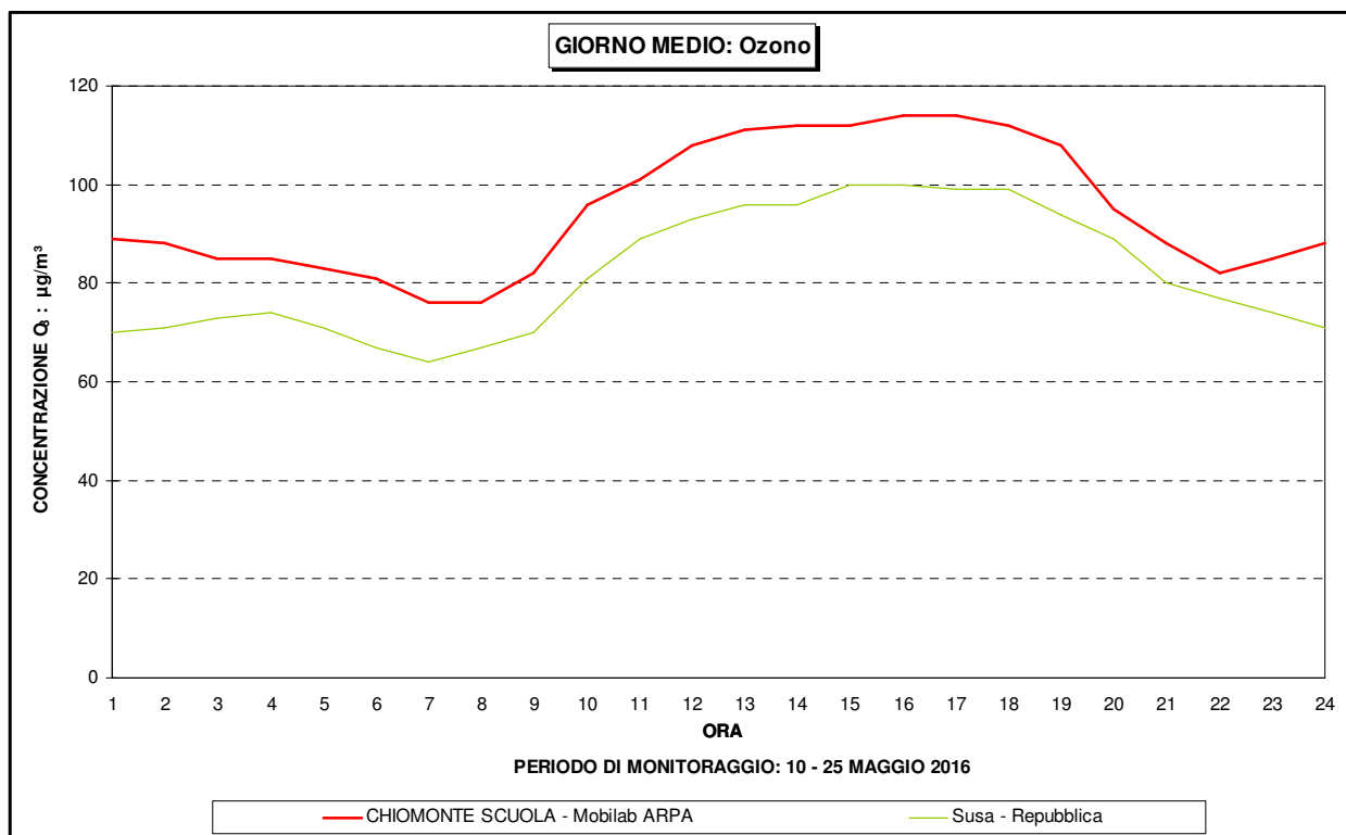
Figura 28 – O 3 : andamento del giorno medio
