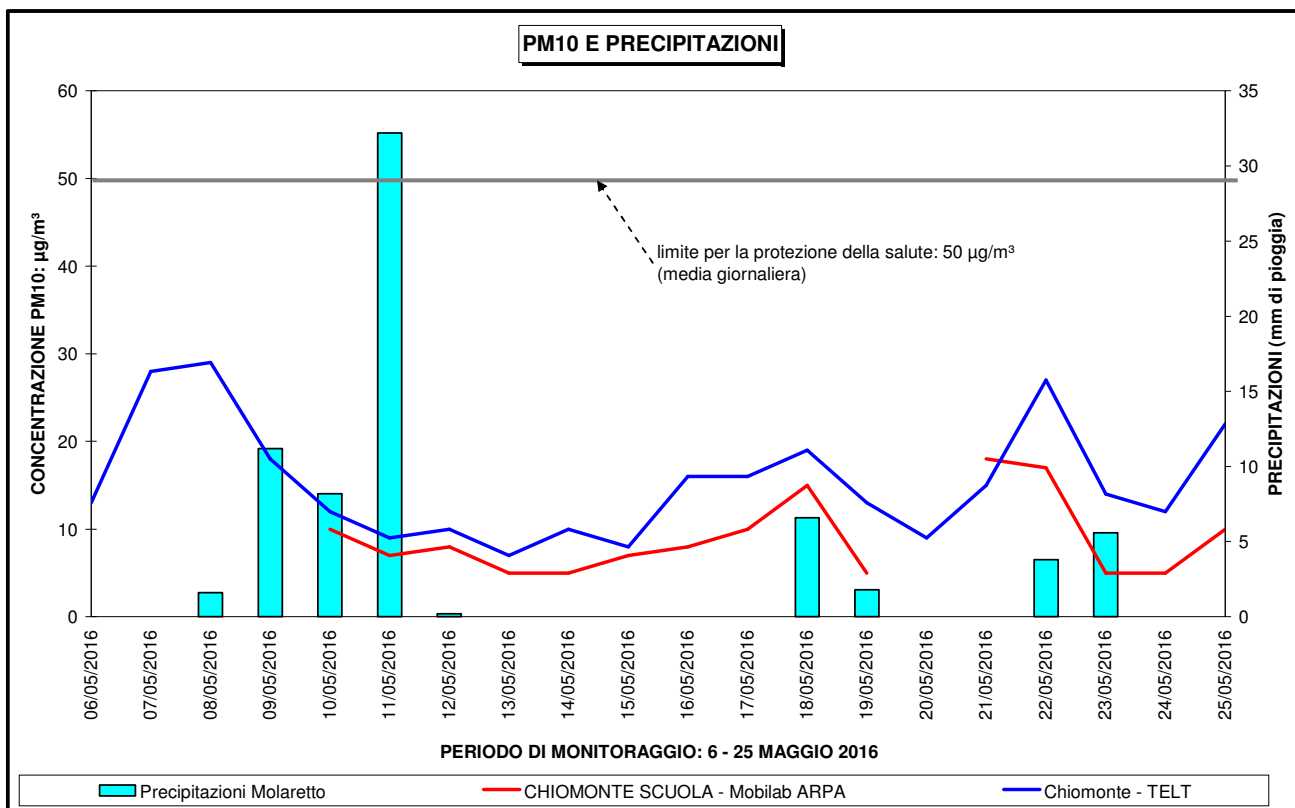
Figura 25 – Particolato sospeso PM 10 confronto con le precipitazioni
