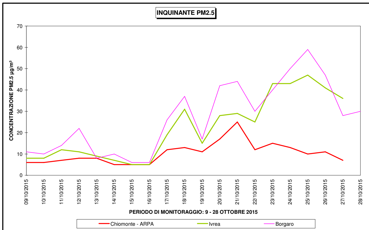
Figura 26 – Particolato sospeso PM 2,5
