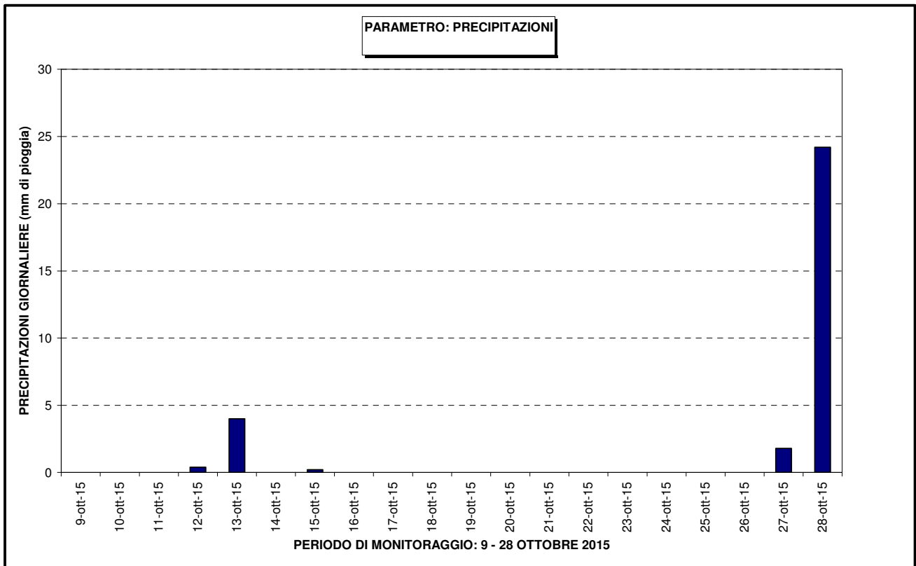
Figura 13- Precipitazioni nel corso della campagna di monitoraggio
