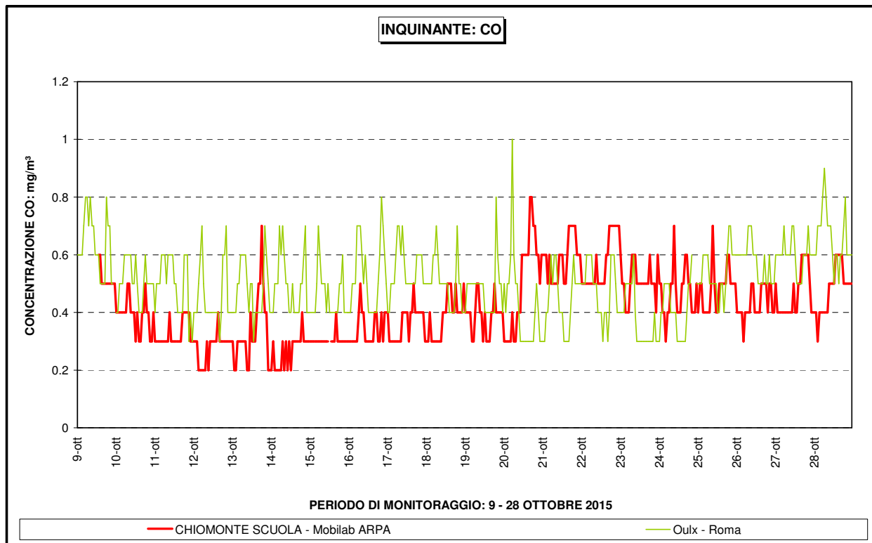
Figura 16 – CO: andamento della concentrazione oraria nel corso della campagna di monitoraggio
