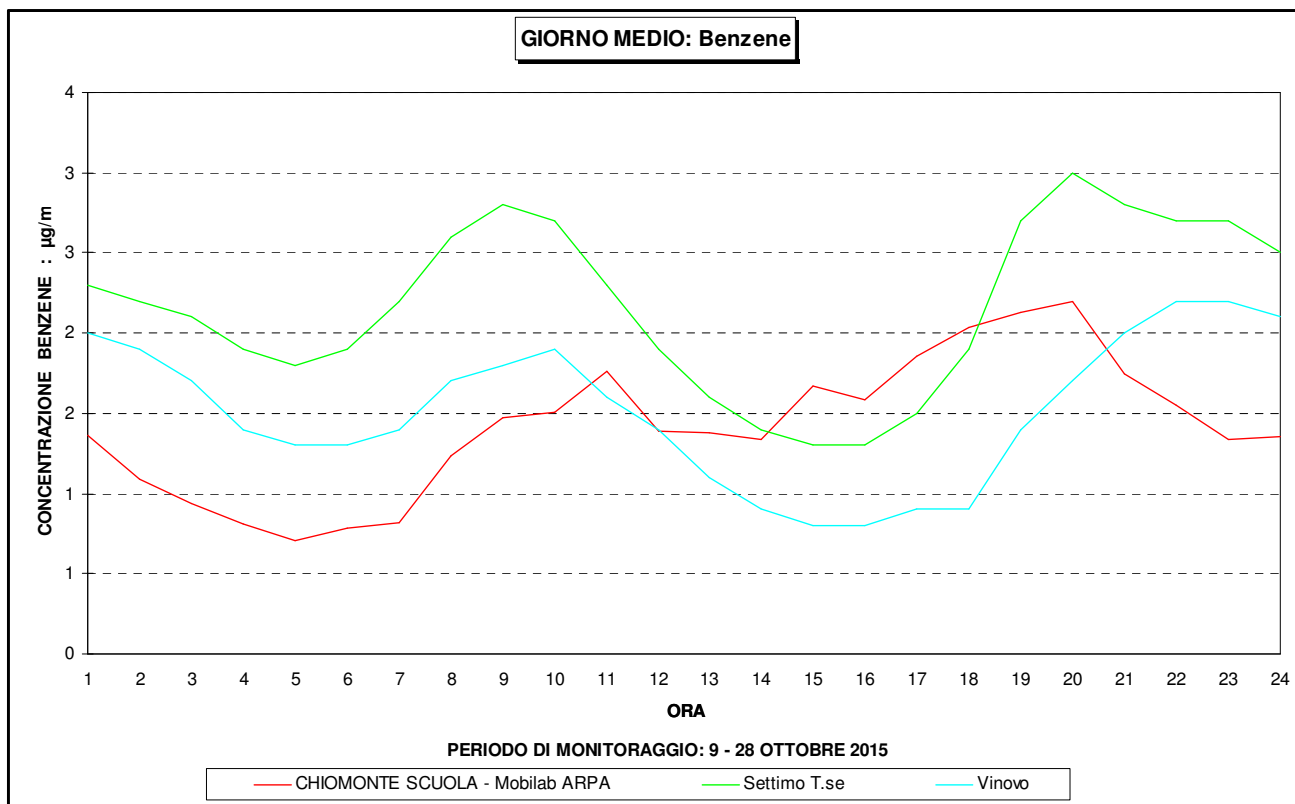
Figura 23 – Benzene: andamento del giorno medio
