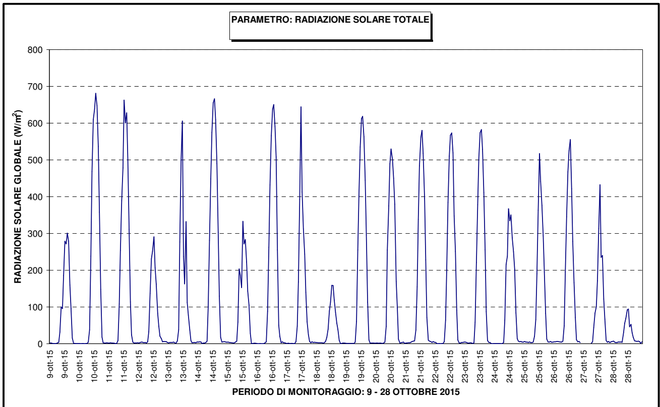
Figura 5 - Andamento della radiazione solare globale (dati della stazione Molaretto – TELT)
